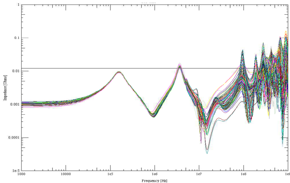
figure 148 : Courbes issues de la simulation « multi-node »
