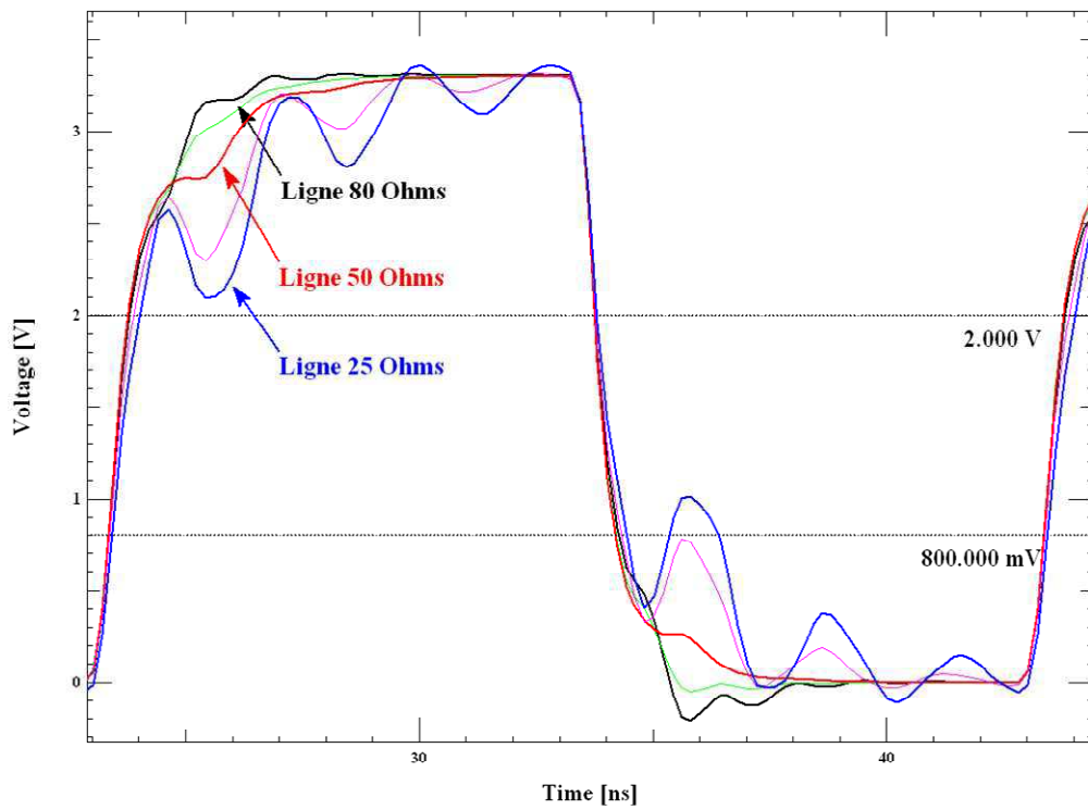
figure 80 : Simulation d'une ligne avec variation d'impédance ( R_{\text{série}} = 50 \Omega )
