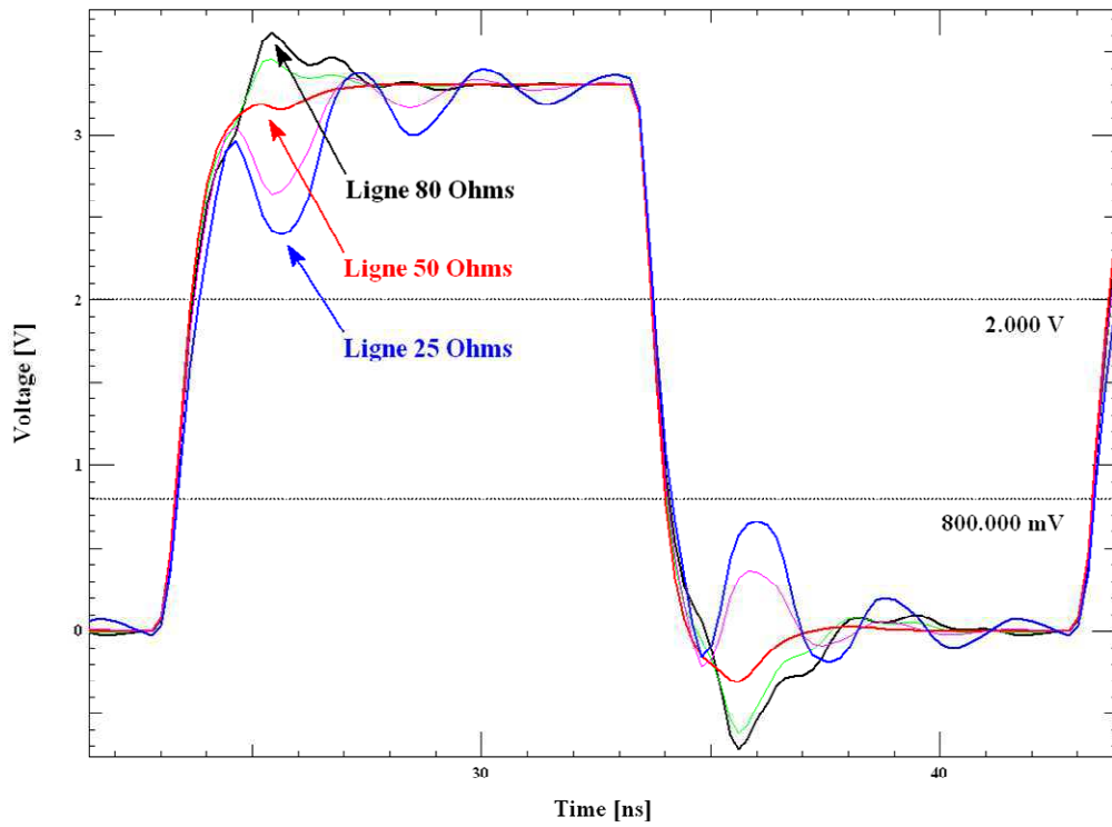
figure 79 : Simulation d'une ligne avec variation d'impédance ( R_{\text{série}} = 35 \Omega )
