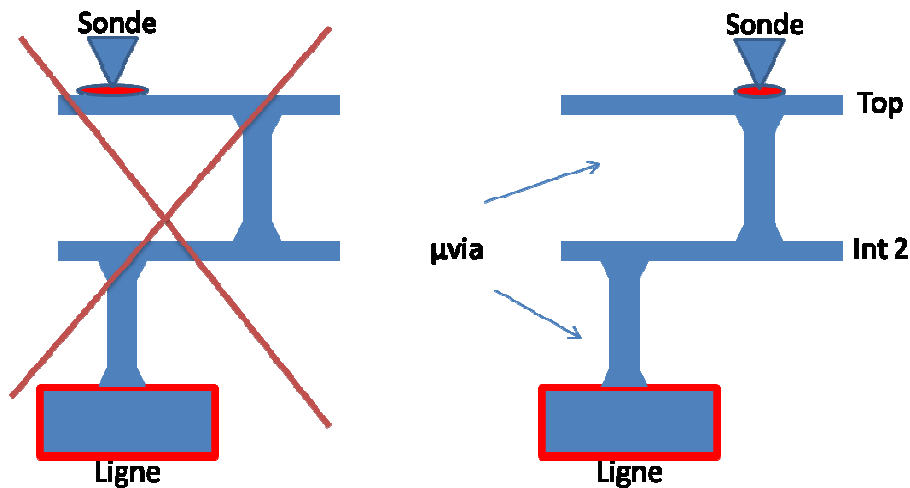
figure 120 : Limitation des perturbations à travers l'optimisation de l'accès à la mesure
