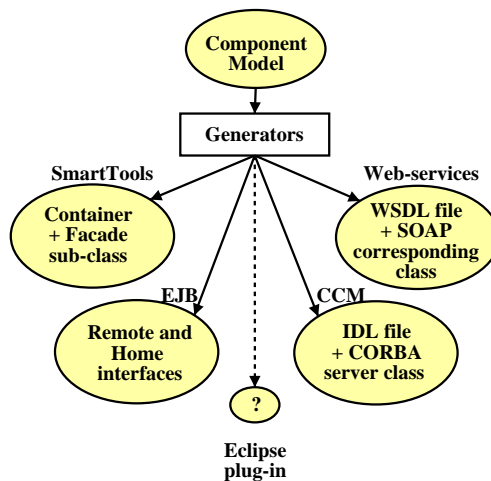
FIG. 1.14: Les transformations de modèles de composants
