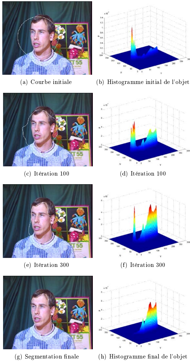
FIG. 6.1 – Evolution de la segmentation et des histogrammes en minimisant l'entropie jointe
