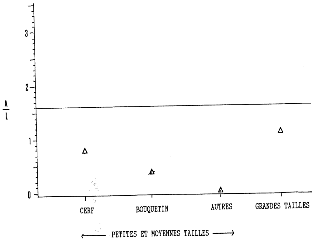
Figure 73 : Rapports d'unités squelettiques ( F/H et A/L ) chez les Artiodactyles du Lazaret (d'après Potts, 1983). Voir explication dans le texte
