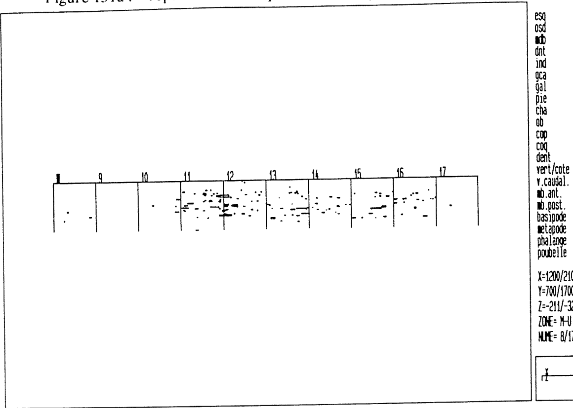
Figure 131a : répartition des coprolithes en coupe longitudinale
