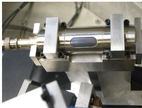
Fig. 2.16 – Photographie du détecteur sur son support.
