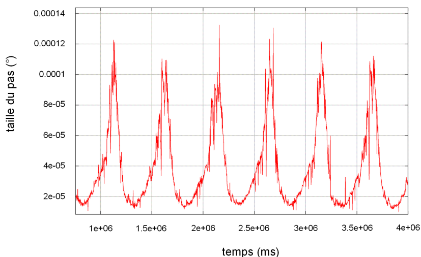
Fig. 2.18 – La taille des pas des moteurs n'est pas constante. Pour ce moteur et des pas de résolution minimale ( 5 \cdot 10^{-5} degrés, l'amplitude d'un pas peut varier d'un facteur 10.
