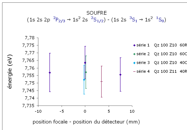
Fig. 1.41 – Résultats pour l'écart en énergie entre la transition 1s\ 2s\ 2p\ ^2P_{3/2} \rightarrow 1s^2\ 2s^2\ ^2S_{1/2} du soufre 13^+ et la transition M1 1s\ 2s\ ^3S_1 \rightarrow 1s^2\ ^1S_0 du soufre 14^+ . Voir la figure 1.40 pour les conventions appliquées à la légende.
