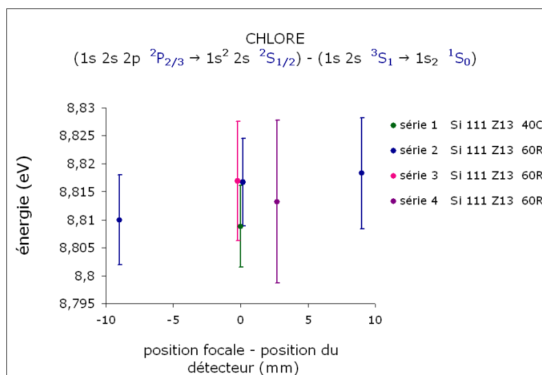
Fig. 1.42 – Résultats pour l'écart en énergie entre la transition 1s\ 2s\ 2p\ ^2P_{3/2} \rightarrow 1s^2\ 2s^2\ ^2S_{1/2} du chlore 14^+ et la transition M1 1s\ 2s\ ^3S_1 \rightarrow 1s^2\ ^1S_0 du chlore 15^+ . Voir la figure 1.40 pour les conventions appliquées à la légende.
