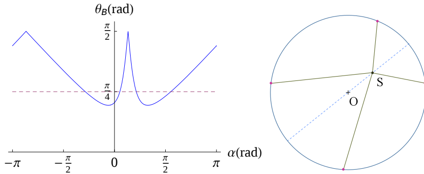
Fig. 1.10 – Exemple de solution des lieux de réflexion, dans le cadre du problème à 2 dimensions.
