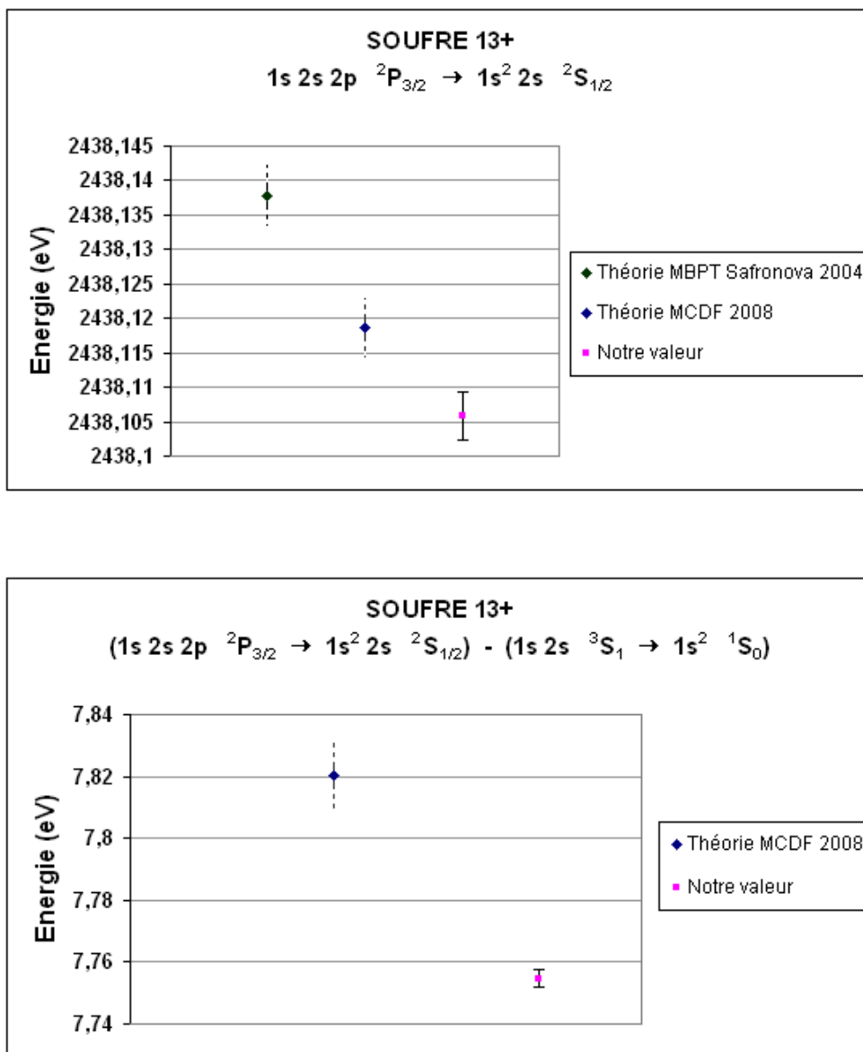
Fig. 1.51 – Comparaison graphique du résultat pour la transition 1s \ 2s \ 2p \ ^2P_{3/2} \rightarrow 1s^2 \ 2s \ ^2S_{1/2} du soufre 13^+ avec les valeurs théoriques [SAFRONOVA and SAFRONOVA 2004 ; INDELICATO 2008]. Sur la figure inférieure, on compare les écarts entre la transition 1s \ 2s \ 2p \ ^2P_{3/2} \rightarrow 1s^2 \ 2s \ ^2S_{1/2} et la transition 1s \ 2s \ ^3S_1 \rightarrow 1s^2 \ ^1S_0 de référence. Les barres d'erreurs en pointillés indiquent que la valeur de l'incertitude n'est pas donnée.
