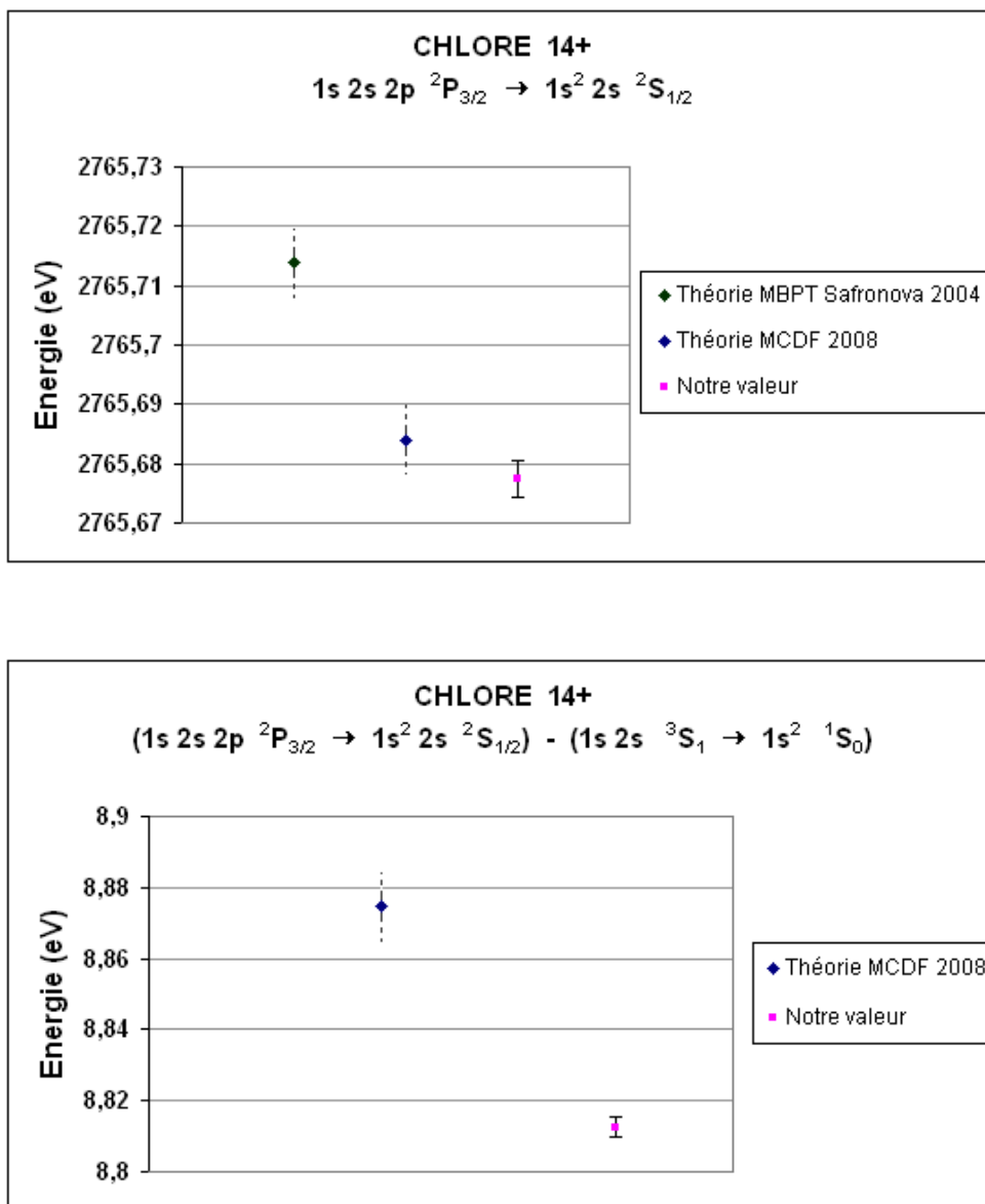
Fig. 1.55 – Comparaison graphique du résultat pour la transition 1s\ 2s\ 2p\ ^2P_{3/2} \rightarrow 1s^2\ 2s^2 S_{1/2} du chlore 14^+ avec les valeurs théoriques [SAFRONOVA and SAFRONOVA 2004 ; INDELICATO 2008]. Sur la figure inférieure, on compare les écarts entre la transition (1s\ 2s\ 2p\ ^2P_{3/2} \rightarrow 1s^2\ 2s^2 S_{1/2}) et la transition 1s\ 2s\ ^3S_1 \rightarrow 1s^2\ ^1S_0 de référence. Les barres d'erreurs en pointillés indiquent que la valeur de l'incertitude n'est pas donnée.
