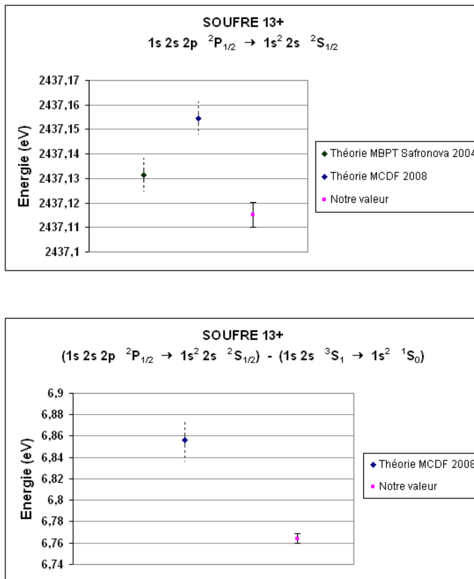
Fig. 1.52 – Comparaison graphique du résultat pour la transition 1s\ 2s\ 2p\ ^2P_{1/2} \rightarrow 1s^2\ 2s\ ^2S_{1/2} du soufre 13^+ avec les valeurs théoriques [SAFRONOVA and SAFRONOVA 2004 ; INDELICATO 2008]. Sur la figure inférieure, on compare les écarts entre la transition (1s\ 2s\ 2p\ ^2P_{1/2} \rightarrow 1s^2\ 2s\ ^2S_{1/2}) et la transition 1s\ 2s\ ^3S_1 \rightarrow 1s^2\ ^1S_0 de référence. Les barres d'erreurs en pointillés indiquent que la valeur de l'incertitude n'est pas donnée.
