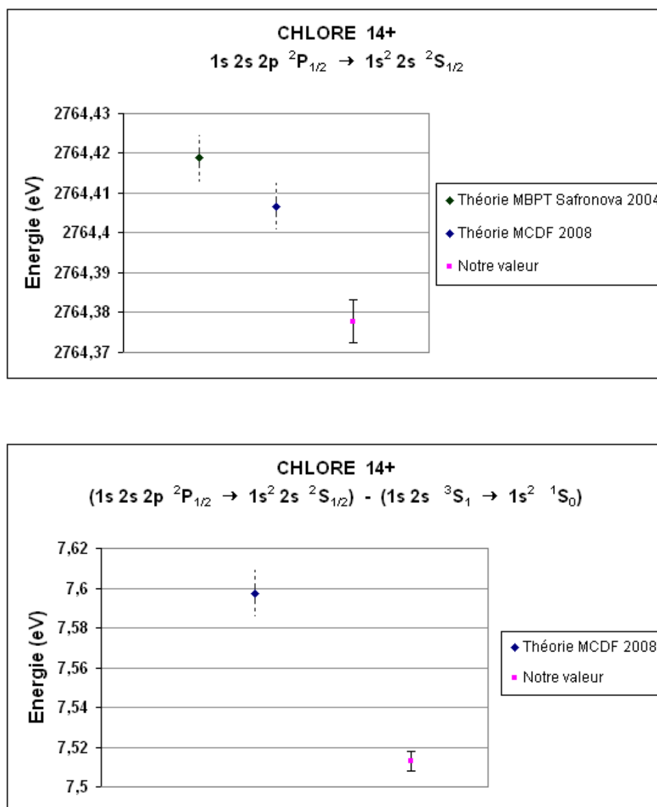
Fig. 1.56 – Comparaison graphique du résultat pour la transition 1s\ 2s\ 2p\ ^2P_{1/2} \rightarrow 1s^2\ 2s^2 S_{1/2} du chlore 14^+ avec la valeur théorique [SAFRONOVA and SAFRONOVA 2004 ; INDELICATO 2008]. Sur la figure inférieure, on compare les écarts entre la transition 1s\ 2s\ 2p\ ^2P_{1/2} \rightarrow 1s^2\ 2s^2 S_{1/2} et la transition 1s\ 2s\ ^3S_1 \rightarrow 1s^2\ ^1S_0 de référence. Les barres d'erreurs en pointillés indiquent que la valeur de l'incertitude n'est pas donnée.
