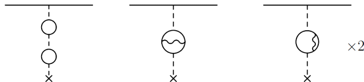
Fig. 3.6 – Diagrammes de polarisation du vide à deux boucles.
