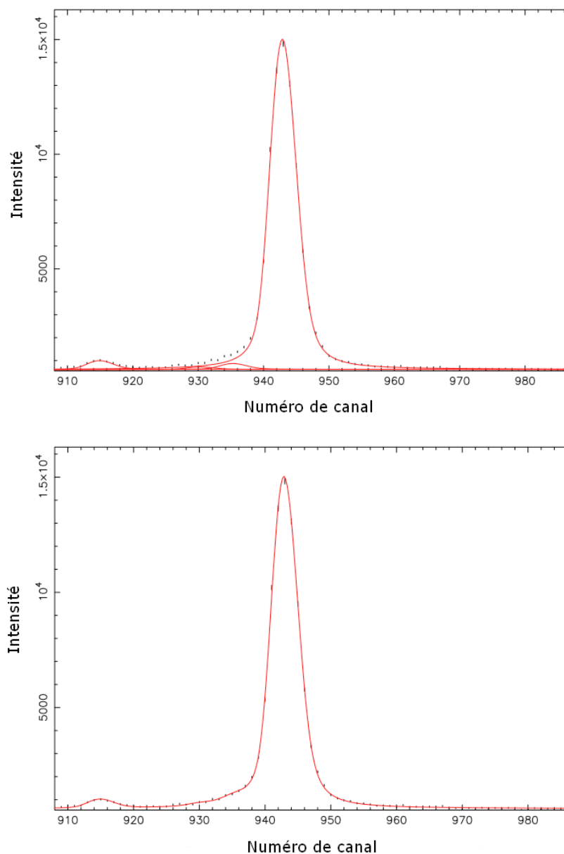
Fig. 1.34 – Exemple de résultat fourni par le programme après l'ajustement des profils simulés pour la raie de la transition M1 de l'argon héliumoïde ( 16^+ ) 1s\ 2s\ ^3S_1 \rightarrow 1s^2\ ^1S_0 . Sur la figure du bas la courbe rouge est la somme des différentes courbes de la figure du haut.
