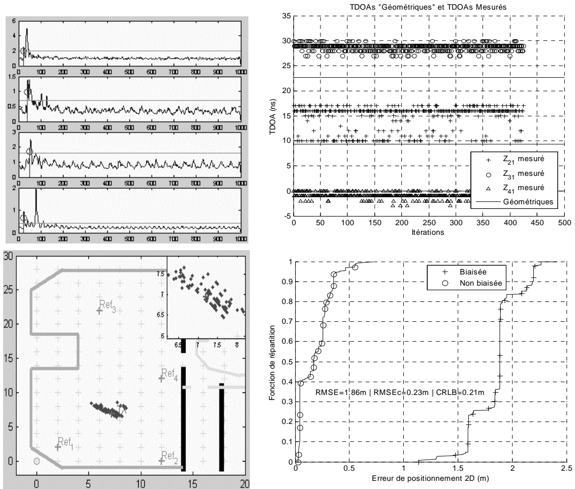
Figure 6 - 9 : Exemple de formes d'onde obtenues après 20 accumulations pour le récepteur « à détection d'énergie » , TDOA théoriques et mesurés , positions estimées (LS-TSE) d'un émetteur TX en (6,8)m avec 4 antennes de référence Ref; en visibilité encadrant la scène, et fonction de la répartition de l'erreur de positionnement
