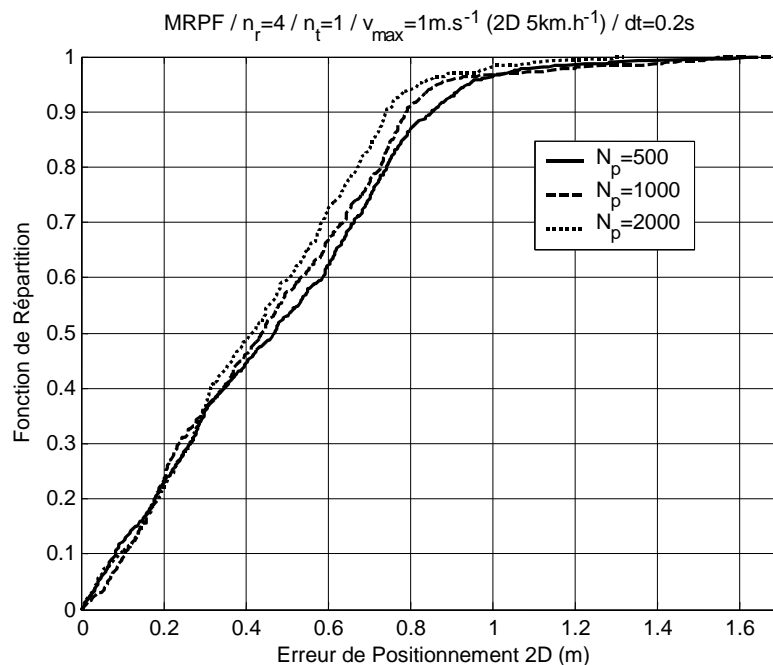
Figure 5 - 8 : Fonction de répartition de l' erreur 2D de positionnement le long de la trajectoire canonique de test (Figure 5 - 1) pour le filtre MRPF , une vitesse maximale 1D de 1\text{m.s}^{-1} , n_r=4 références, une détection systématique du plus fort trajet ( n_t=1 trajet estimé), et une période de rafraîchissement dt=0.2\text{s} , en fonction du nombre N_p de particules
