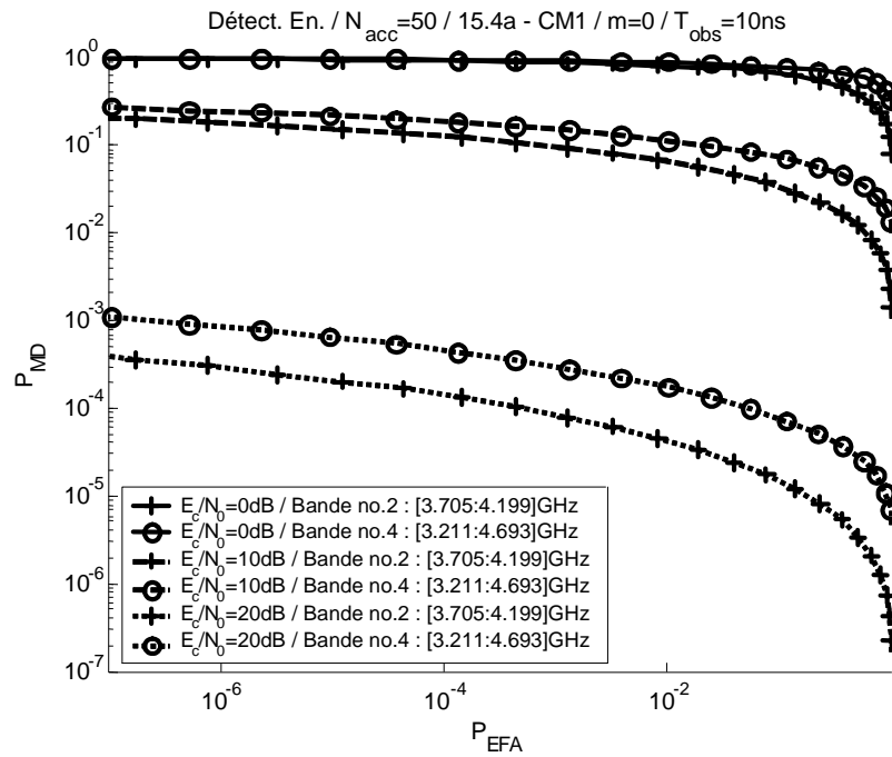
Figure 3 - 10 : Performances de détection de l'architecture à base de détection d'énergie pour le canal 15.4a – CMI après accumulation de l'énergie de N_{acc}=50 impulsions successives, en fonction de la bande et de l' énergie étalée sur l'intégralité du canal (d'après (Eq. 3 – 23) avec m=0 , et (Eq. 3 – 26) avec T_{obs}=10ns )
