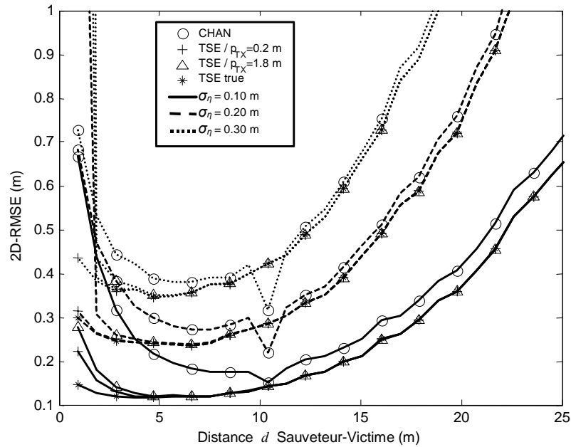
Figure 4 - 23 : Racine de l'erreur quadratique moyenne 2D-RMSE en fonction de la distance sauveteur-victime avec une référence principale en (0,0,1.5)m, des référence périphériques en (0,15,0.05)m, et (15,0,0.05)m, un émetteur enfoui en différentes positions depuis l'origine jusqu'à (20,20,-1)m, avec n_s=1.7 , \sigma_\eta entre 0.10m et 0.30m
