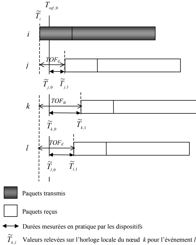
Figure 1 - 10 : Protocole générique “aller-simple” (OWR) dans le mode actif pour la mesure de différences de temps d’arrivée (TDOA) défini à l’aide de trois nœuds isochrones
