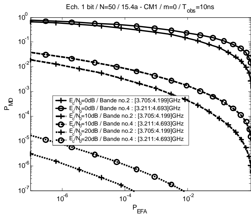
Figure 3 - 11 : Performances de détection de l'architecture à base d' échantillonnage et quantification sur 1 bit pour le canal 15.4a – CMI avec intégration cohérente de N=50 impulsions successives, en fonction de la bande et de l' énergie étalée sur l'intégralité du canal (d'après (Eq. 3 – 23) avec m=0 , et (Eq. 3 – 26) avec T_{obs}=10ns )
