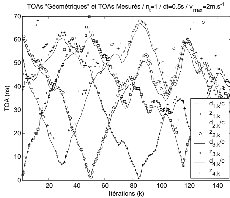
Figure 5 - 2 : Exemples de temps d'arrivée mesurés pour la trajectoire représentée sur la Figure 5 - 1, avec une détection systématique du plus fort trajet ( n_t=1 )
