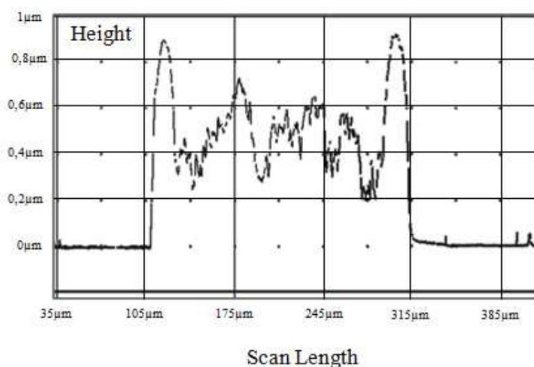
Figure.22 : Profil en épaisseur d'une couche de ZnO de 30 gouttes
