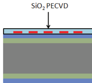
Figure.4 : Dépôt de la couche d'isolation \text{SiO}_2 PECVD
