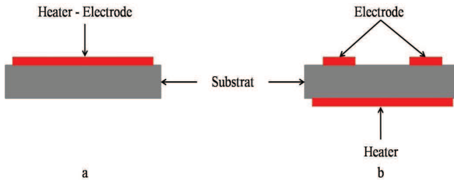
Figure.5 : Plateforme sur substrat a) métallisations sur la même face b) métallisations double faces
