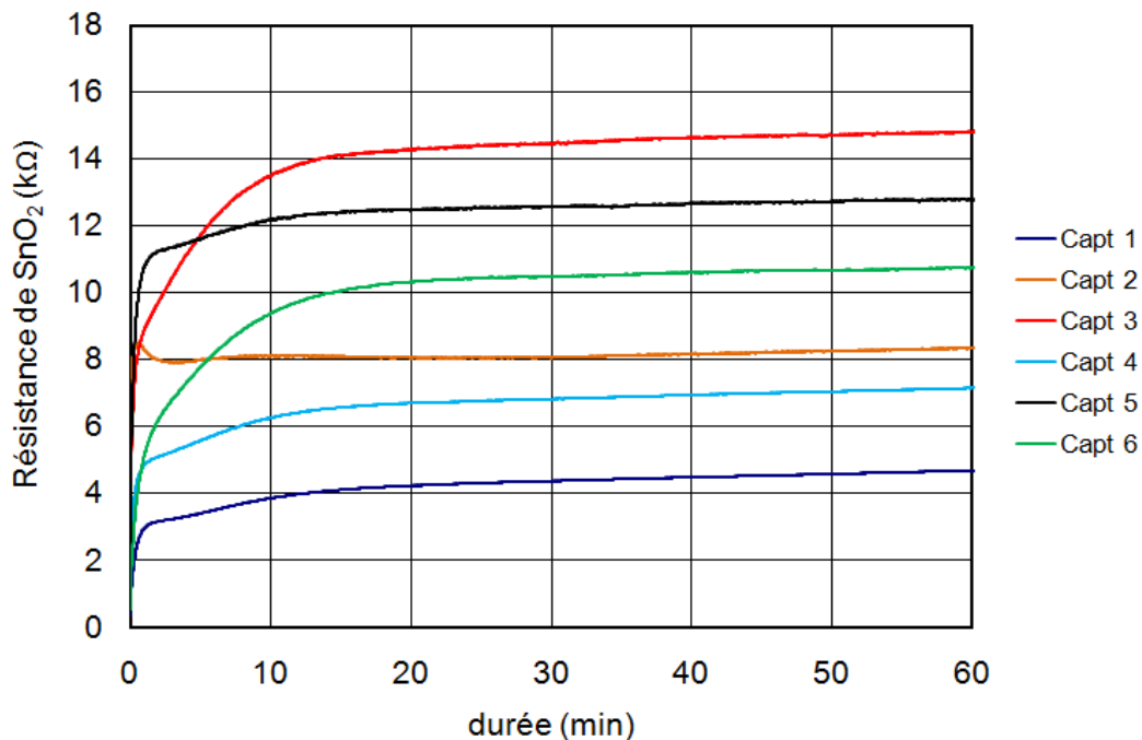
Figure.2 : Réponses sous air de 6 capteurs de R_H de l'ordre de 440\Omega sur le banc du LCC : disparité des résistances
