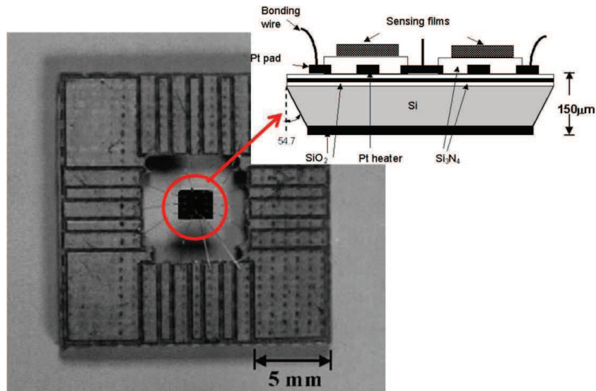
Figure.14 : Plateforme sur substrat suspendue [52]
