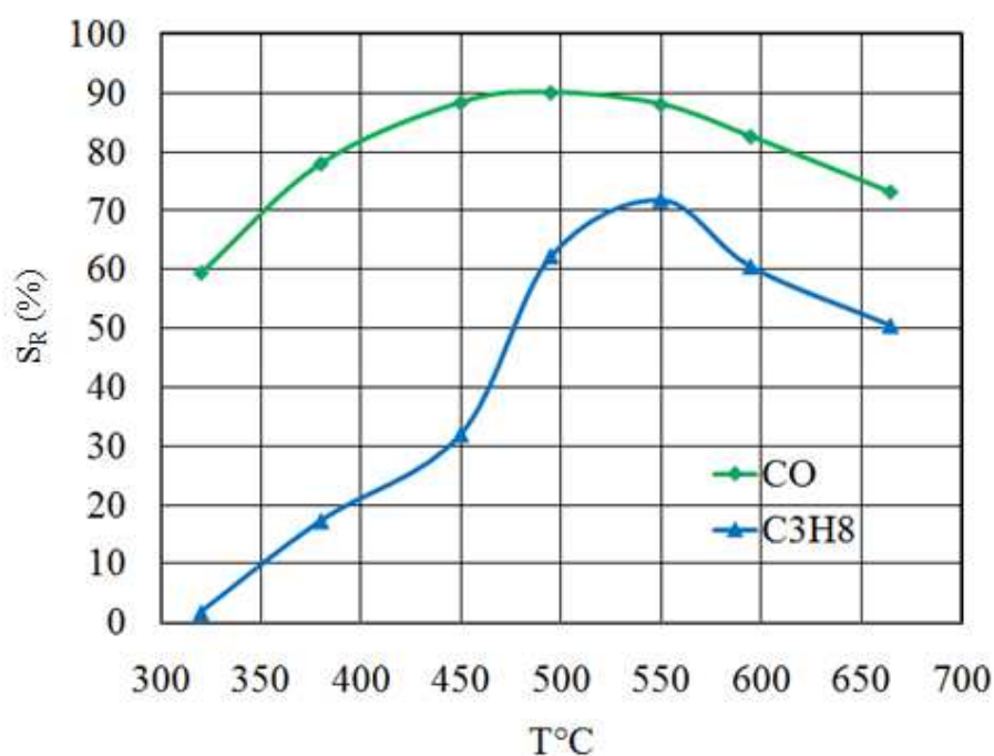
Figure.6 : Variation de réponse relative S_R au CO et au C 3 H 8 en fonction de la température de fonctionnement
