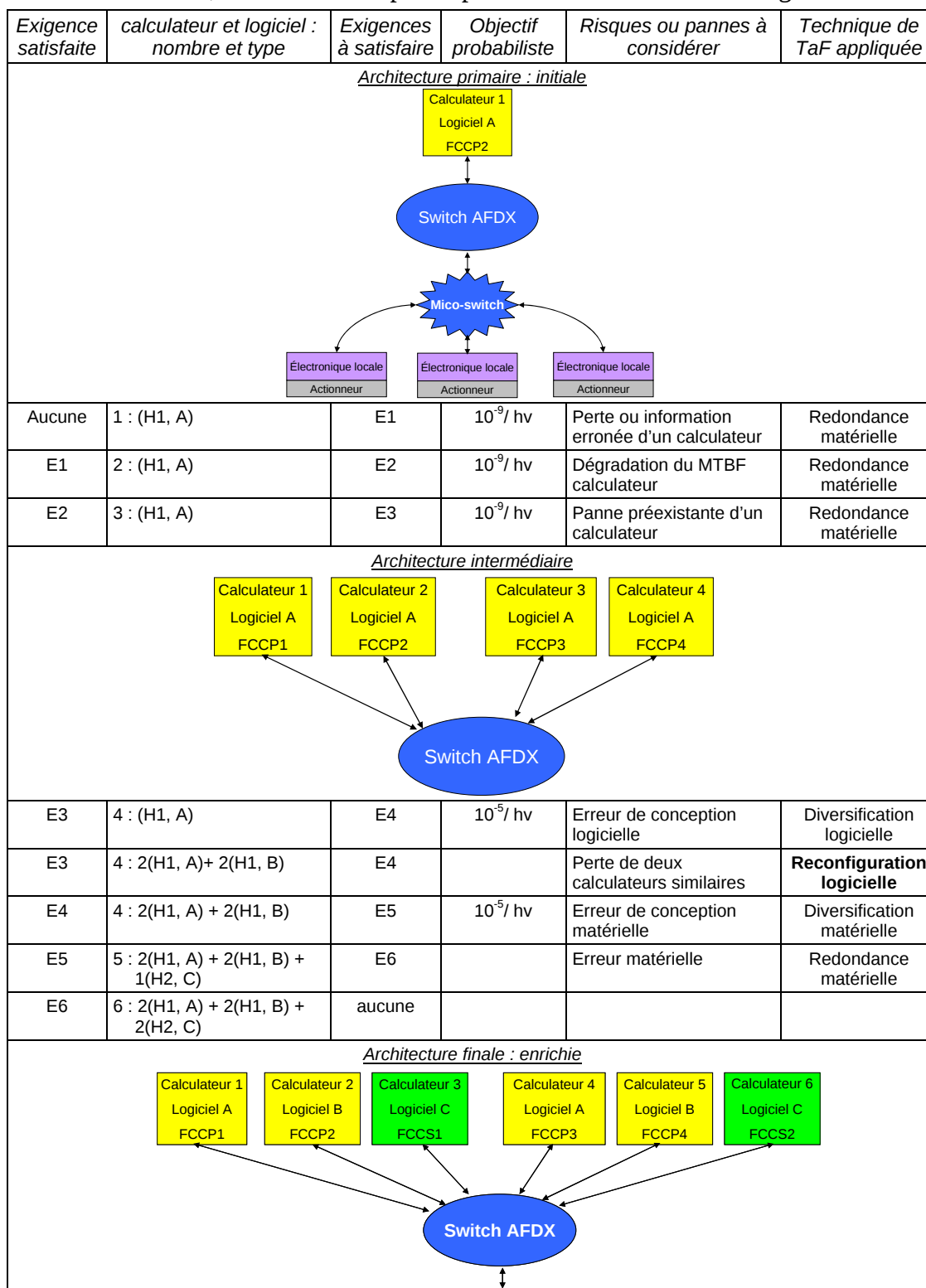
Figure II.5. – Exemple d'injection des exigences non fonctionnelles sur le sous-système calculateur
