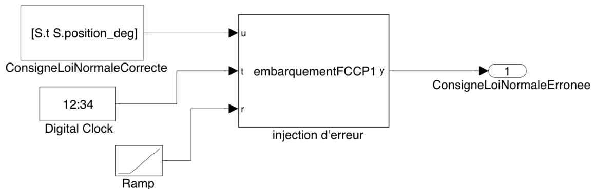
Figure IV.26 - Modèle d'injection d'erreur pour la panne solide
