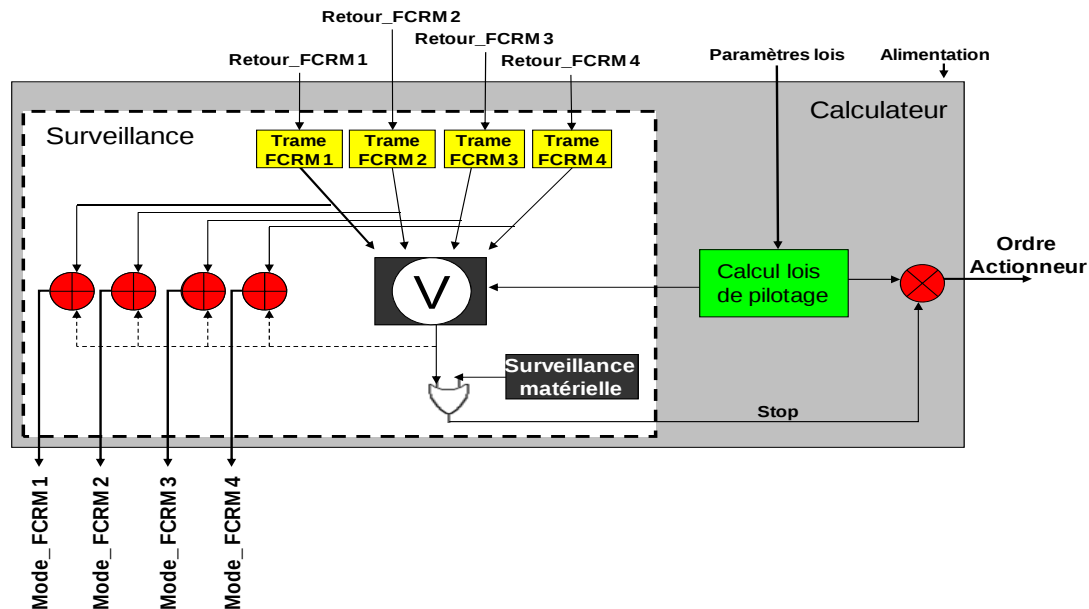
Figure III.3 - Schéma fonctionnel détaillé d'un calculateur simplex
