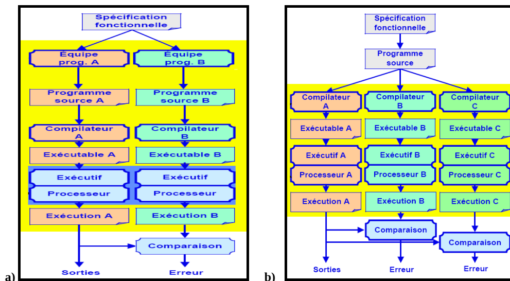
Figure I.2. - Principe de développement d'un composant logiciel diversifié :
