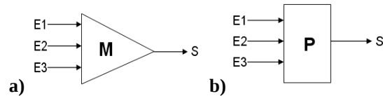
Figure III.8 - Schéma fonctionnel d'un : a) voteur de la médiane ; b) passivateur
