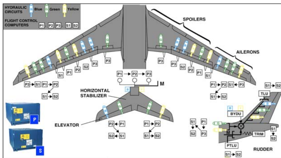
Figure I.4. - Distribution des ordinateurs PRIM et SEC sur les gouvernes
