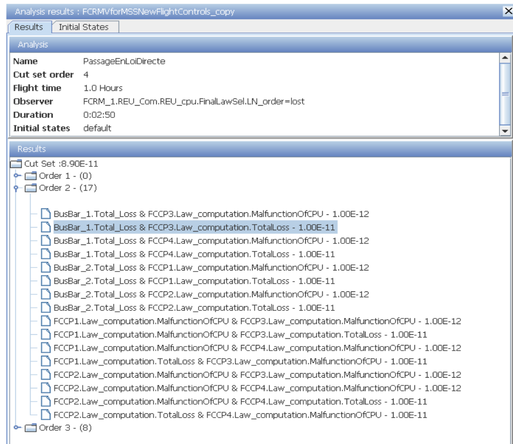
Figure IV.18 - FC2 : Passage en loi directe
