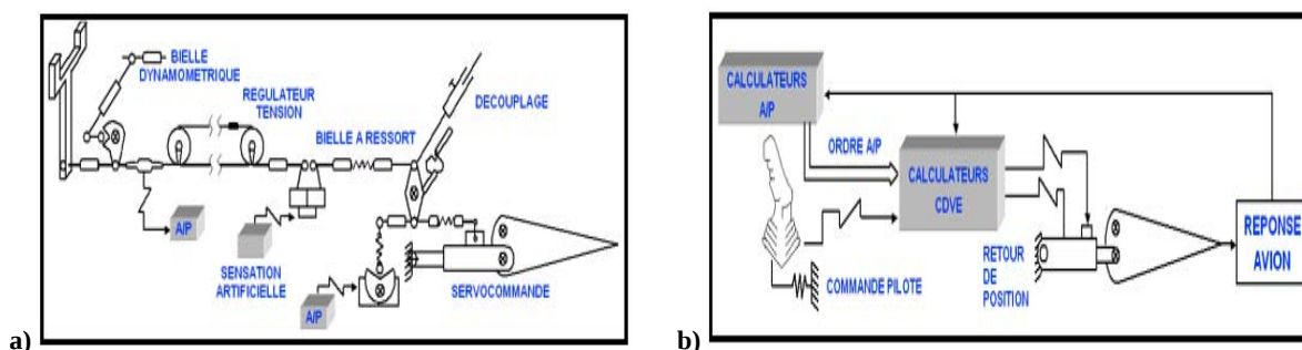
Figure I.1 - a) Commandes de vol mécanique avec servocommande des actionneurs b) Commandes de vol totalement électriques
