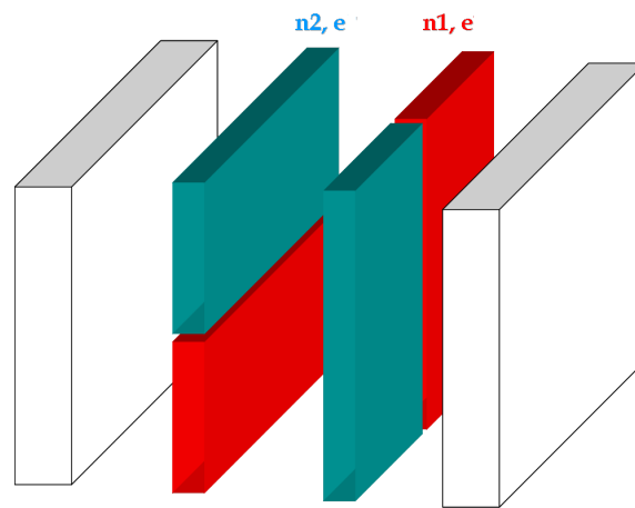
FIG. 2.2 – Assemblage optique du masque coronographique de l'APKC : deux couteaux de phase de 99 \mu\text{m} d'épaisseur sont accolés entre deux épais lames de verre de 6 mm.
