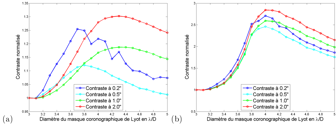
FIG. 5.10 – Optimisation de la taille du masque coronagraphique en tenant compte des aberrations : évolution des contrastes de l’ALC à 0.2", 0.5", 1" et 2" en fonction du diamètre angulaire du masque coronagraphique pour (a) le cas brut, (b) en tenant compte de l’allure de la PSF.
