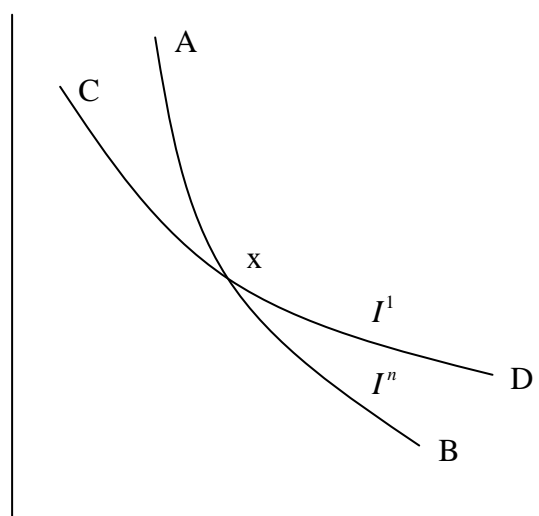
Figure 1 : Intersection d'un classement partiel ( ibidem ).
