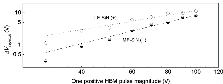
FIGURE 4.14: La dérive de V_{capamin} en fonction d'une impulsion positive HBM pour des valeurs de tension allant de 30 à 100V, pour les structures MF-SiN et LF-SiN.
