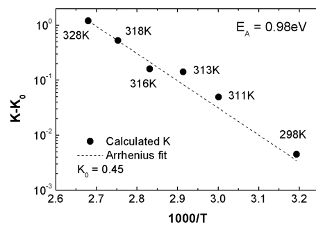
FIGURE 4.22: Le fit utilisant la loi d'Arrhenius.
