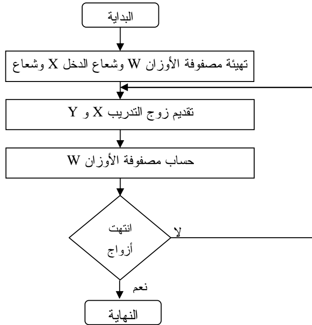
الشكل (5-2)، المخطط الصندوقي لمرحلة التدريب لشبكة BAM.
