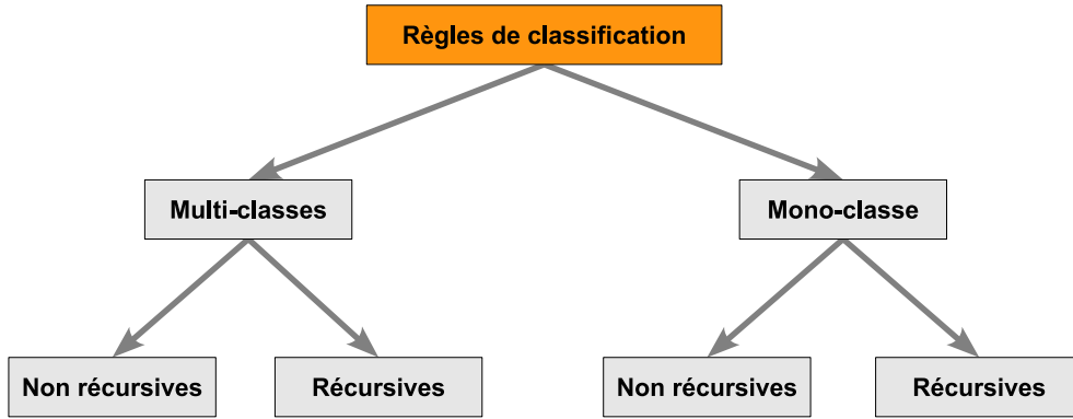
FIGURE 3.12 – Hiérarchie des règles de classification.
