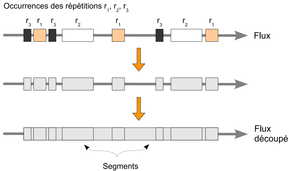
FIGURE 2.9 – Schéma de découpage du flux à partir des occurrences des répétitions.
