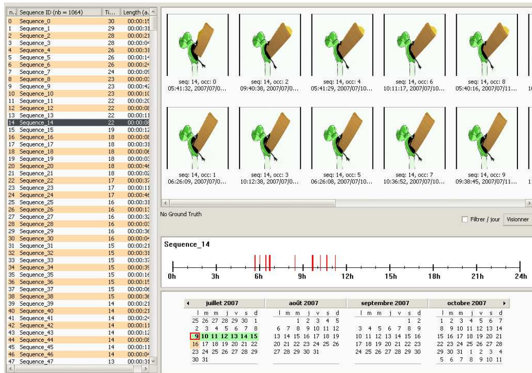
FIGURE 13 – Interface de l'explorateur des répétitions détectées.
