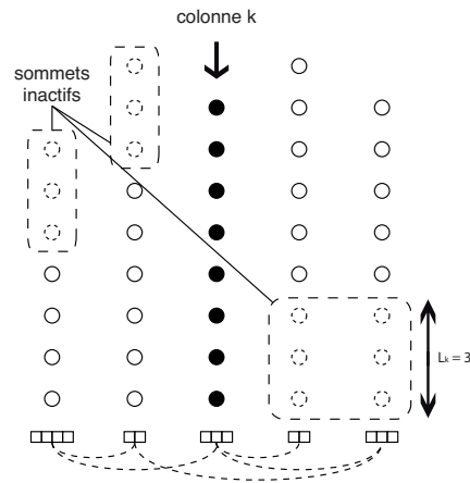
FIG. 5.3 – Illustration du découpage induit par l'activation d'une colonne sur un graphe GAL1 . Les contraintes d'ordre et de non-chevauchement impliquent l'inactivation des sommets en pointillés si la colonne centrale est activée.
