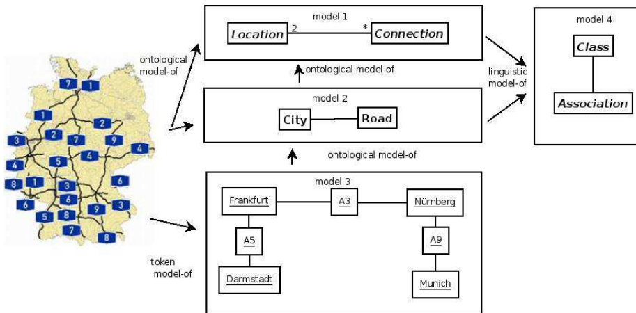
FIG. 2.2 : Illustration des relations est un modèle de
