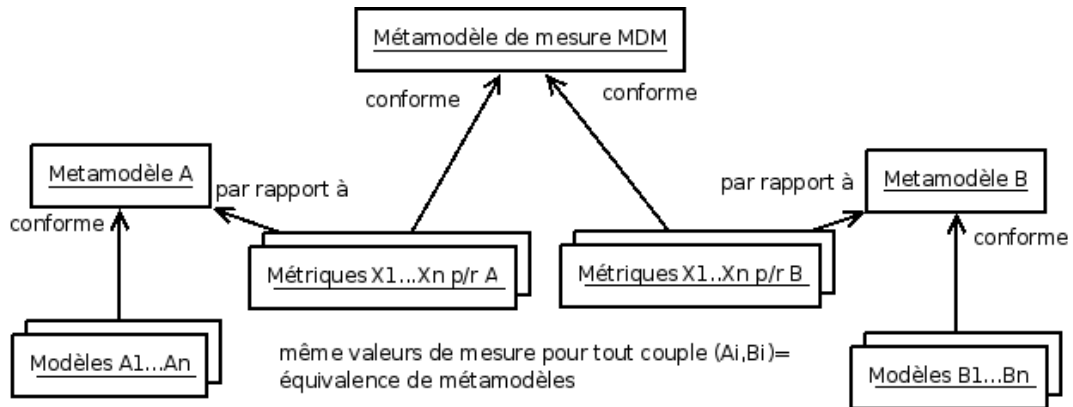
FIG. 5.1 : Classe d'équivalence des métamodèles définie par la mesure
