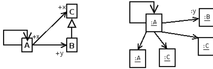
FIG. 3.10 : Un métamodèle fictif et un modèle conforme
