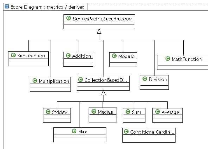
FIG. 3.12 : Opérateurs pour les métriques dérivées
