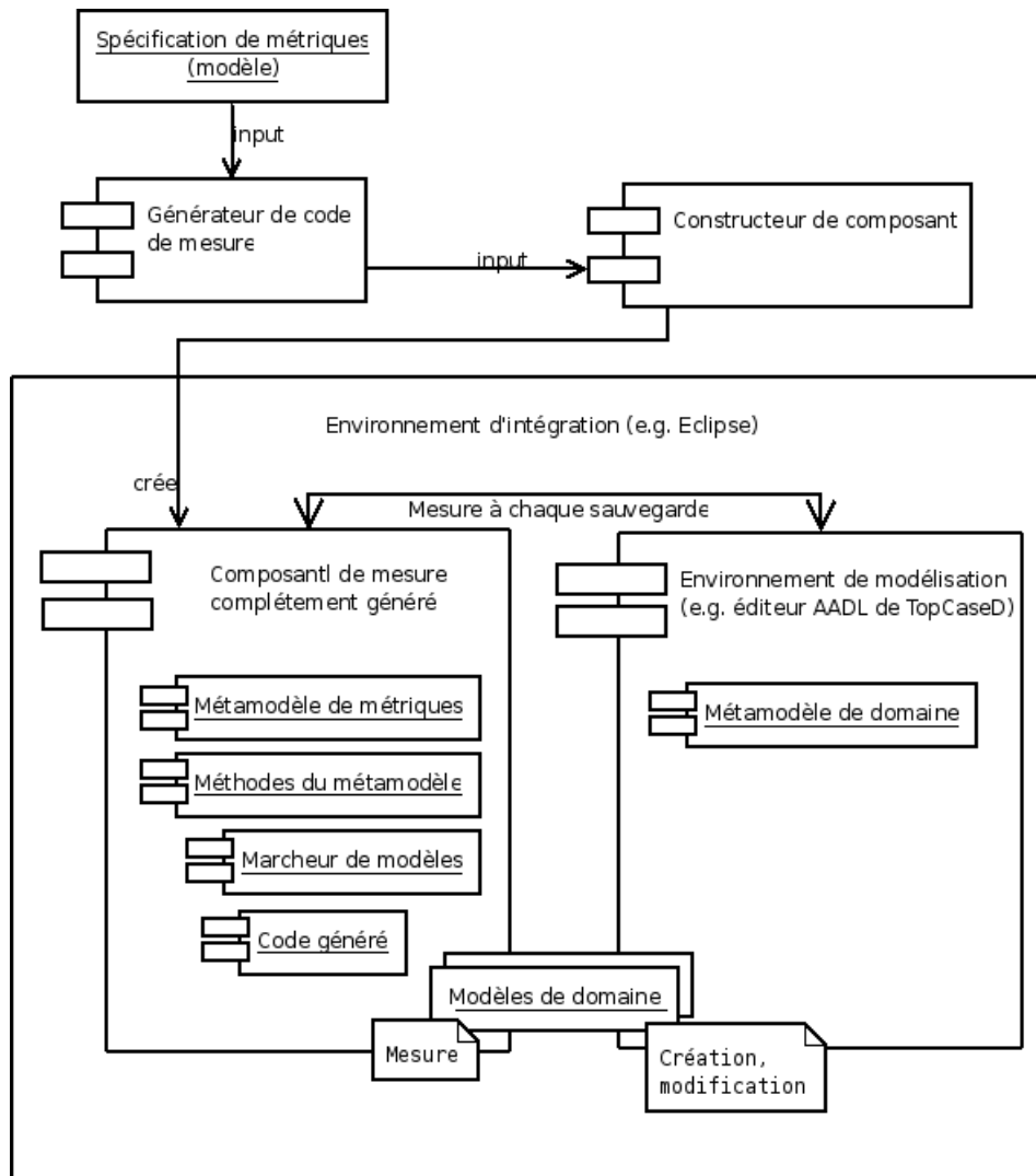
FIG. 3.22 : Vue globale de notre contribution: composants
