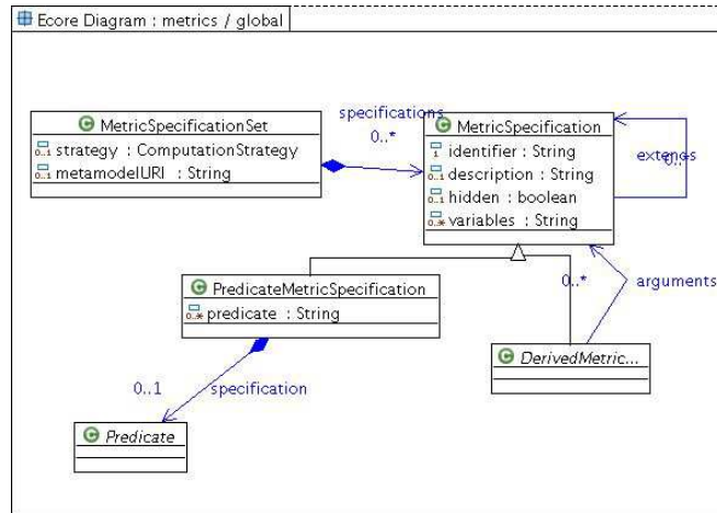
FIG. 3.7 : Le coeur du métamodèle de spécification de métriques
