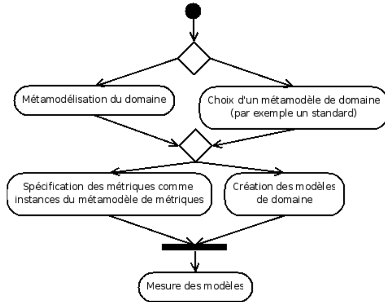
FIG. 3.4 : Un diagramme d'activité de l'approche MDM
