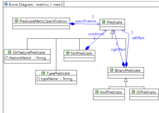
FIG. 3.13 : Les prédicats
