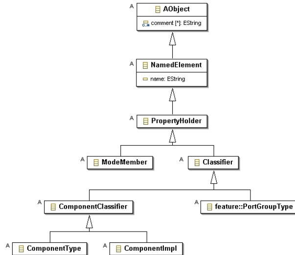
FIG. 4.3 : Extrait du métamodèle AADL
