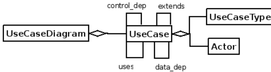
FIG. 2.6 : Métamodèle de cas d'utilisation de [Saeki, 2003]
