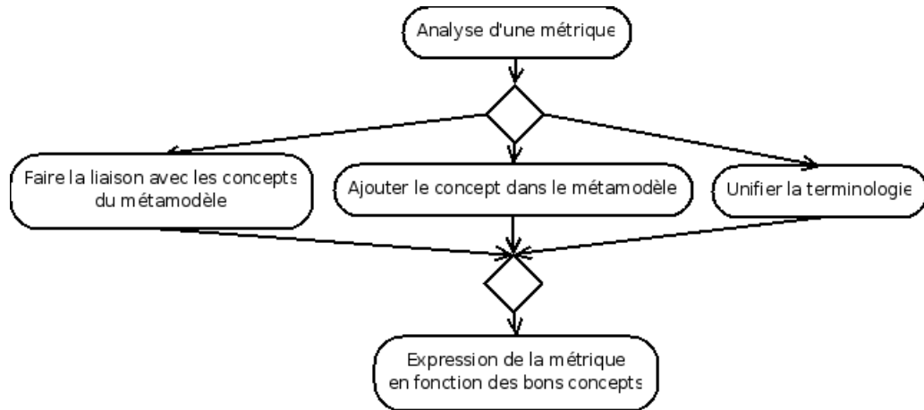
FIG. 4.7 : Le processus de métamodélisation dirigé par les métriques
