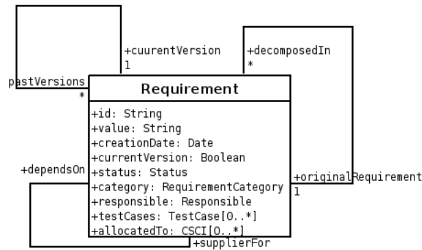
FIG. 4.9 : La classe représentant une exigence
