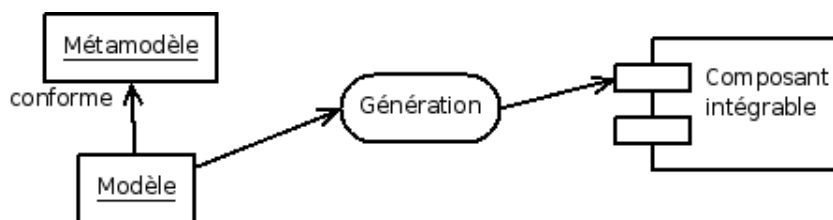
FIG. 3.20 : Principe de génération d'un composant logiciel à partir d'un modèle
