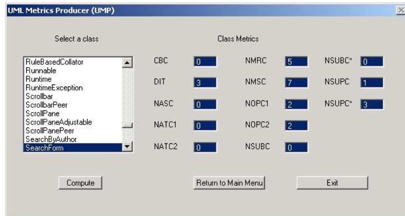
FIG. 2.5 : Une vue de l'interface graphique de UMP [Kim et Boldyreff, 2002]
