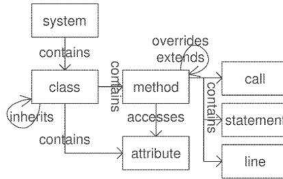
FIG. 2.3 : Métamodèle de logiciel OO de [Lanza et Ducasse, 2002]
