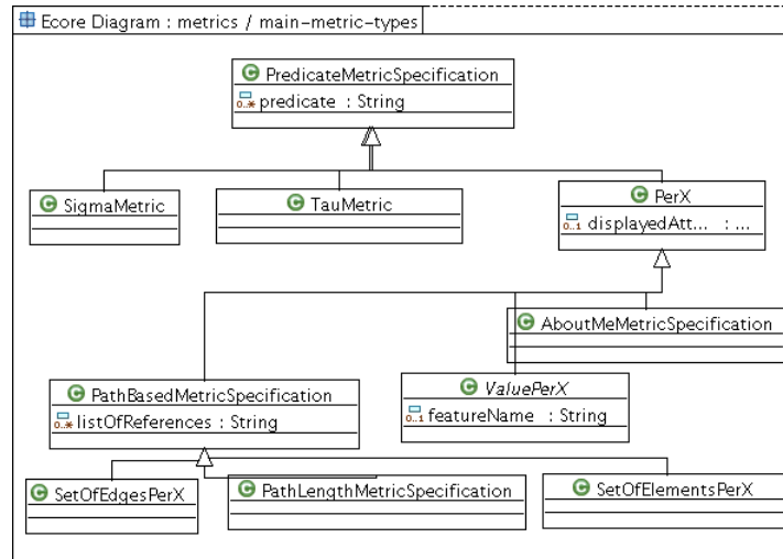
FIG. 3.8 : Les différents types de métriques identifiés
