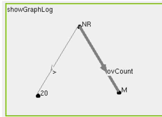
FIG. 2.7 : Exemple de métrique spécifiée en GraphLog
