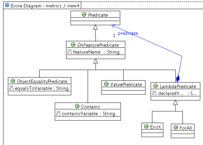
FIG. 3.14 : Test sur les caractéristiques d'un élément de modèle
