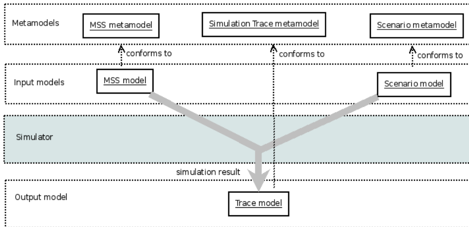
FIG. 4.5 : L'architecture du processus de simulation
