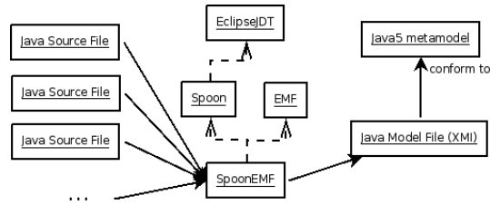
FIG. 4.2 : La transformation Java vers modèle
