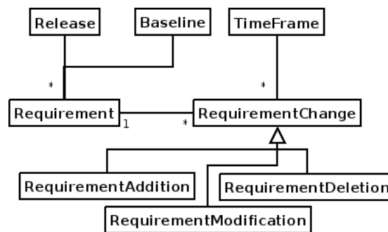
FIG. 4.10 : Gestion du cycle de vie des exigences
