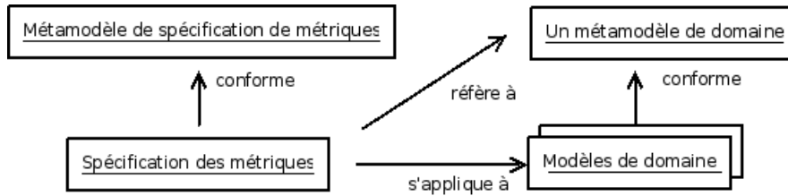
FIG. 3.3 : Artefacts de type modèles impliqués dans notre approche
