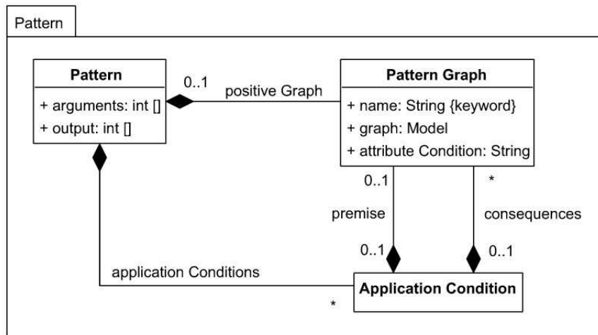
FIG. 2.9 : Le métamodèle de pattern de Slammer
