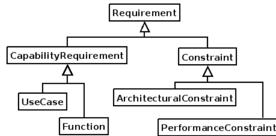
FIG. 4.8 : L'arbre d'héritage des types d'exigences
