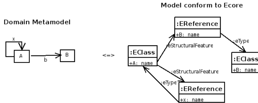
FIG. 4.11 : Un métamodèle de domaine vu en tant que modèle
