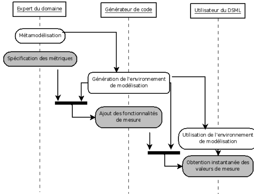
FIG. 3.6 : Vue globale de notre contribution: processus
