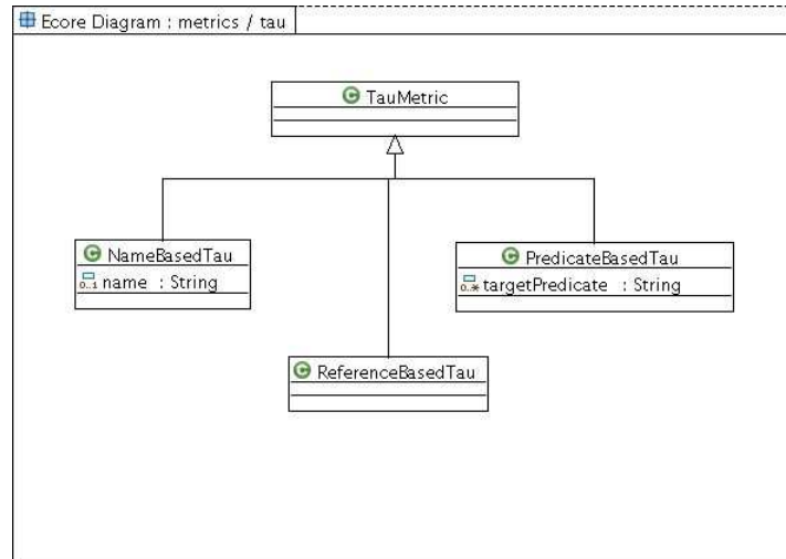
FIG. 3.11 : Les trois raffinements de la métrique Tau
