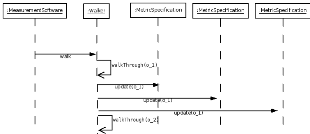
FIG. 3.17 : Interactions entre le marcheur et les spécifications de métriques
