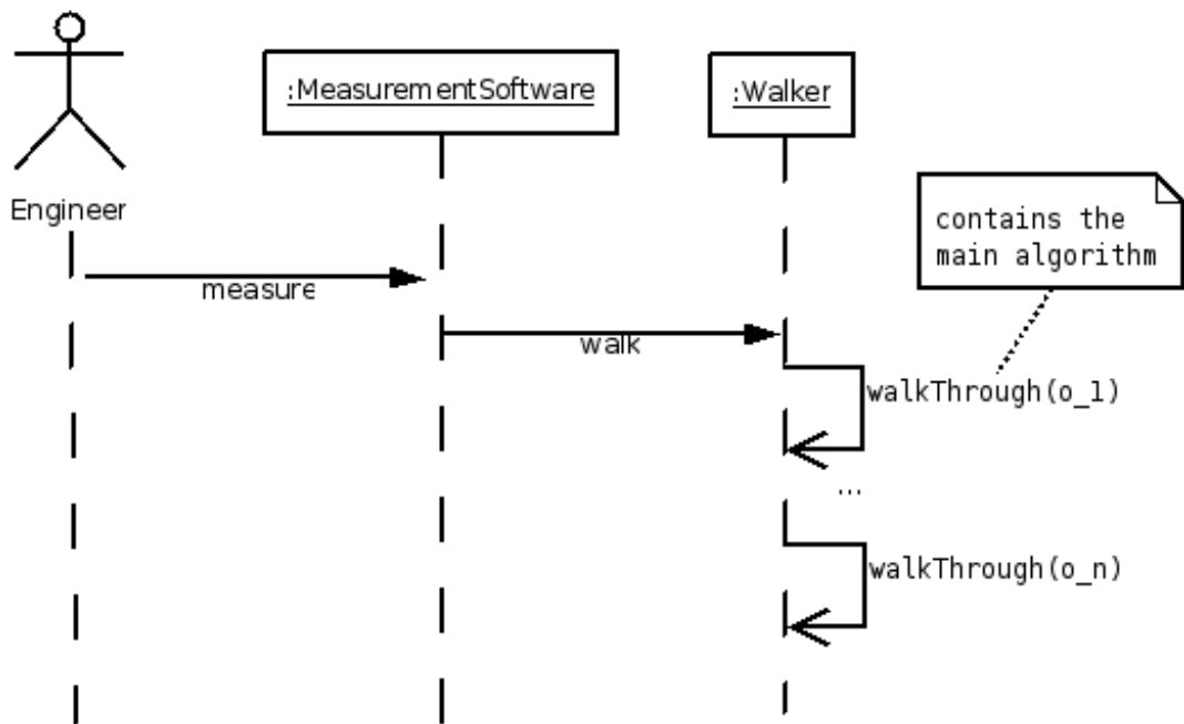
FIG. 3.16 : Principe de la marche
