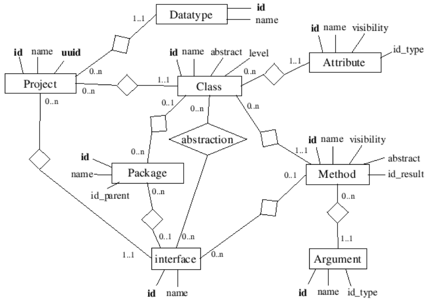
FIG. 2.4 : Un extrait du schéma ER pour UML de [Lavazza et Agostini, 2005]
