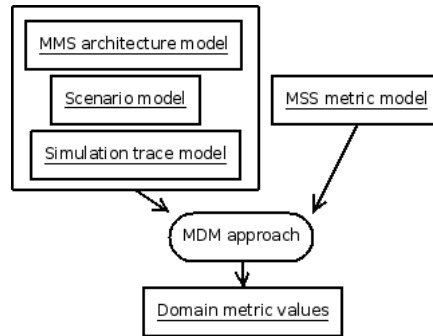
FIG. 4.6 : L'approche MDM appliquée aux modèles de systèmes de surveillance maritime
