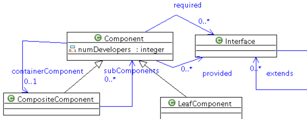
FIG. 3.2 : Le métamodèle de domaine que nous utiliserons pour illustrer notre contribution.
