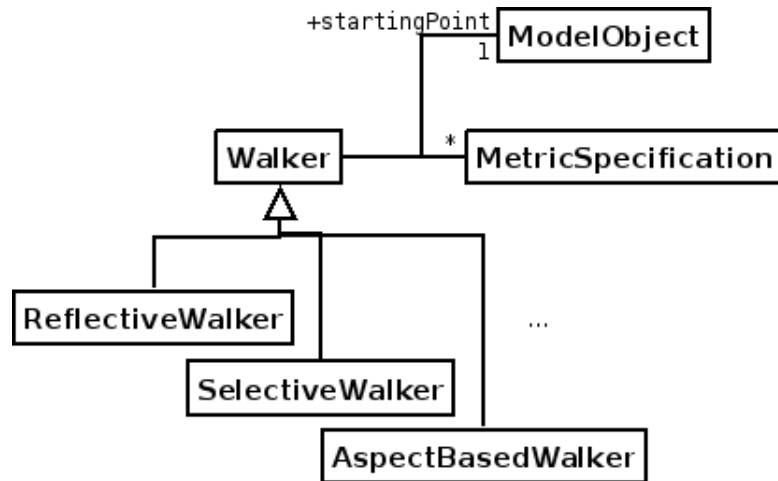
FIG. 3.15 : Marcheur: références et sous-classes
