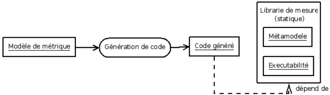
FIG. 3.18 : Principe du métamodèle comme librairie
