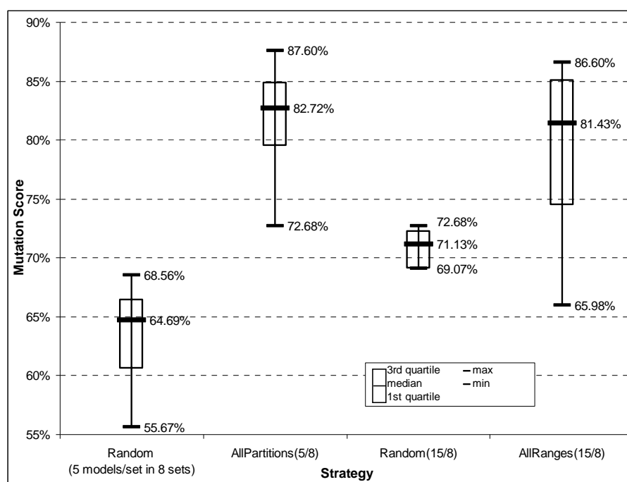
Figure 5-24 - Diagramme "boîte à moustaches" pour la comparaison des stratégies de sélection de modèles
