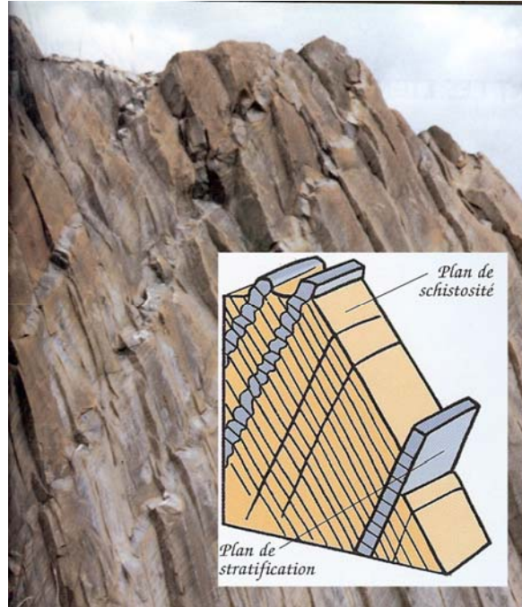
Fig. 12 : L'ardoise, exemple typique de roche schisteuse (Mattauer, 1998 : 115)
