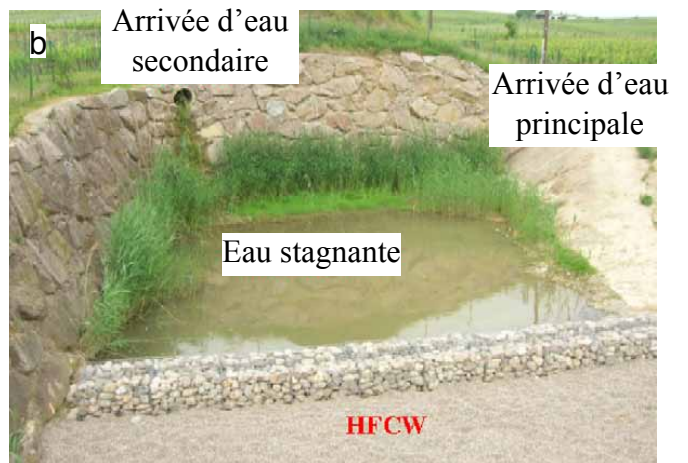
Figure II.3 : Arrivées d'eau du bassin d'orage et points de prélèvement. a : schéma vue de dessus (Source personnelle) ; b : photo vue depuis l'Est (Wanko et coll. 2009).
