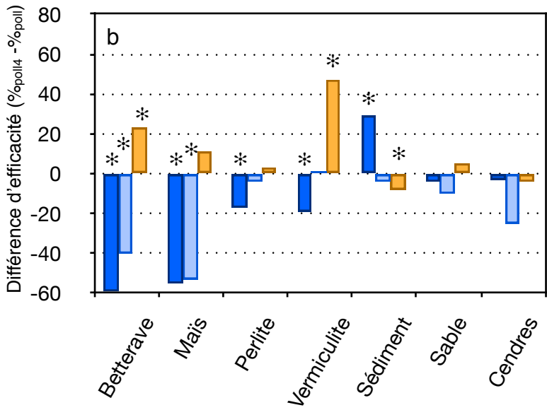
Figure III.3 : Evolution de la sorption du glyphosate, du diuron et du 3,4-DCA en milieu complexe (mélange de polluants). a : glyphosate ; b : diuron ; c : 3,4-DCA. Les valeurs représentées sont les différences de pourcentage de sorption entre la modalité polluant en mélange (poll4) et polluant seul (poll) : \%ads_{poll4} - \%ads_{poll} . Les astérisques signalent les cas où les pourcentages \%ads_{poll4} et \%ads_{poll} sont significativement différents ( P < 0,05 ).
