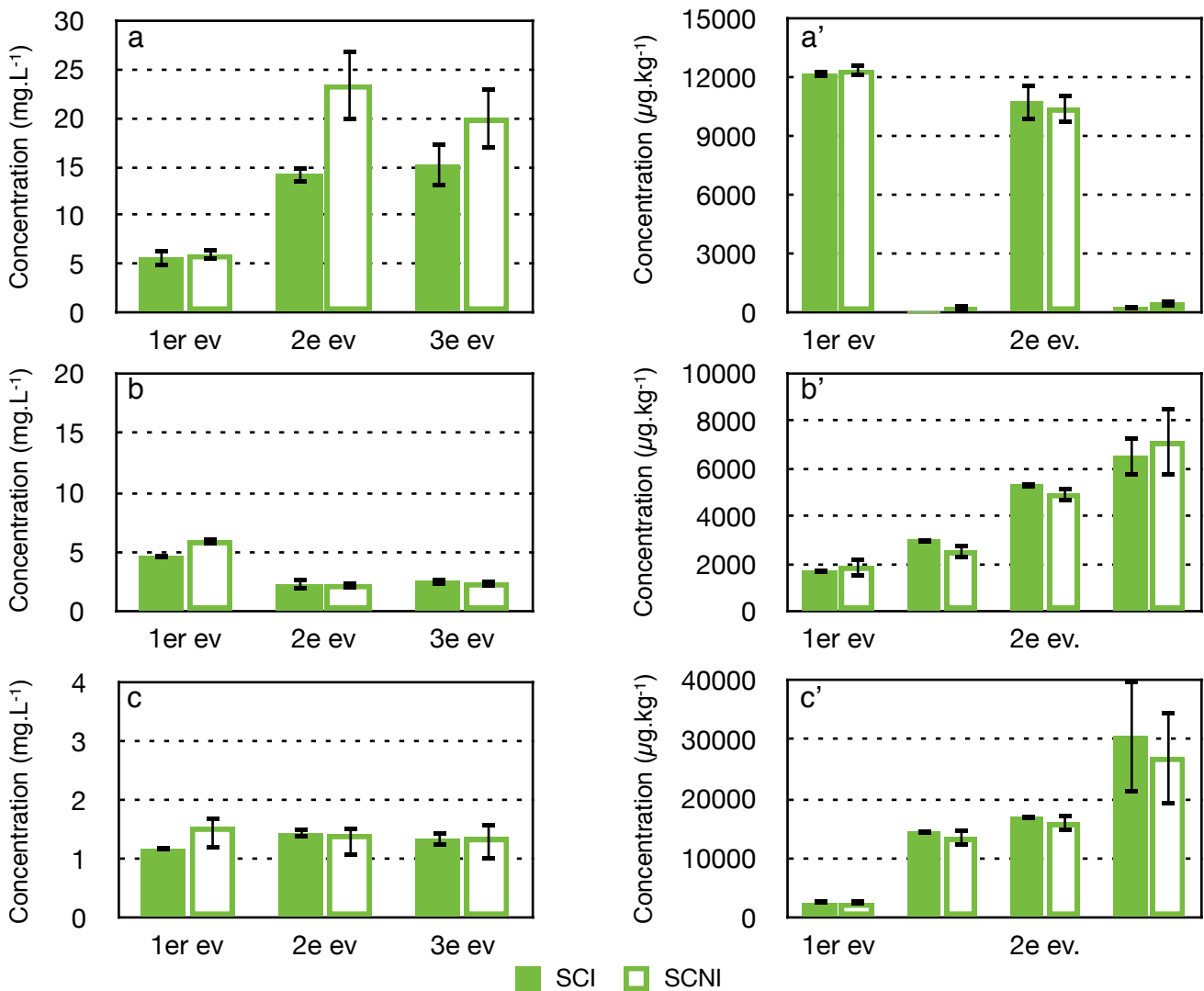
Figure III.30 : Evolution de la concentration en polluants dans l'eau et dans le mélange sable-sédiment (Expérience V). A gauche figure l'évolution des concentrations dans l'eau, à droite la concentration dans le mélange sable-sédiment. a, a' : glyphosate ; b, b' : diuron ; c, c' : 3,4-DCA. SCI : modalité semi-continue inoculée, SCNI : modalité semi-continue non inoculée. Le tf est prélevé une semaine après le dernier événement pluvieux. Les barres d'erreur représentent les erreurs-types.
