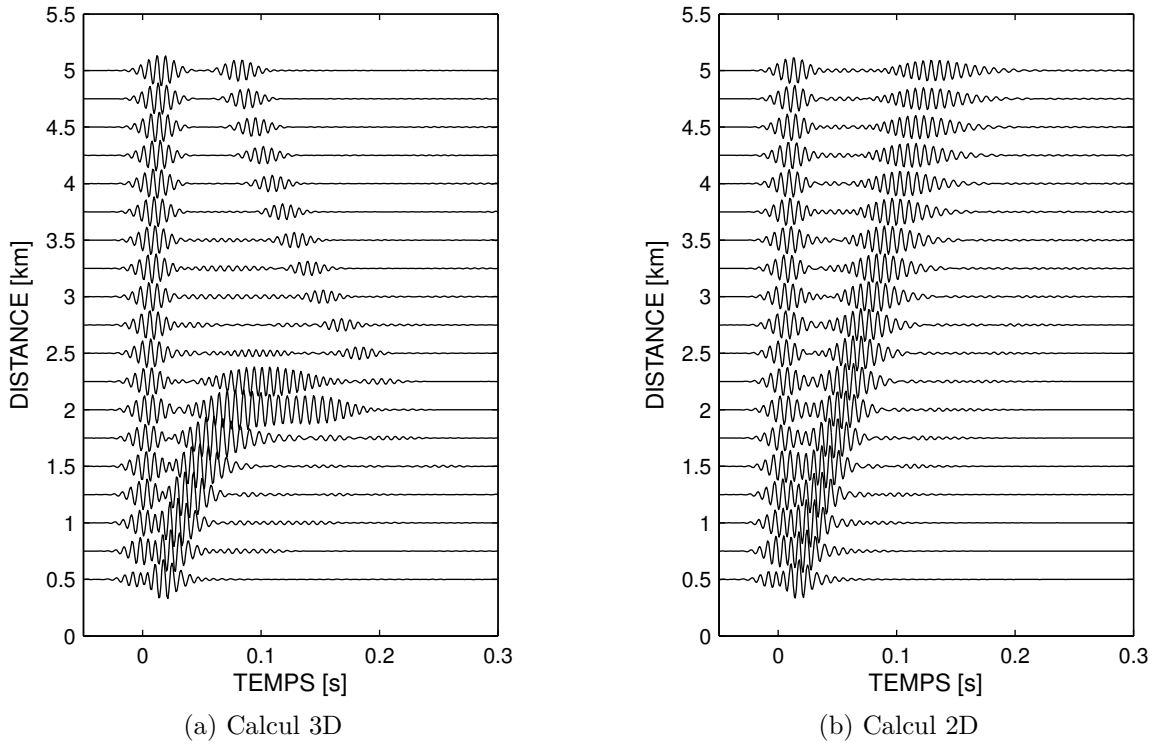
FIG. 2.27 – Prédiction numérique (code 3DWAPE) pour les signaux temporels reçus en fonction de la distance, pour une immersion de récepteur de 26 m. (a) Calcul 3D et (b) calcul 2D. L’immersion de la source est z_S = 10 m).
