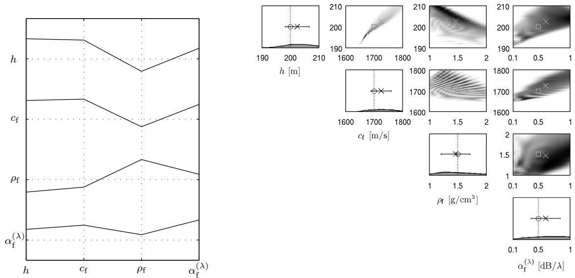
FIG. B.3 – Corrélations entre paramètres (à gauche) et densités marginales a posteriori 1D (à droite en diagonale) et 2D (à droite hors diagonale) pour une antenne verticale située à une distance de 5 km pour une fréquence de 15 Hz.
