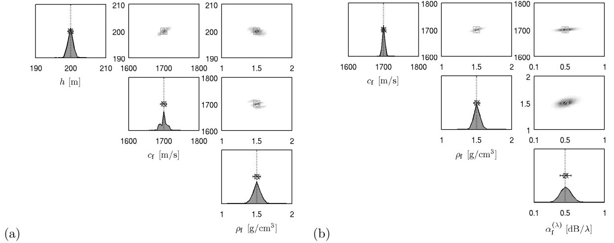
FIG. 3.13 – Densités marginales 1-D et 2-D pour (a) \mathbf{m} = [h, c_f, \rho_f]^T et (b) \mathbf{m} = [c_f, \rho_f, \alpha_f^{(\lambda)}]^T pour une antenne verticale placée à une distance de 5 km et pour une fréquence de 25 Hz.
