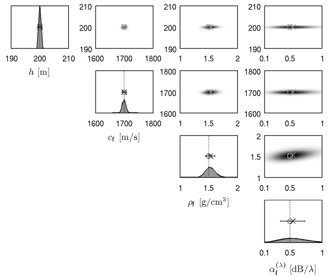
FIG. B.13 – Corrélations entre paramètres (à gauche) et densités marginales a posteriori 1D (à droite en diagonale) et 2D (à droite hors diagonale) pour une antenne verticale située à une distance de 0.5 km pour une fréquence de 100 Hz.
