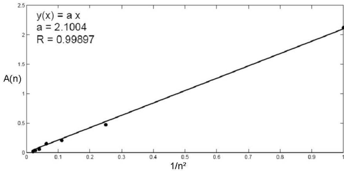
FIGURE 6.15 – fit de A(n) en fonction de n^{-2} .
