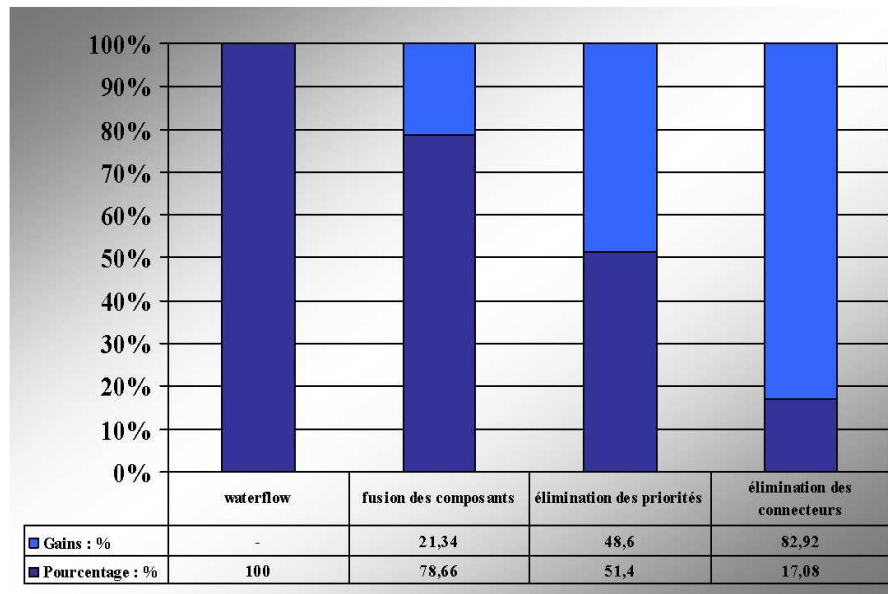
FIG. 7.15 – Évaluation des gains des techniques d'optimisations
