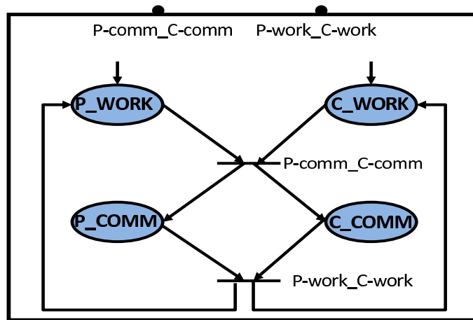
FIG. 7.8 – Architecture du système après la fusion
