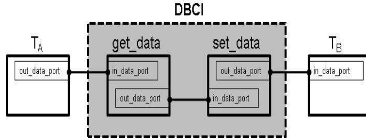
FIG. 6.6 – Communications entre les threads et DBCI
