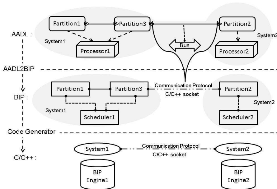
FIG. 6.9 – Déploiement d’une application répartie
