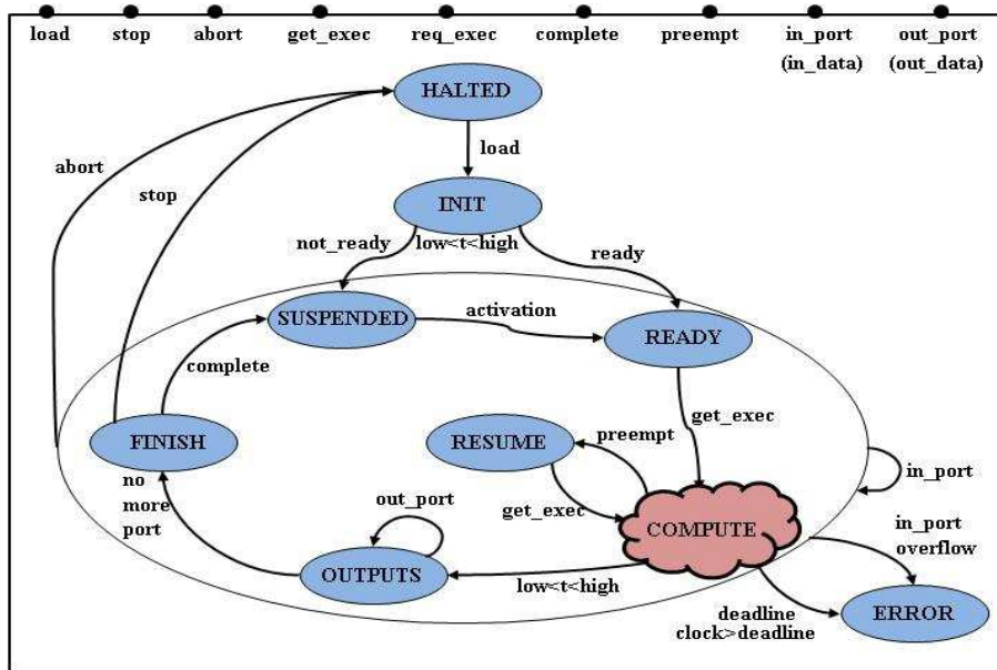
FIG. 5.7 – Traduction du thread vers BIP
