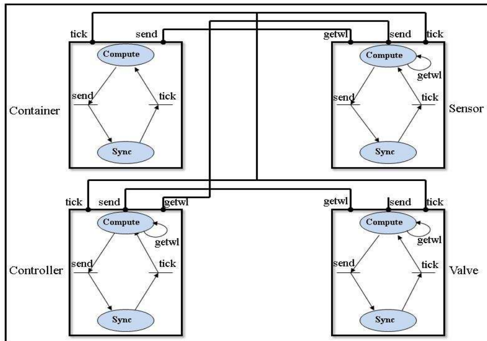
FIG. 7.9 – Le modèle du WaterFlow
