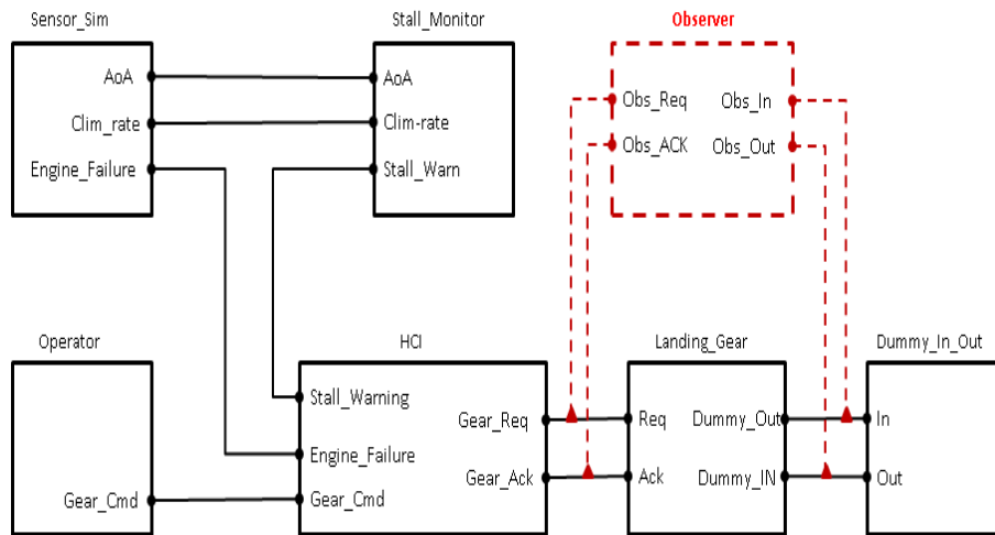
FIG. 8.5 – Le modèle BIP du Flight Computer (comportant le composant observateur en pointillés)
