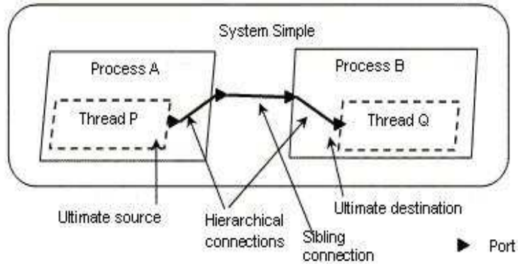
FIG. 3.6 – Les connexions de port
