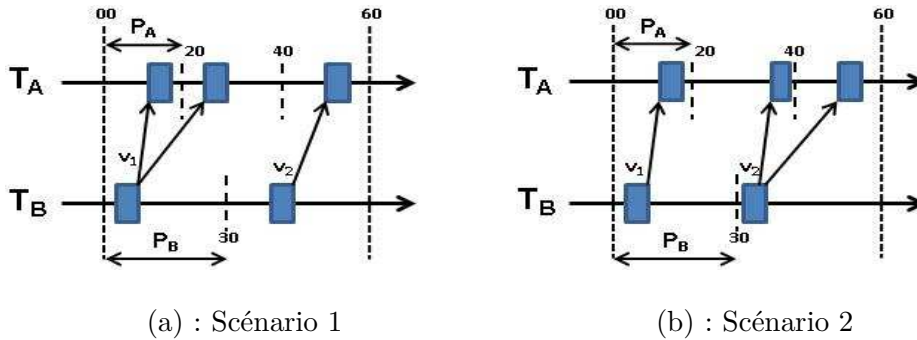
FIG. 6.2 – Non-determinisme : Connexion immédiate
