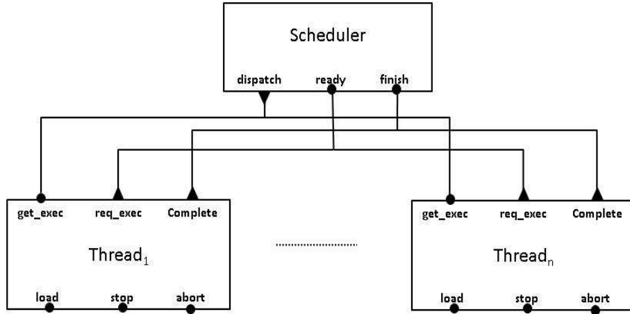
FIG. 5.14 – Représentation en BIP des connexions entre l’ordonnanceur et les threads
