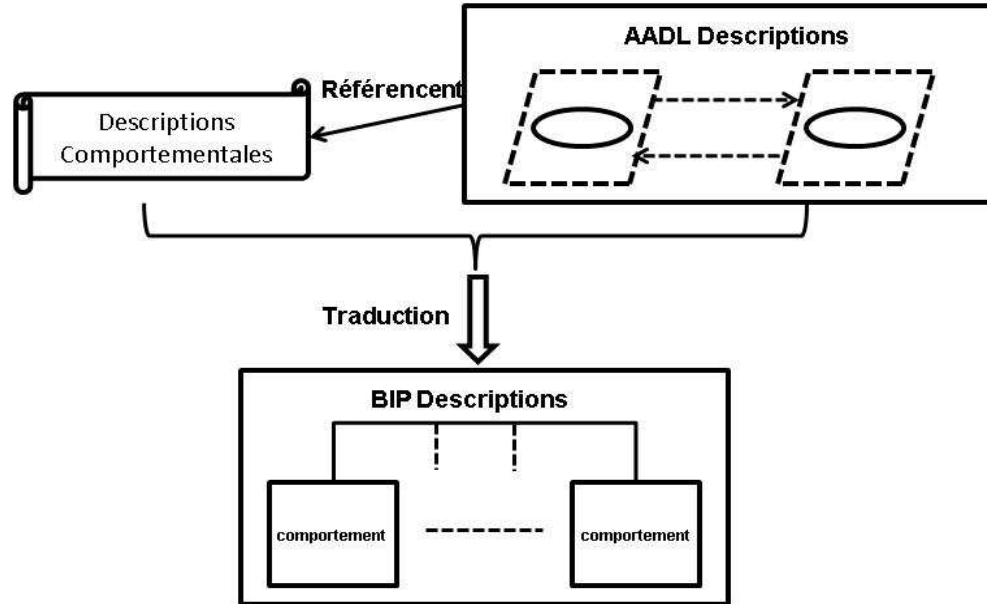
FIG. 5.2 – Génération de l'application BIP
