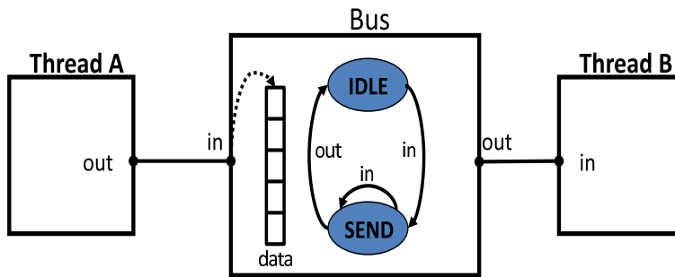
FIG. 5.16 – Modélisation du bus en BIP
