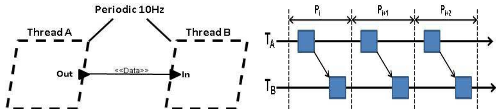
FIG. 3.7 – Connexion Immédiate
