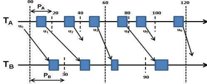
FIG. 6.4 – Protocole de communication pour une connexion immédiate
