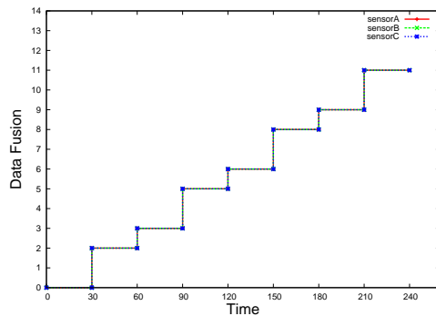
FIG. 8.8 – Avec DBCI
