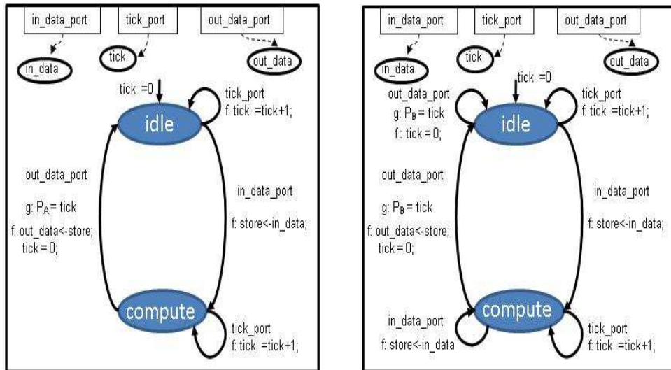
(a) : get_data
