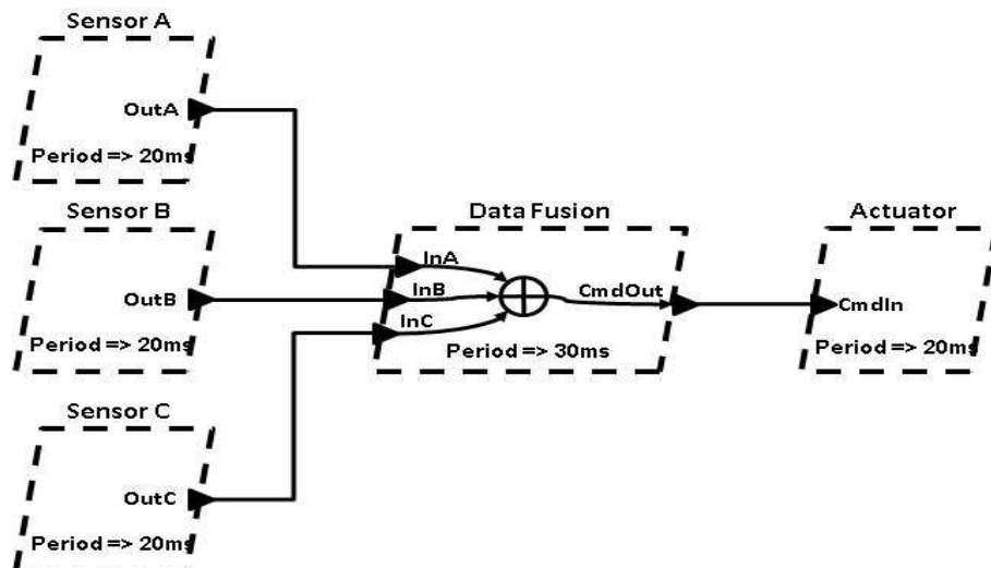
FIG. 8.7 – Système de contrôle
