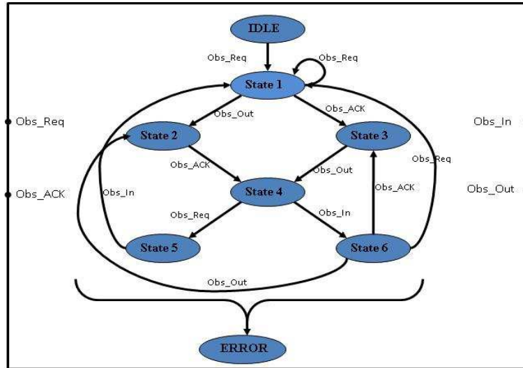
FIG. 8.6 – Le comportement du composant observateur
