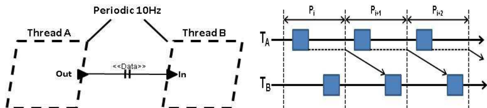
FIG. 3.8 – Connexion Retardée
