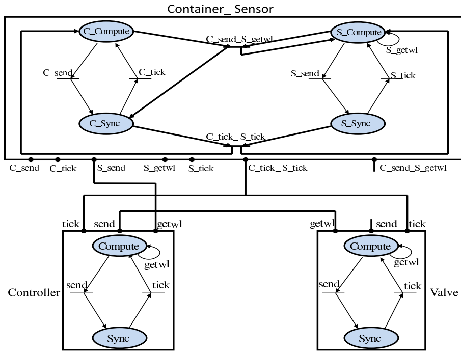
FIG. 7.11 – Fusion de deux composants
