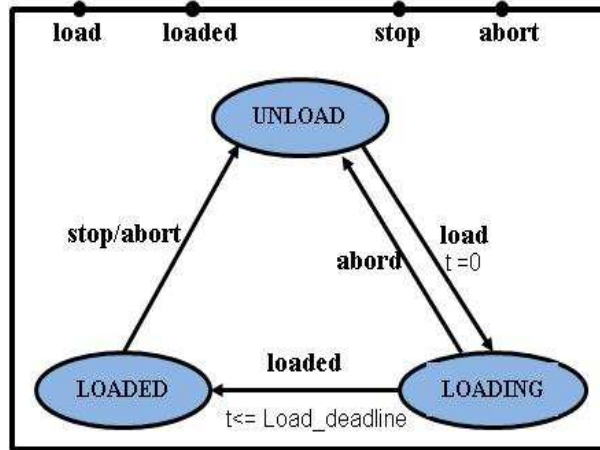
FIG. 5.11 – Modélisation du processus en BIP
