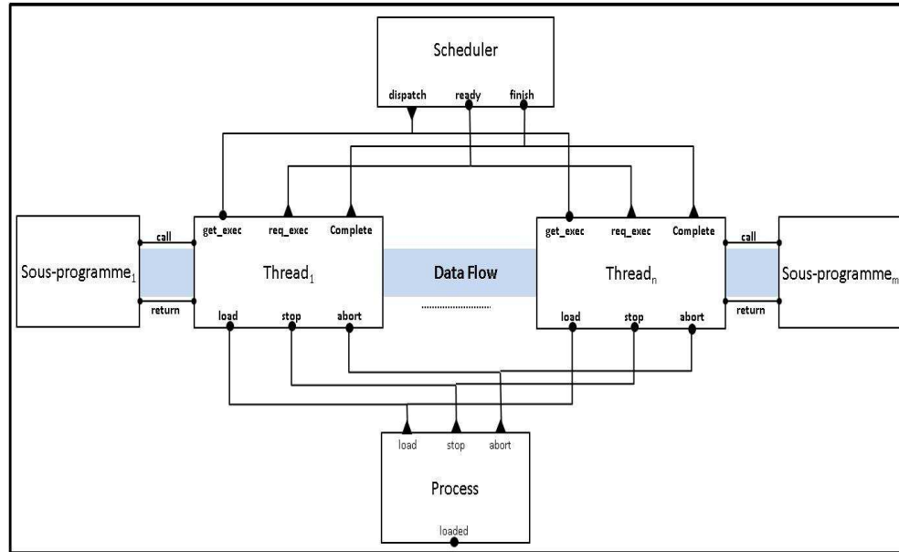
FIG. 5.18 – Représentation graphique d'un système en BIP
