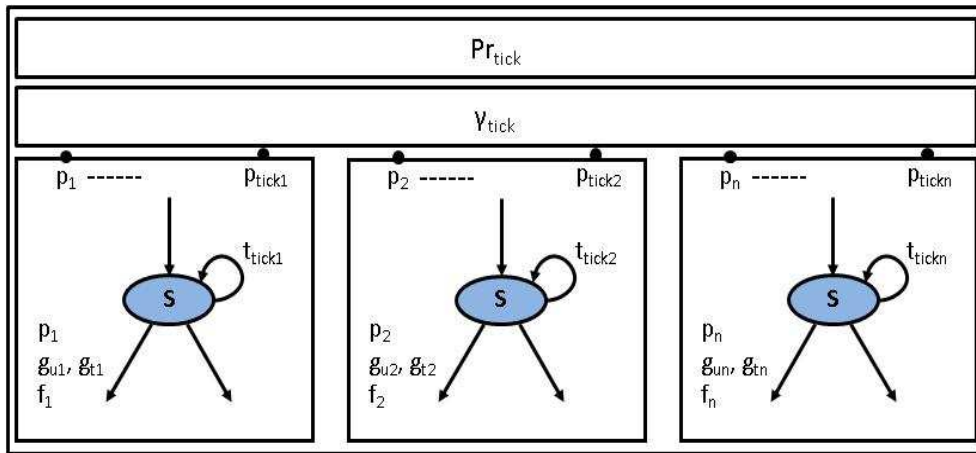
FIG. 7.4 – Composition du composants non temporisé
