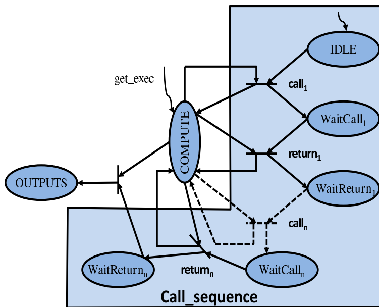
FIG. 5.10 – Séquences d'appel du thread en BIP
