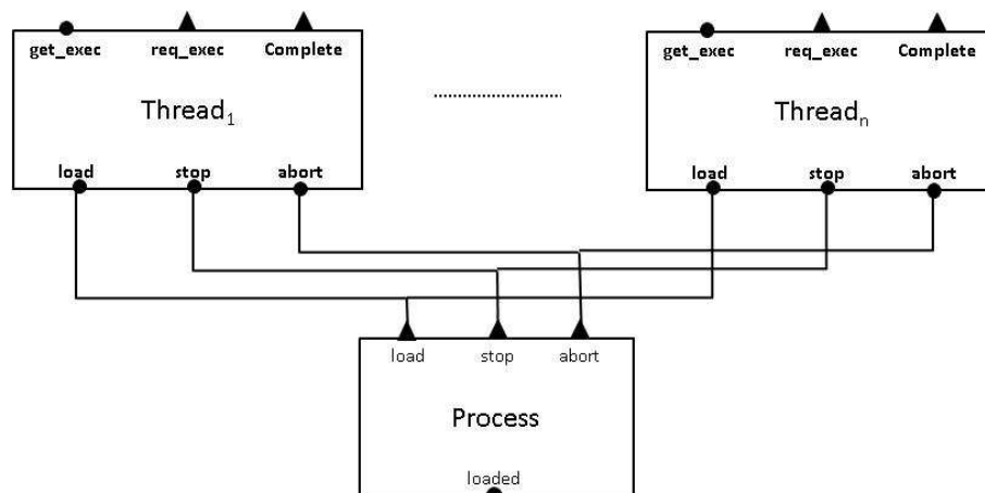
FIG. 5.12 – Représentation en BIP des connexions entre le processus et les threads
