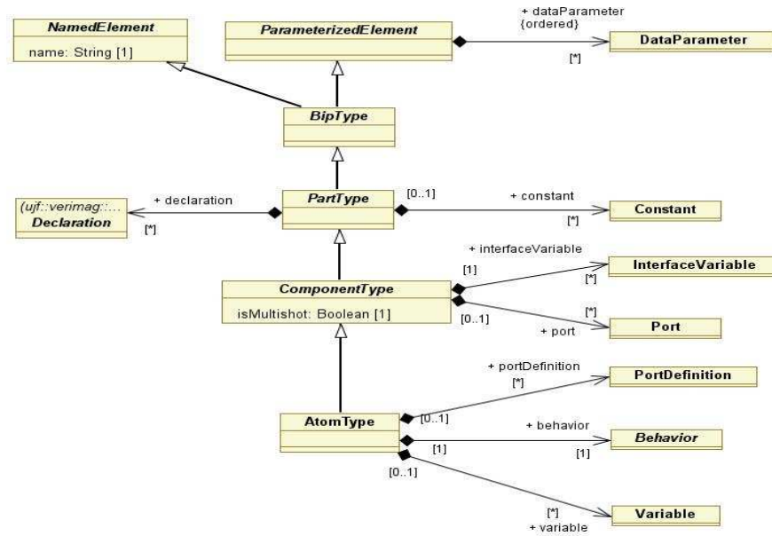
FIG. 8.2 – La représentation des atomes dans le méta-modèle
