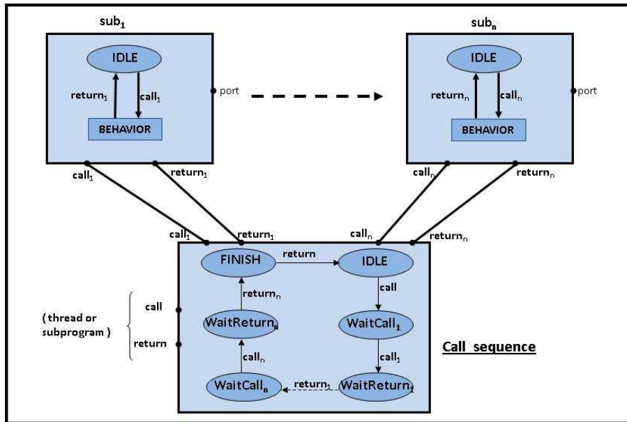
FIG. 5.6 – Traduction du séquences d'appel vers BIP
