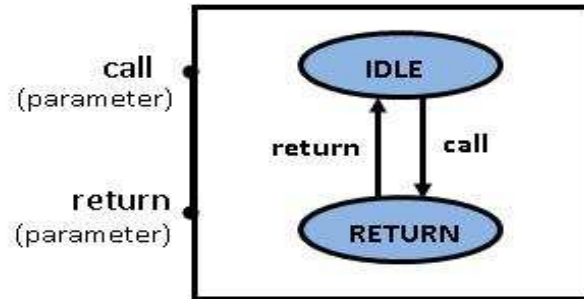
FIG. 5.3 – Sous-programme sans implantation
