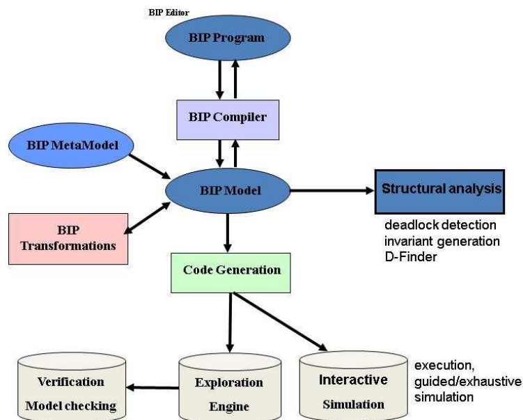
FIG. 4.5 – Chaîne d'outils
