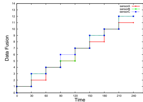
FIG. 8.9 – Sans DBCI
