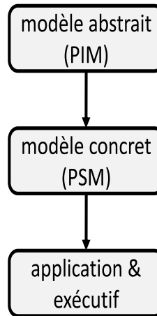
FIG. 1.1 – L’approche MDA
