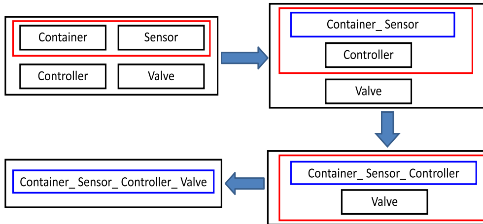
FIG. 7.10 – Fusion binaire
