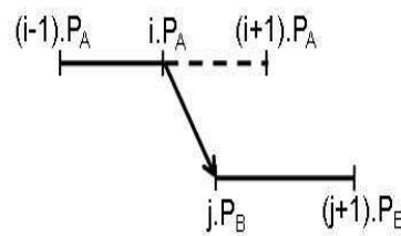
FIG. 6.3 – Deuxième règle
