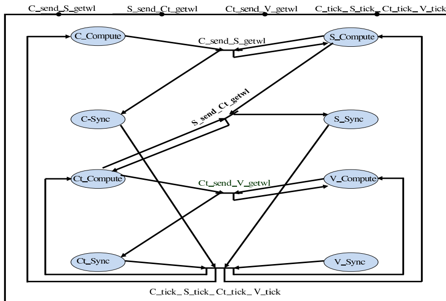
FIG. 7.12 – Fusion n-aire
