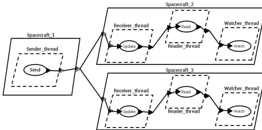
FIG. 8.10 – Vue logicielle de MPC
