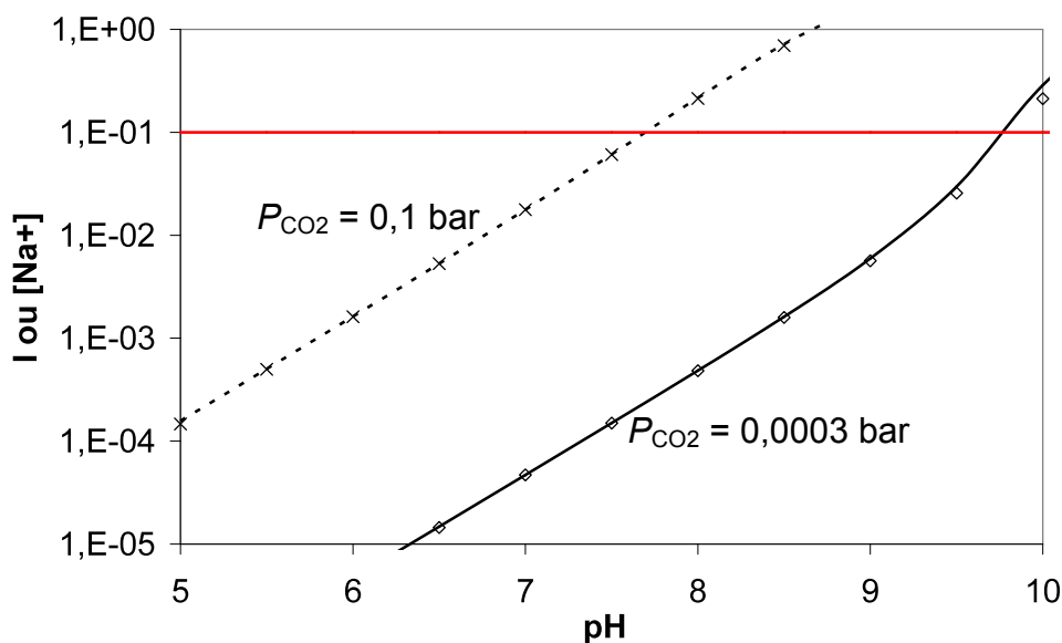
Figure 1 : Evolution de la force ionique dans le système Na-CO 2 -H 2 O pour deux P_{\text{CO}_2} . Les symboles représentent la concentration de Na + associée, calculée d'après l'équation (24).
