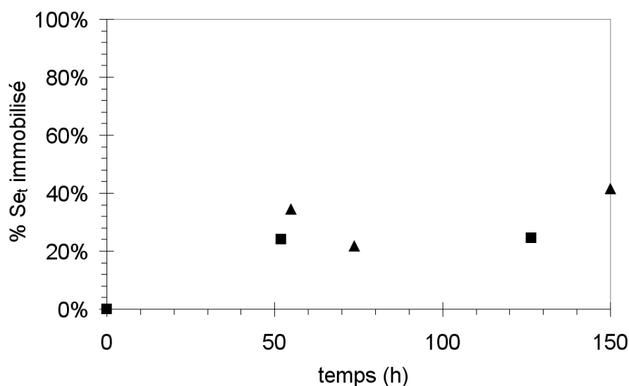
Figure 12 : Cinétique de rétention de Se(IV) dans le blanc expérimental pour Se_t = 9,1 \cdot 10^{-4} \text{ mol.L}^{-1} (▲) et 9,9 \cdot 10^{-5} \text{ mol.L}^{-1} (■).
