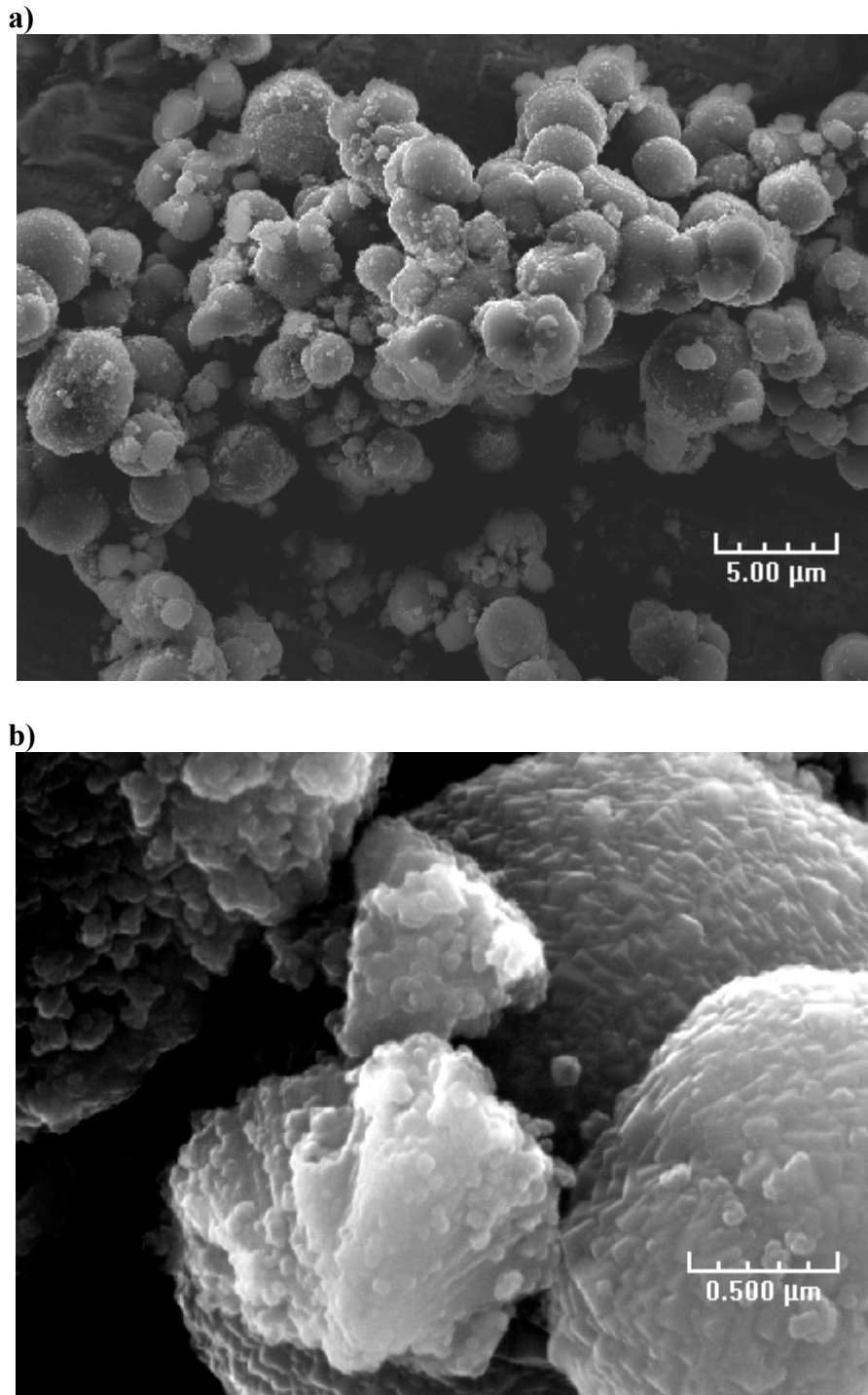
Figure 8 : Clichés MEB de poudre de sidérite synthétique (synthèse n°2) réalisés en électrons secondaires. a) grandissement \times 3500 , b) grandissement \times 43000
