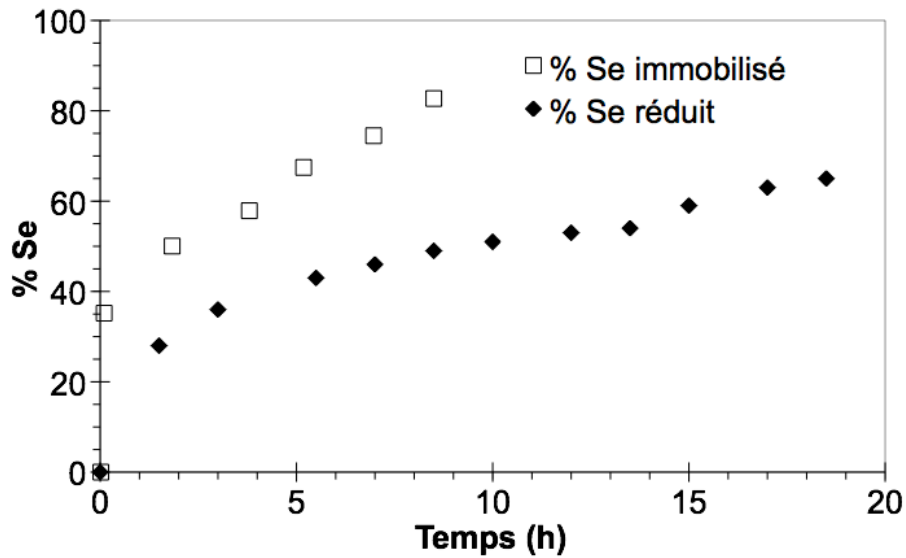
Figure 20 : Pourcentage de sélénium réduit in situ en présence de sidérite en fonction du temps pour Se_I = 1,0 \cdot 10^{-3} \text{ mol.L}^{-1} de Se(IV) dans une suspension de sidérite (voir Tableau 10), accompagné du pourcentage de sélénium immobilisé en présence de sidérite pour Se_I = 7,4 \cdot 10^{-4} \text{ mol.L}^{-1} (voir figure 11).
