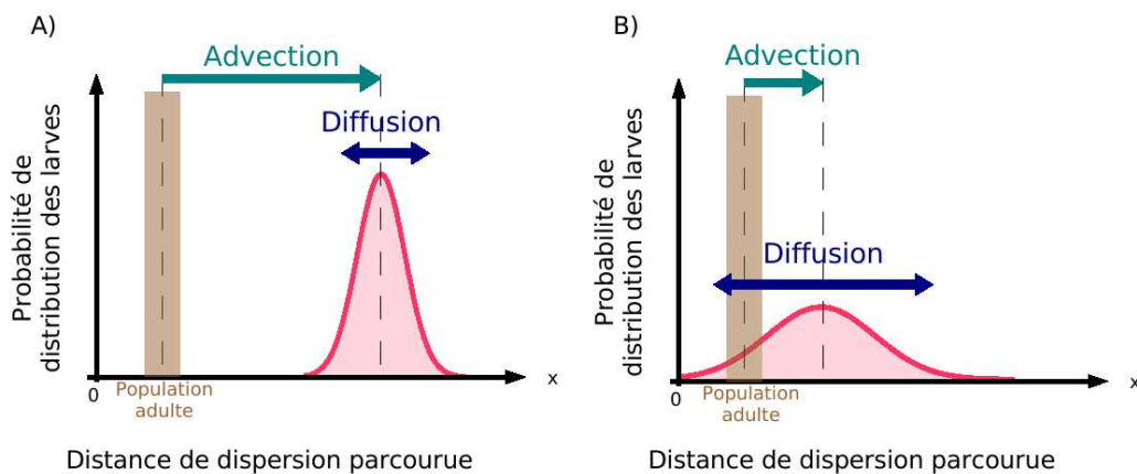
Figure I.6 – Conséquences de l'advection et de la diffusion turbulente sur la distribution des larves. (A) Conséquences d'une advection forte et d'une diffusion faible sur le noyau de dispersion. (B) Conséquences d'une diffusion forte et d'une advection faible sur le noyau de dispersion. Les processus d'advection sont représentés par une flèche turquoise et les processus de diffusion par une double flèche bleue. La localisation du site d'émission des larves au-dessus de la population adulte est représentée en marron et les noyaux de dispersion en rose.
