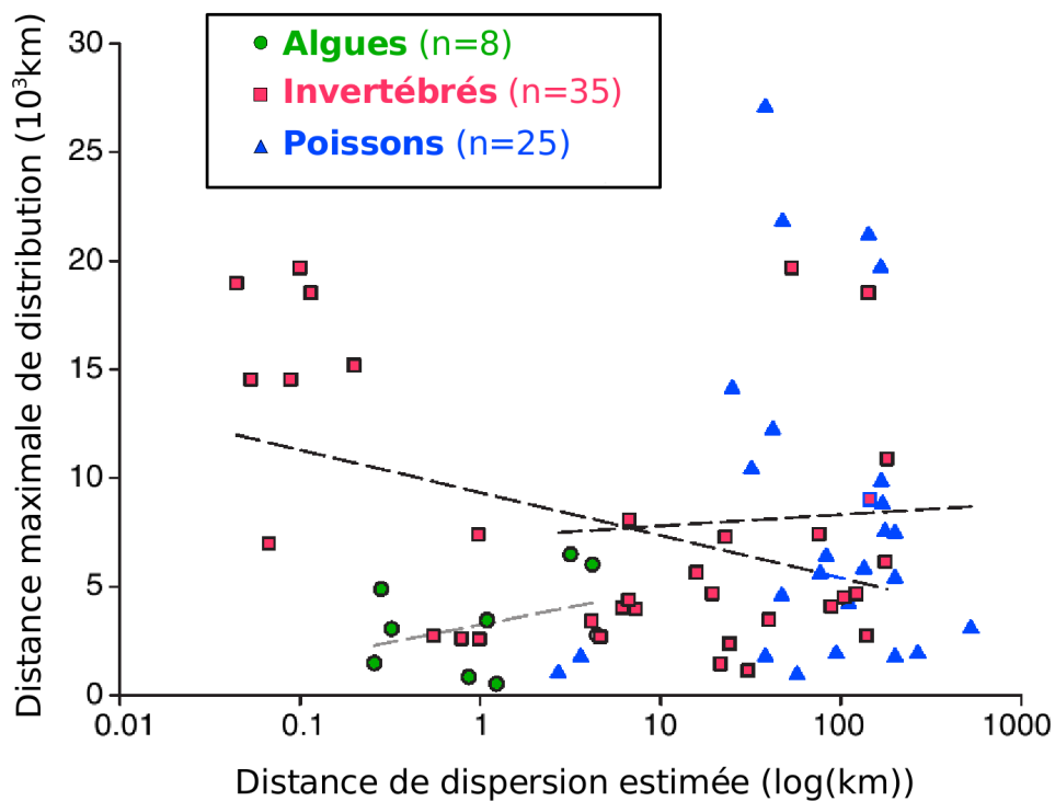
Figure I.24 – Relation entre l'aire de distribution des espèces marines ( i.e. distance linéaire maximale entre les limites d'aire de distribution de l'espèce) et la distance de dispersion efficace estimée à partir de données génétiques, d'après Lester et al. (2007). Pour chaque groupe taxonomique ( i.e. algues, invertébrés, poissons), la relation représentée par une ligne pointillée est non significative.
