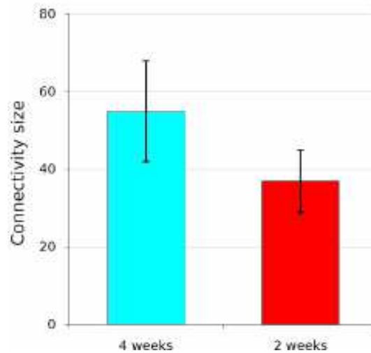
FIG. 3.4 – Conséquence d’une diminution de la durée de vie larvaire de 4 à 2 semaines sur la taille de connectivité. Les moyennes sont calculées pour 35 dates de ponte et 16 populations. La taille de connectivité est définie comme le nombre de connections obtenues dans les matrices de connectivité entre les 16 populations.
