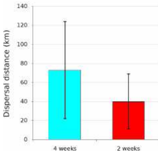
FIG. 3.3 – Conséquence d’une diminution de la durée de vie larvaire de 4 à 2 semaines sur la distance de dispersion orthodromique moyenne. Les moyennes sont calculées pour 35 dates de ponte et 16 populations.
