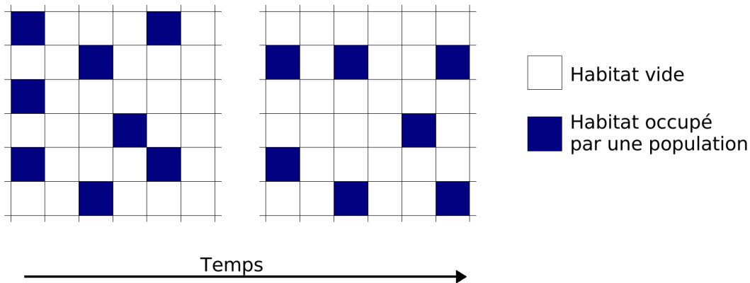
Figure I.12 – Modèle de métapopulation de Levins (1969), composé d'un maillage infini de fragments d'habitat (carrés) équidistants et de mêmes caractéristiques. Les fragments d'habitat sont vides (en blanc) ou occupés par une population locale (en bleu).
