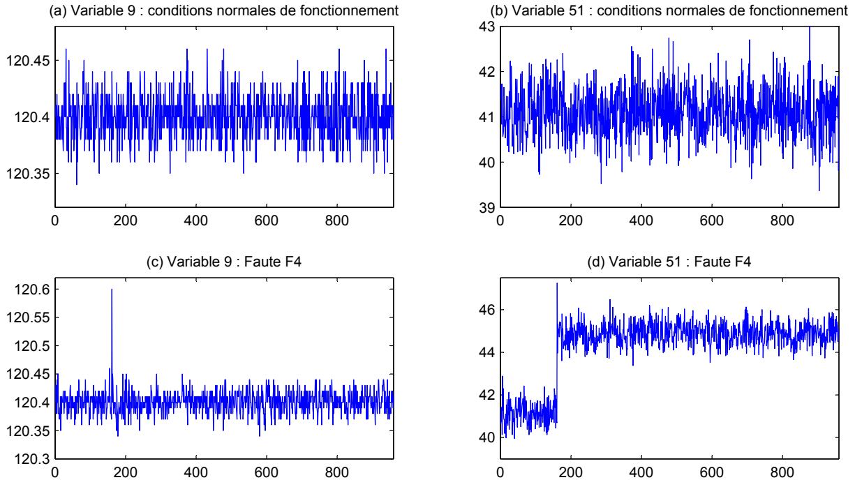
FIG. 4.3 – Comparaison des variables 9 (XMEAS9) et 51 (XC10) pour le fonctionnement normal et pour la faute F4
