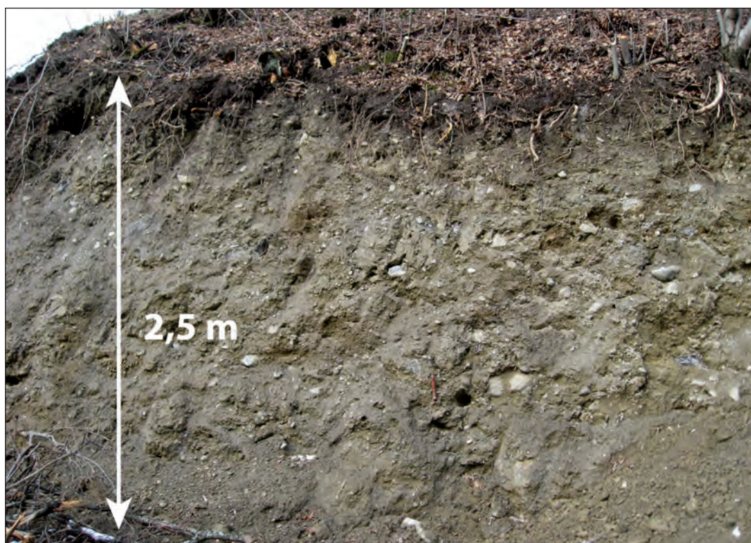
Fig. III. 18 – Coupe d'une moraine latérale : la diamictite est visible à la faveur d'une incision pratiquée pour la construction d'une route (Combloux, Haute-Savoie) ;
