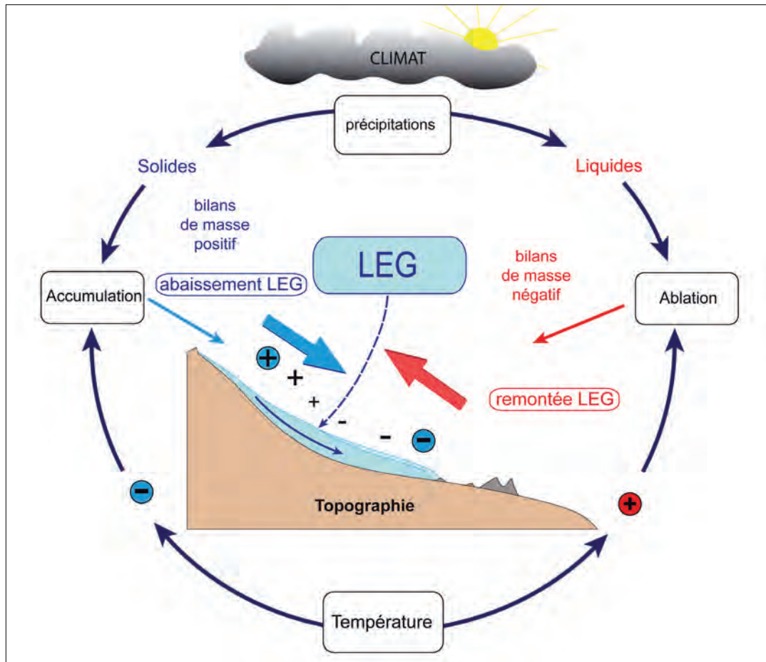
Fig. 1.1 - Schéma - approche systémique de la LEG : à droite de la figure, les différents paramètres influençant la remontée de la LEG. À gauche de la figure les paramètres favorisant l'abaissement de la LEG. La durée de fonctionnement contraint les deux processus.
