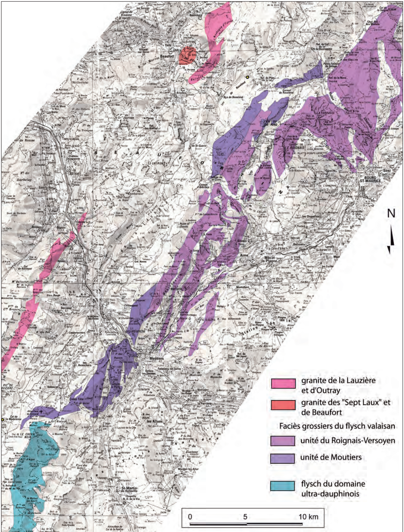
Fig. 2. 25 – Carte de localisation des flyschs des zones valaisannes (unités de Moutiers et du Roignais-Versoyen) et ultra-dauphinoises.
