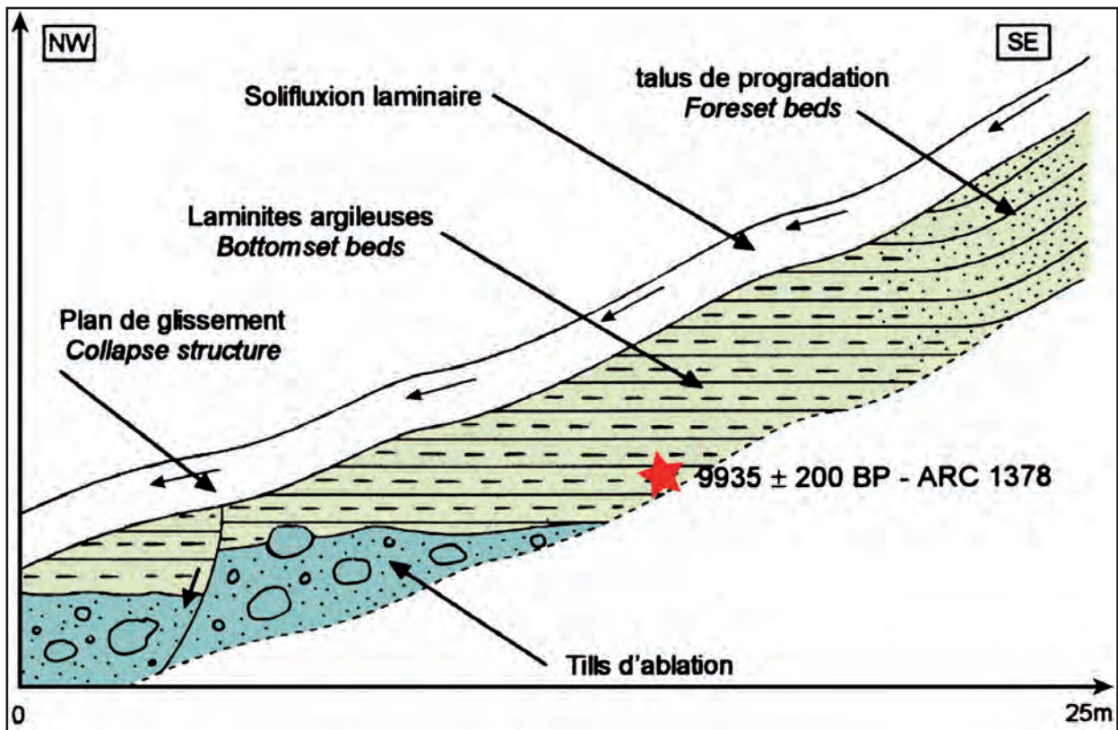
Fig. II. 58 - Coupe stratigraphique de la formation lacustre et de la moraine des Frasserands (Lucena, 1998 ; Jaillot et Ballandras, 1999), colorisé.
