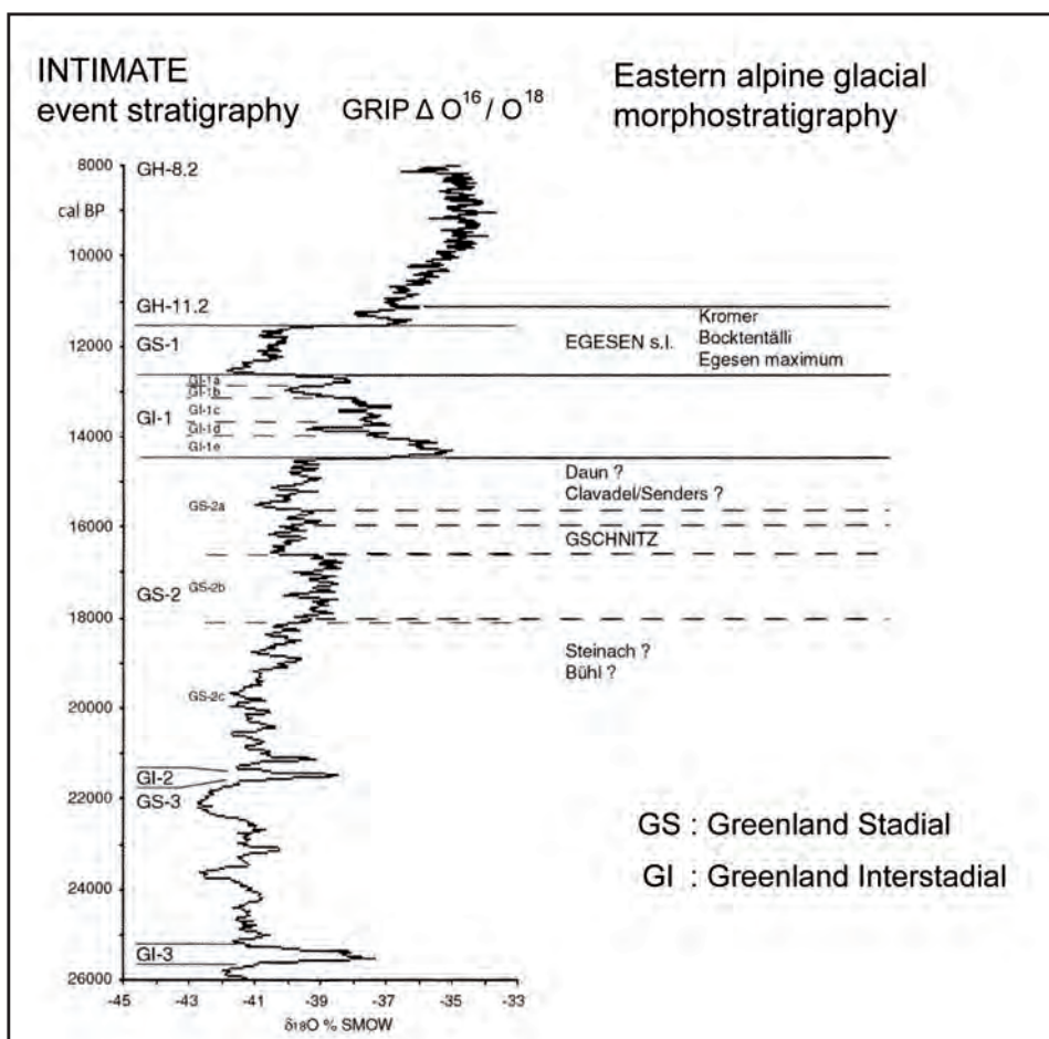
Fig. II. 57 - Hypothèse de corrélation des stades tardiglaciaires des Alpes orientales avec la stratigraphie INTIMATE, basée sur la courbe GRIP (Schoeneich, 2003).
