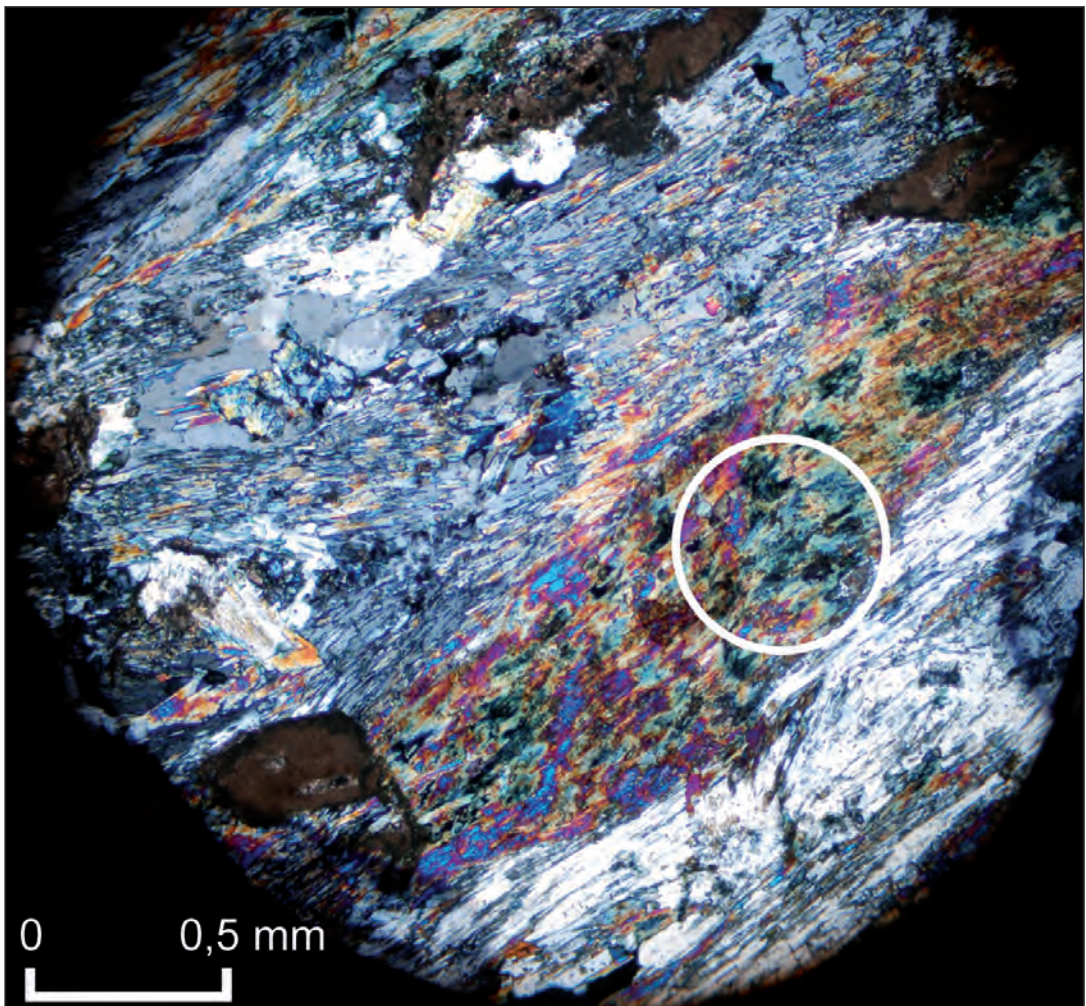
Fig. 2. 40 - Détail d'une lame mince de métagabbros : la lame montre bien le litage métamorphique ainsi que le remplacement des pyroxènes par des assemblages à amphiboles, chlorite et talc (cercle blanc).
