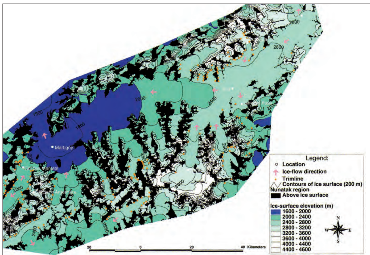
Fig. II. 6 - Reconstitution paléogéographique du Valais d'après Kelly (Kelly et al. 2004).
