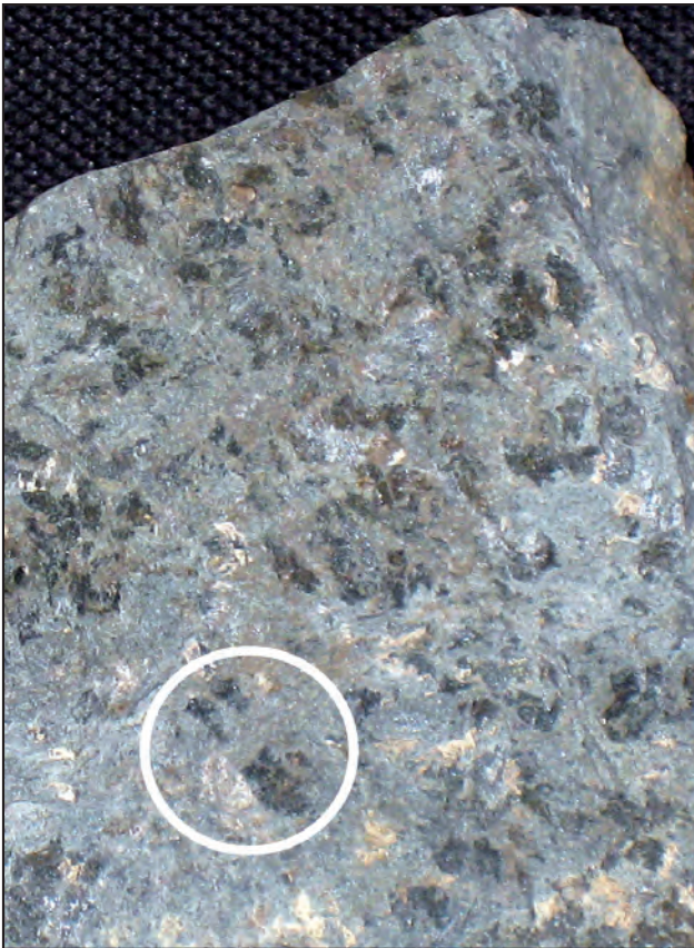
Fig. 2. 39 - Détail macroscopique d'un bloc erratique de gabbros : l'examen montre des pyroxènes résiduels orientés dans un fond à grain fin difficilement identifiable macroscopiquement.
