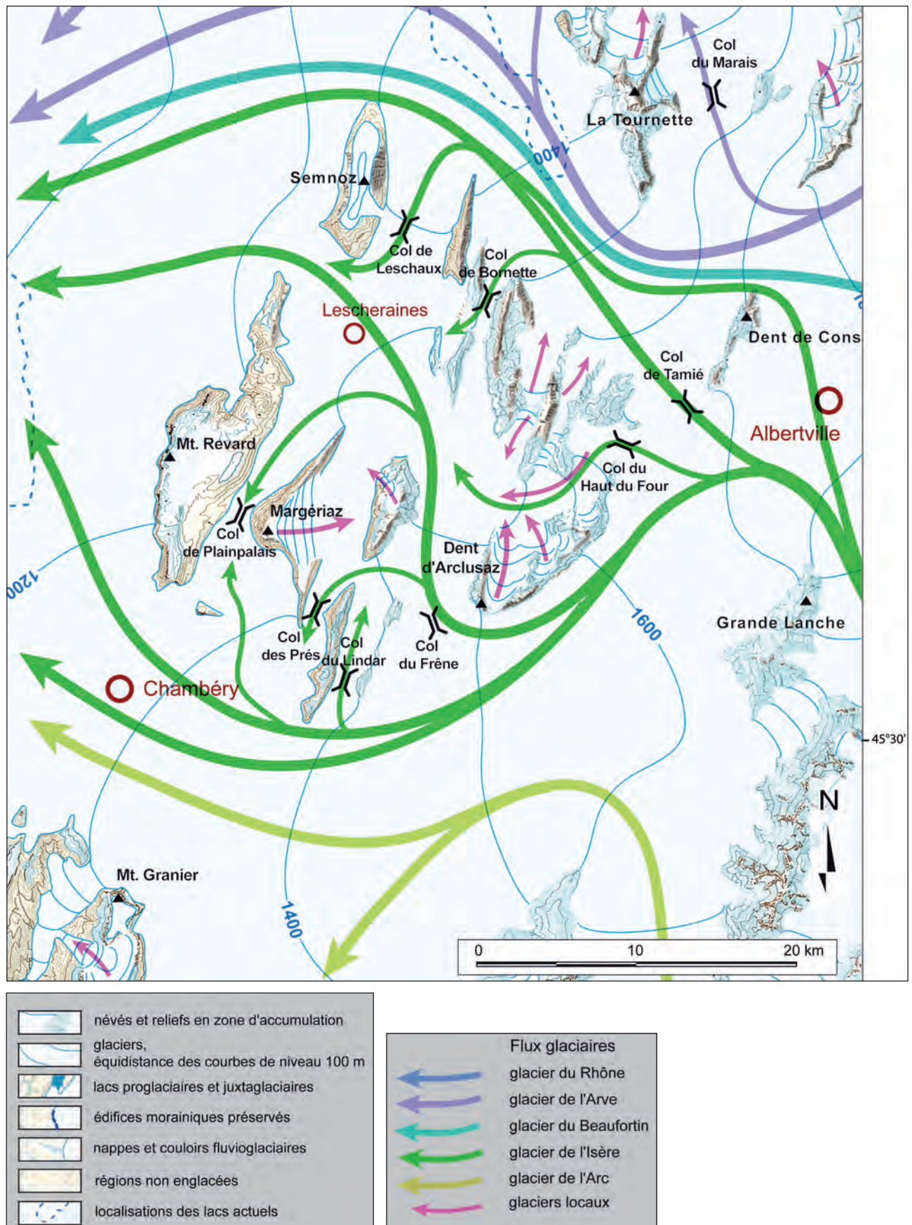
Fig. 4. 28 - Carte paléogéographique du glacier isérois et du massif des Bauges, interprétation des flux glaciaires locaux et alloctones au WGM à partir des données de Revil (1913), Nicoud (1973), Hobléa (1986), Dusseau (1992), Doudoux et al. (1999) et ce travail.
