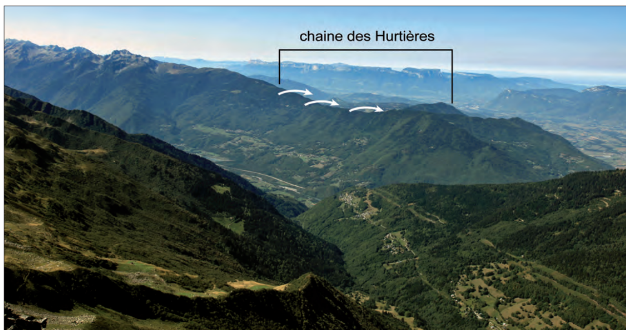
Fig. 3. 17 – La chaîne des Hurlières présente des nombreux sillons d'érosion glaciaire liés au débordement du glacier de l'Arc.
