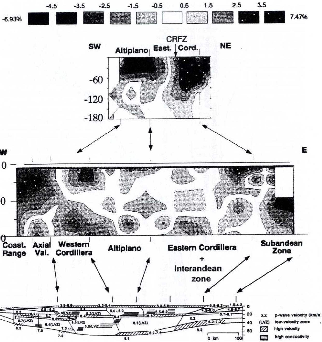
Fig. 94— Compilation des résultats des transects géophysiques le long des Andes Centrales.
