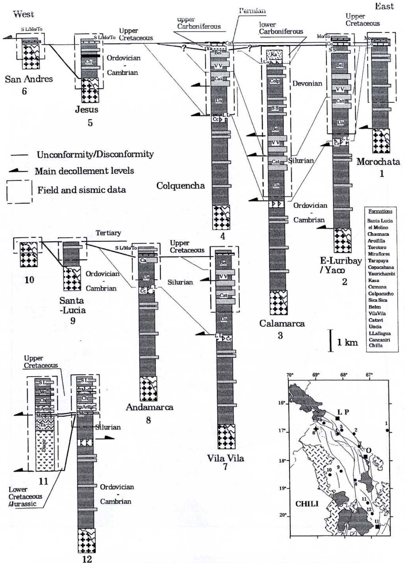
FIG. 10- Corrélations stratigraphiques des séries ante-tertiaires de l'Altiplano
