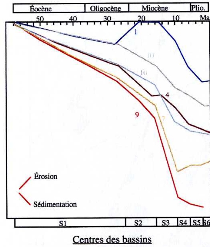
FIG. 67- Subsidence relative comparée des différents bassins de l'Altiplano.
