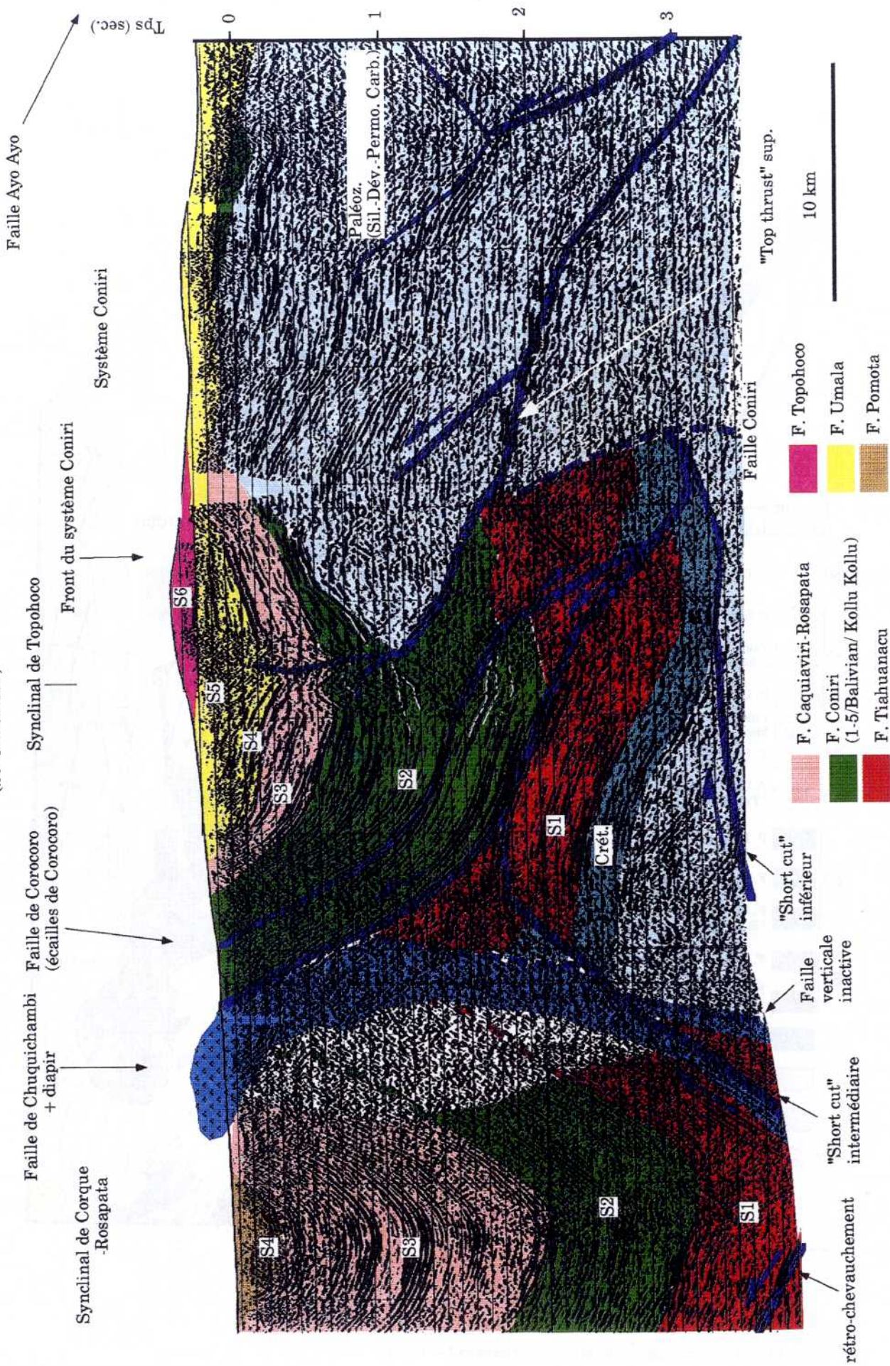
FIG. 49— Coupe de la bordure est du bassin de Corque et du synclinal de Corocoro à la latitude de 17° 15' S (sismique réflexion YPFB).
