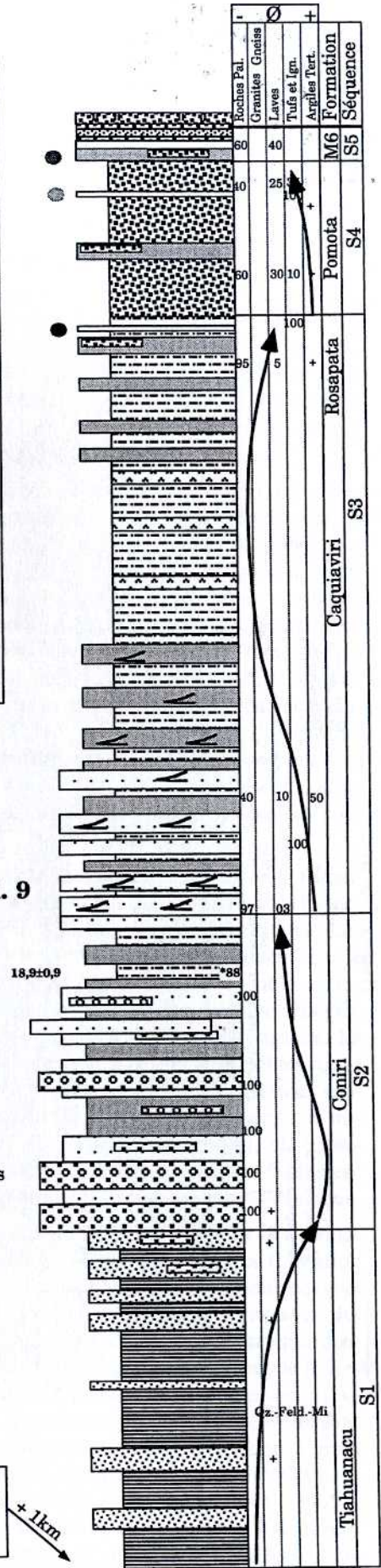
Fig. I. 18: col. lithostratigraphiques du bassin Corque (suite) Légende (cf fig. I.17)
