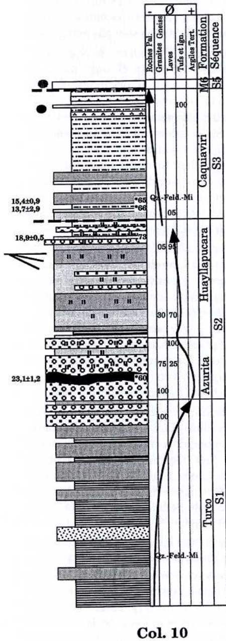
Fig. I. 18: col. lithostratigraphiques du bassin Corque (suite) Légende (cf fig. I.17)
