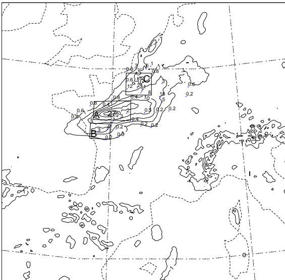
FIG. 4.8 – Précipitations cumulées sur 6 heures, entre 6 et 12 h d'échéance, pour le 03/05/2001. Prédiction de contrôle sans perturbation initiale par un gradient. Les petits chiffres indiquent les cumuls de pluie observés. La valeur "27" dans le carré "A" indique le maximum des cumuls modélisés par Aladin.
