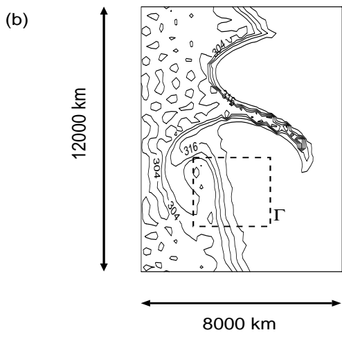
FIG. 2.2 – Température potentielle tous les 4 K, au sol et au toit du modèle semi-géostrophique. La situation correspond au jour 8 de l'évolution de l'onde barocline. (a) surface, (b) toit.
