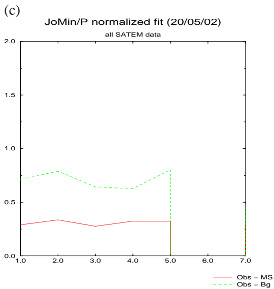
FIG. 3.5 – Evolution temporelle, dans la fenêtre d’assimilation du 4D-VAR Arpège, des écarts au carré observations moins ébauche (trait tireté) et observations moins analyse (trait continu) normés par les variances d’erreur d’observations et le nombre total d’observations par timeslot (tous champs mesurés confondus). (a) radiosondage ( P_{total} \approx 70000 ) ; (b) avion ( P_{total} \approx 36000 ) ; (c) radiances satellite ( P_{total} \approx 23000 ).
