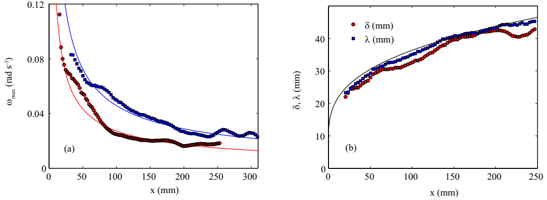
FIG. 2.7 – Diffusion visqueuse d’un faisceau d’onde d’inertie. (a) D clinaison du maximum de l’enveloppe de vorticit  pour 2 valeurs de la vitesse angulaire \Omega , et comparaison avec la pr diction en x^{-2/3} . (b) Largeur   mi-hauteur de l’enveloppe de vorticit  ( \delta ), longueur d’onde apparente ( \lambda ), et comparaison avec la solution de similitude (2.8) incluant l’effet de taille finie de la source (d’apr s Cortet et al. (2010) [36]).
