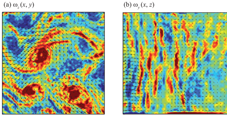
FIG. 3.6 – Champs de vorticit  dans le plan horizontal (a) et vertical (b), obtenus sur la plateforme Coriolis. Vitesse angulaire \Omega = 0.10 \text{ rad s}^{-1} , tV_g/M \simeq 770 . D'apr s Moisy et al. (2010) [95].
