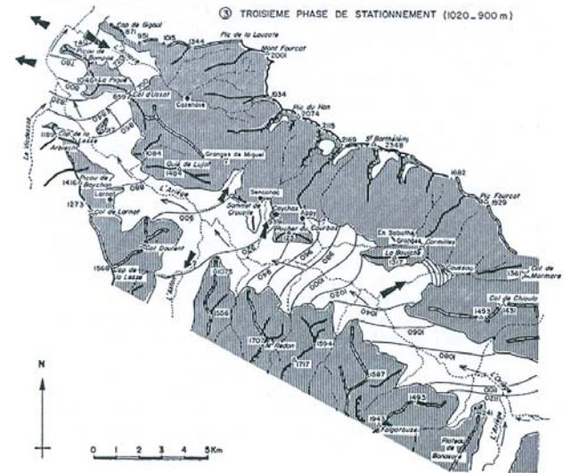
Fig. 5.28 : Les trois phases de stationnement du glacier dans le val d'Ariège (Extrait de Bertrand, 1963)
