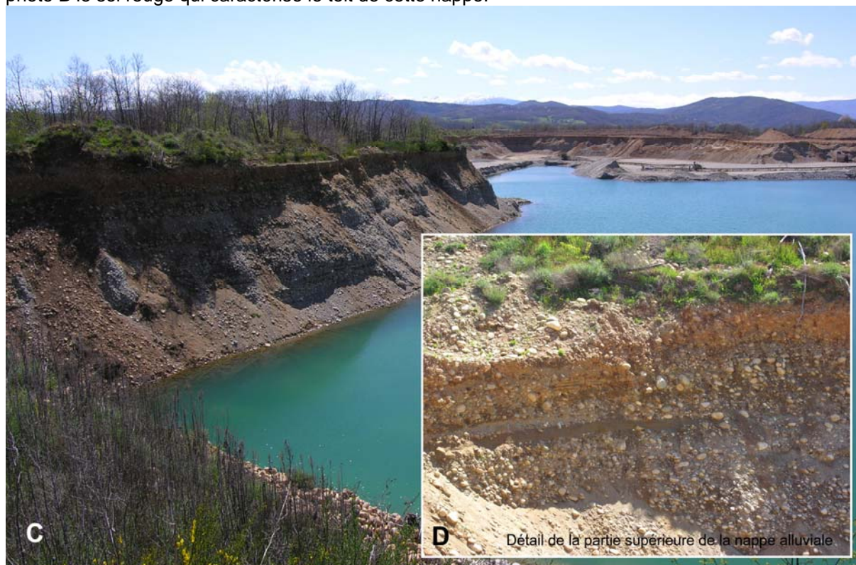
C et D – La Grausse de Pamiers (nappe fluvioglacière T1) au niveau de la gravière de Filatié. Noter sur la photo B le faible état d'altération des blocs et de la matrice.
