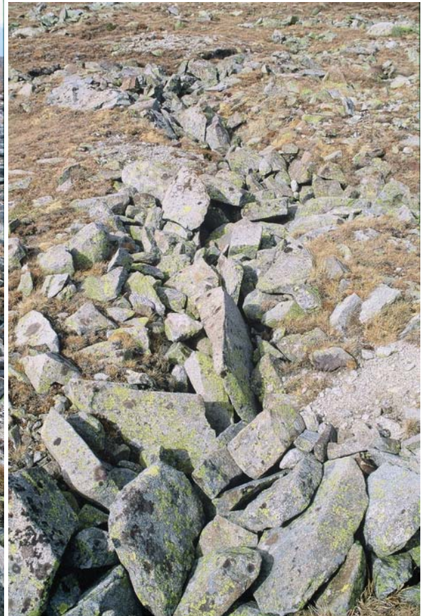
B et C – Polygones périglaciaires attribués au Pléniglaciaire würmien (Soutadé, 1980) et attestant l'absence de recouvrement par la glace.
