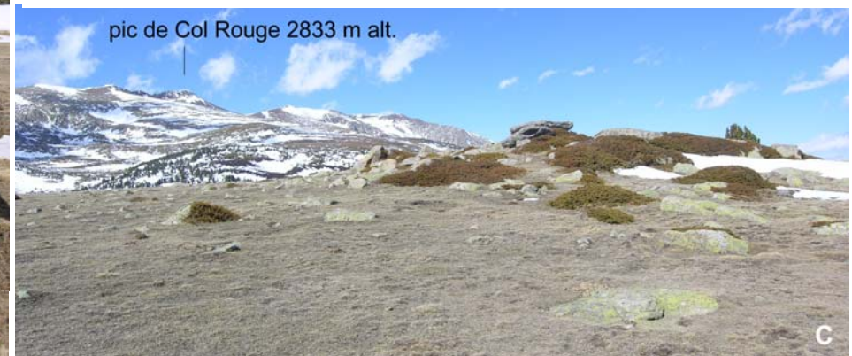
C – Tor démantelé situé en avant du front MEG Würm des Estagnets. Ce tor a probablement été recouvert au cours des cycles glaciaires pré-würmiens mais aucun indice de till n'a permis de le confirmer (idem pour la vasque à encorbellement de la photo B).
