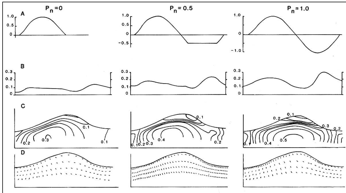
Fig. 1.4 : Variation des champs de contraintes entre l'amont et l'aval d'un obstacle d'après le modèle de Morland & Boulton (1975) (Extrait de Drewy, 1986)
