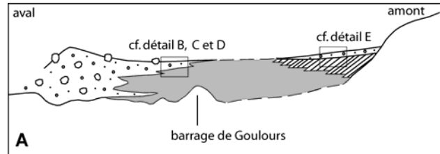
A – Reconstitution stratigraphique du remplissage détritifique de Goulours-La Forge.
