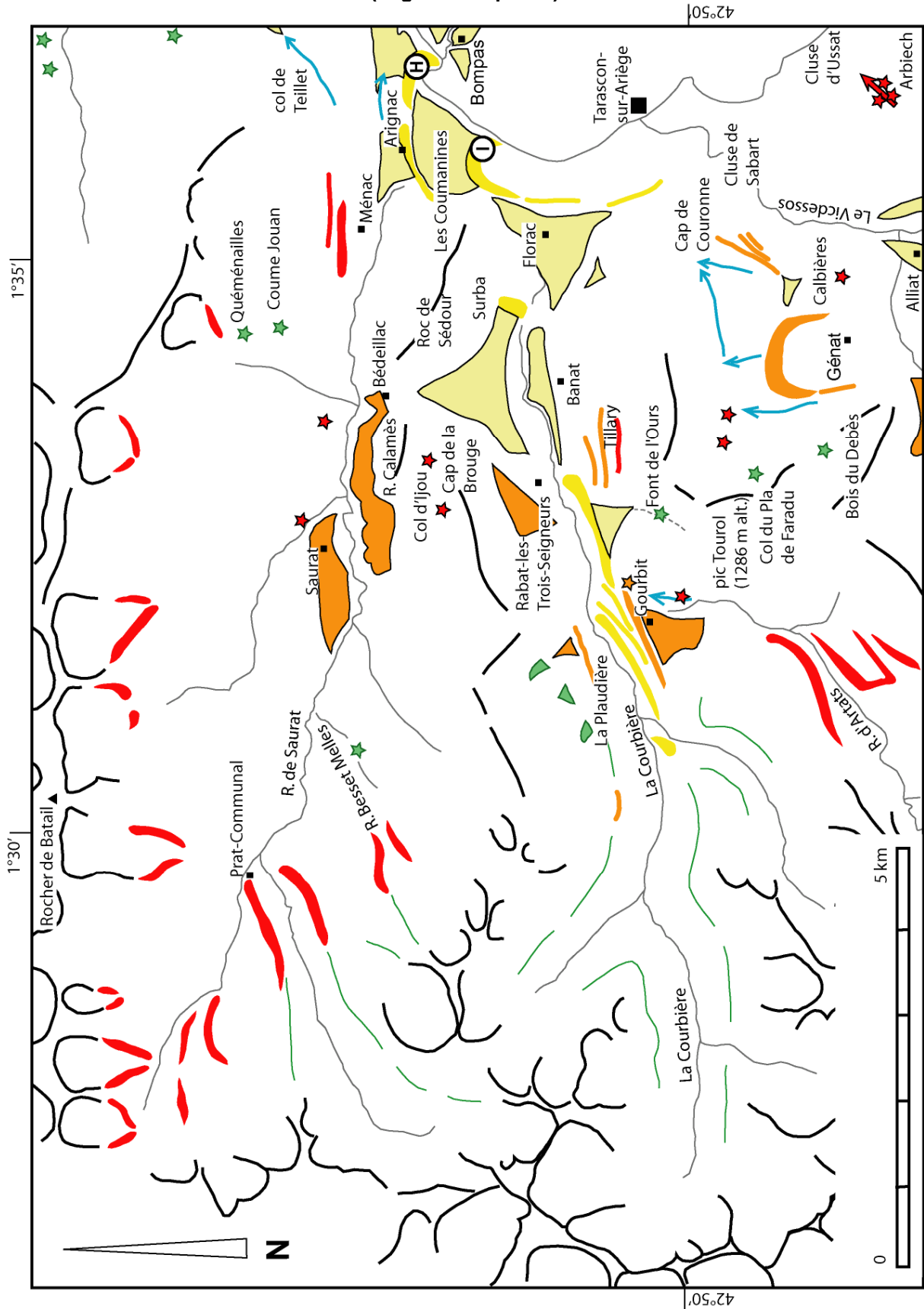
Fig. 5.9 : Carte géomorphologique des formes et dépôts glaciaires : Bassin de Tarascon secteur Ouest (Légende cf. p. 157)
