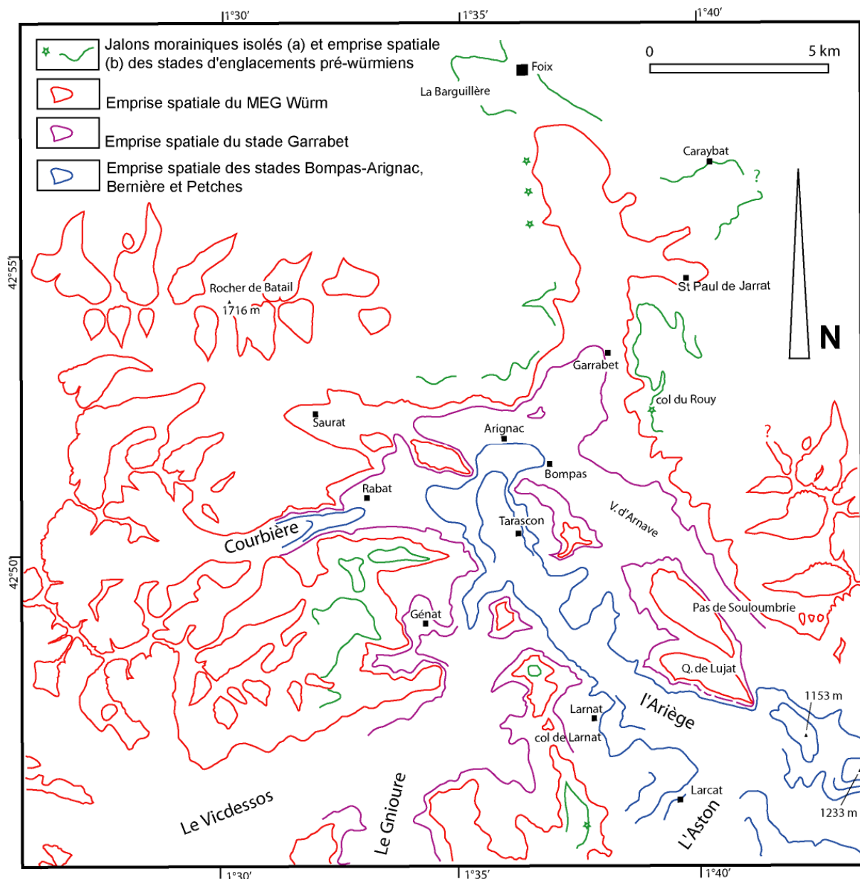
Fig. 5 44 : Emprise spatiale des paléoenglacements würmiens et pré-würmiens secteur aval
