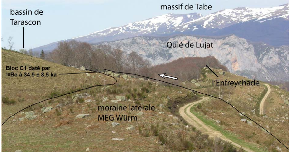
B – Cordon morainique latéral situé à 1400 m et associé au MEG Würm.
