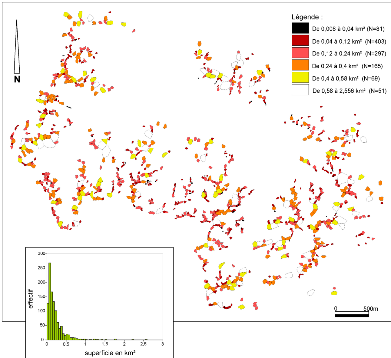
Tabl. 8.9 : Analyse descriptive du paramètre superficie
