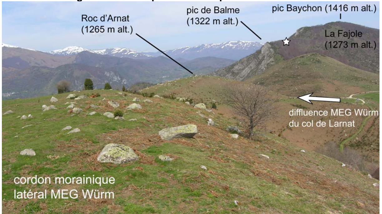
A – Les moraines würmiennes du col de Larnat vues du sud. L'étoile blanche localise le site N.
