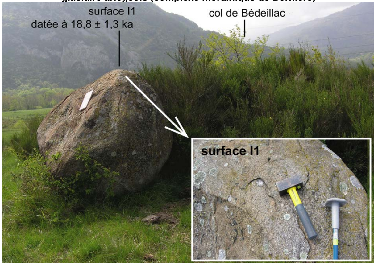
Fig. 6.18 : Les surfaces rocheuses échantillonnées sur le site I du bassin glaciaire ariégeois (complexe morainique de Bernière)
