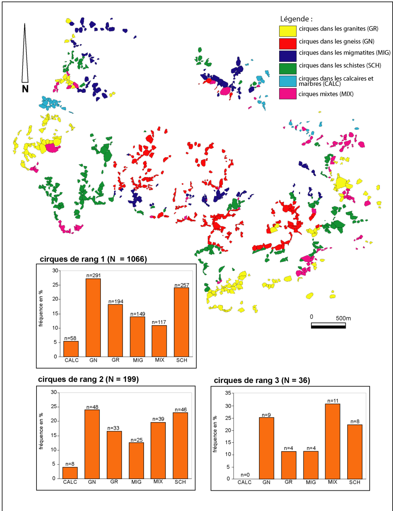
Fig. 8.11 : Lithologie dominante des cirques glaciaires est-pyrénéens
