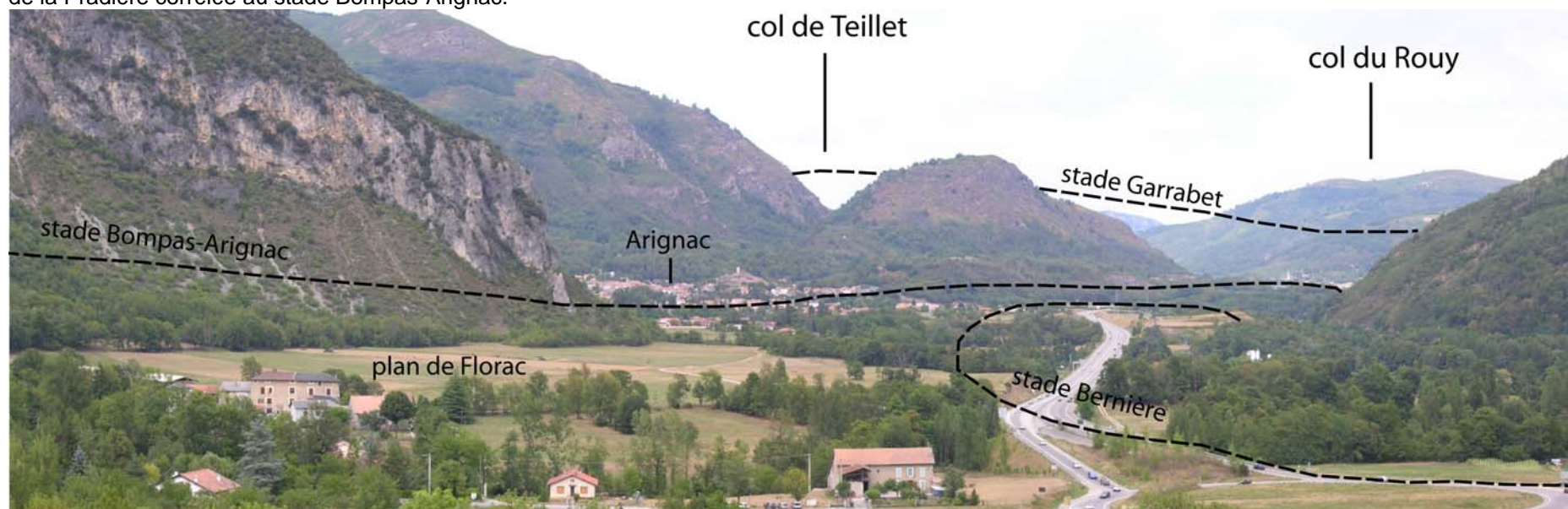
B – Emprise spatiale des stades premiers stades de déglaciation dans le bassin de Tarascon.
