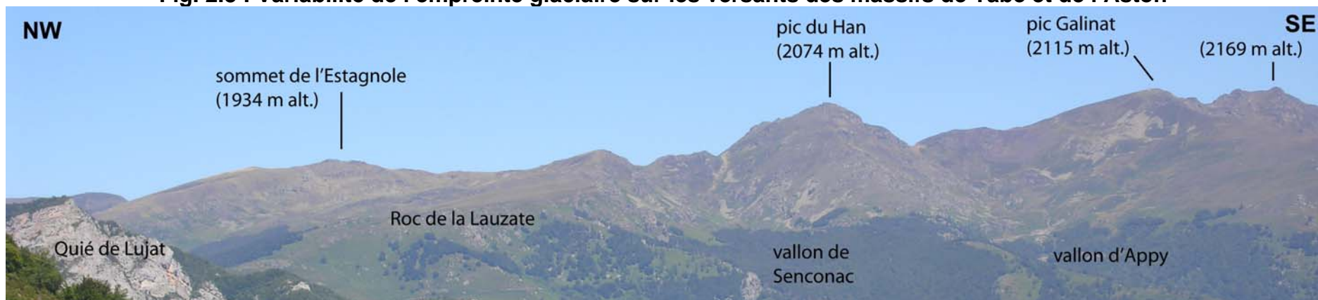
Fig. 2.8 : Variabilité de l’empreinte glaciaire sur les versants des massifs de Tabe et de l’Aston
