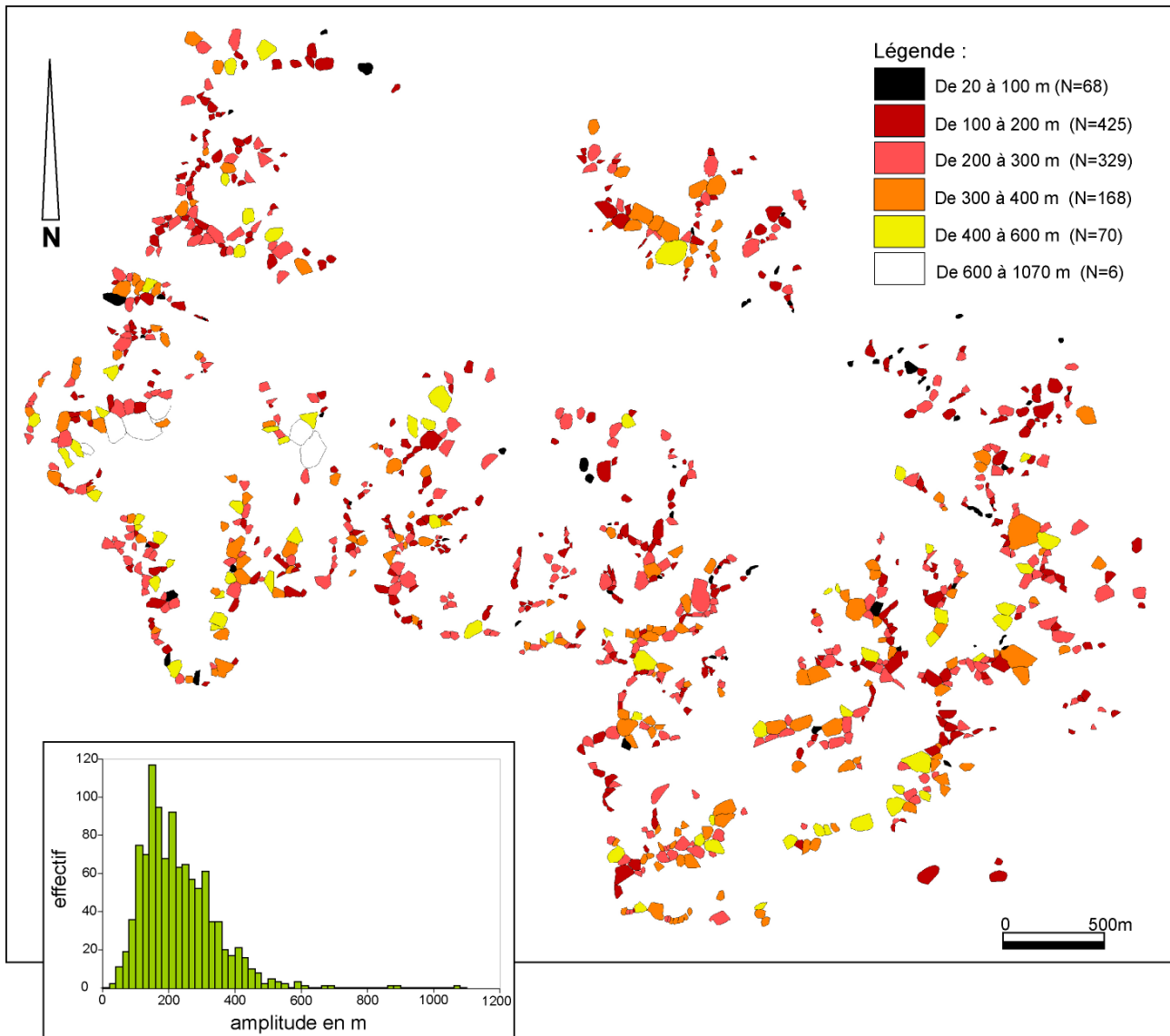
Fig. 8.15 : Cartographie du paramètre amplitude
