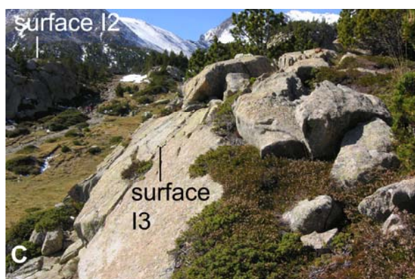
C – Au premier plan, détail de la surface Têt I3 datée par ^{10}\text{Be} à 20 \pm 2,7 ka (Py05-22). En arrière plan, la bosse rocheuse associée aux surfaces Têt I2 (Py04-05), en position sommitale, et Têt I4 (Py05-23), sur la paroi aval du verrou.
