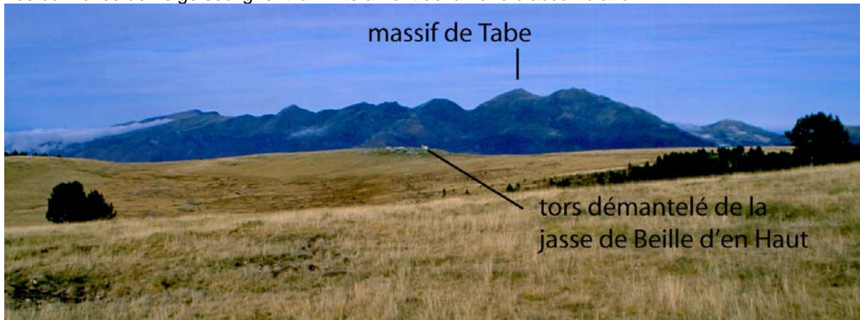
B – Esquisse de cirque situé au niveau de la jasse de Beille d'en Haut. Vue vers le nord.
