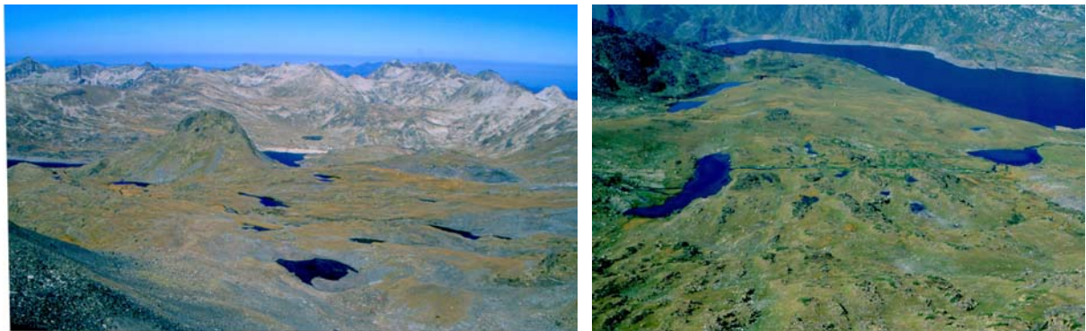
B et C – Le haut bassin du Carol, dépression du Lanoux (Carlit nord)
