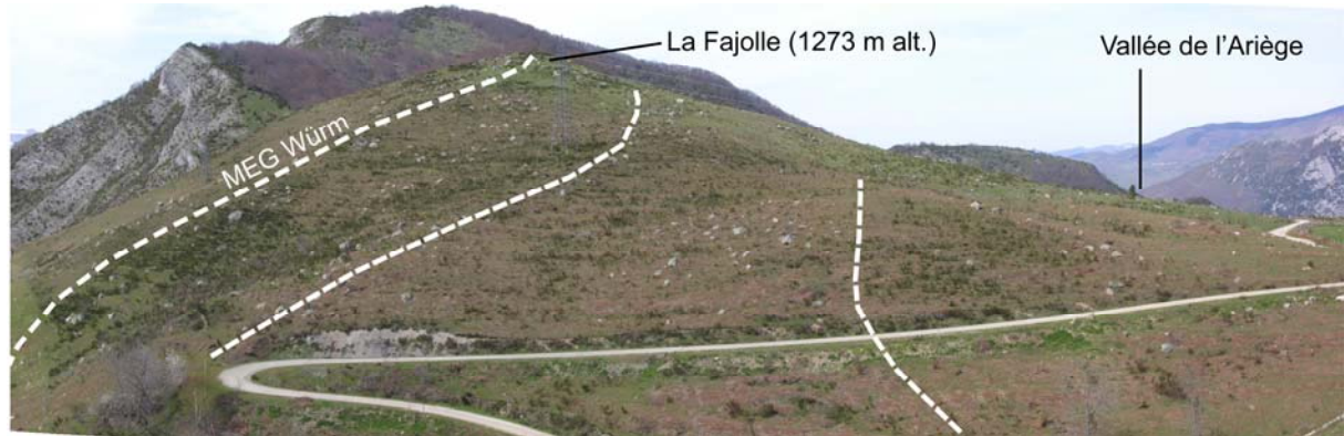
B – Le tracé des moraines indique une difffluence de la glace ariégeoise vers le Vicdessos.
