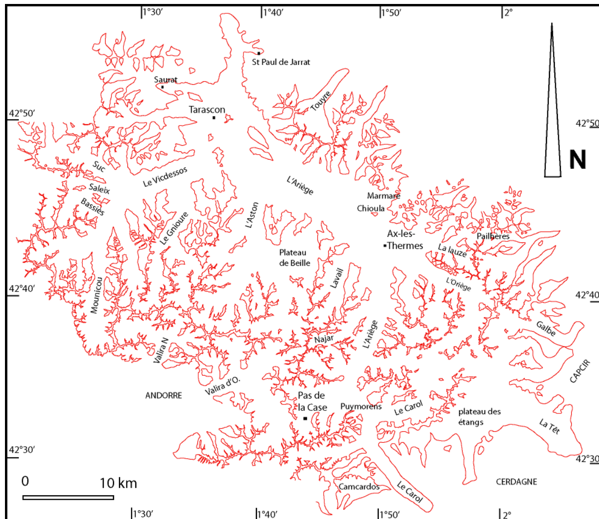
Fig. 5.62 : L'emprise spatiale des paléoenlacements würmiens dans l'est des Pyrénées (d'après Calvet, 2004 et levées personnelles)
