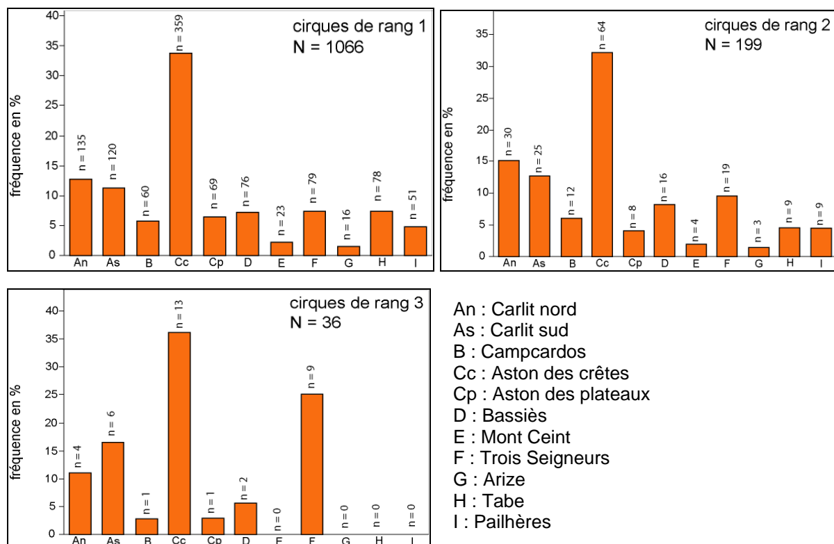
Fig. 8.7 : Fréquences et effectifs des cirques glaciaires est-pyrénéens classés par massifs d'appartenance
