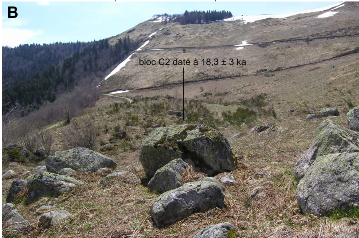
B – Blocs erratique posé sur la moraine MEG Würm de Larcat. Surface datée à 18,3 \pm 3 ka sur le sommet du bloc (C2, Py05-07)
