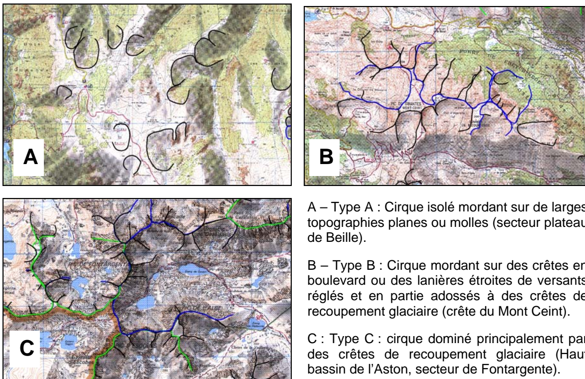
Fig. 8.5 : Les trois modalités du paramètre type de ligne de crête
