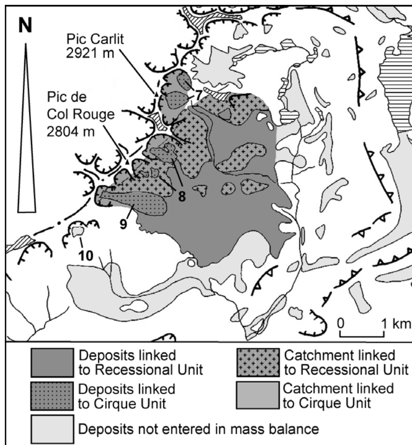
Fig. 7.5 : L'emprise spatiale des dépôts au faciès openwork du secteur Soccarades (Extrait de Delmas et al., 2009, modifié)
