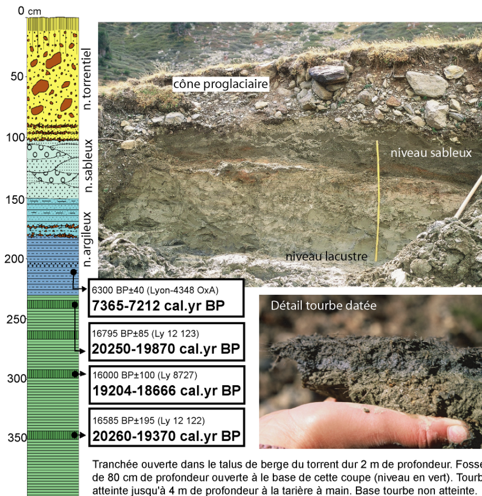
C – La coupe et la position des échantillons datés par 14 C
