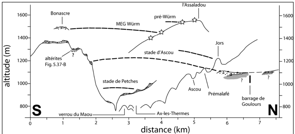
Fig. 5.41 : Würm et pré-Würm dans le bassin d'Ax-les-Thermes
