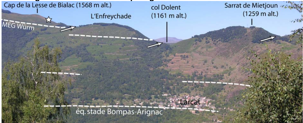
A – Vue depuis la rive droite de la vallée d'Aston. L'étoile blanche localise un jalon morainique pré-würmien (photo C). Les flèches blanches localisent les zones de difffluence.
