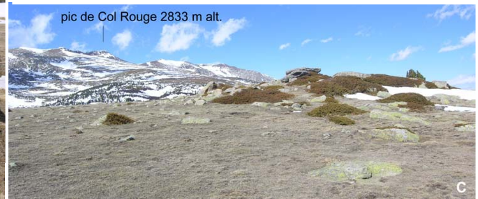
C – Tor démantelé situé en avant du front MEG Würm des Estagnets. Ce tor a probablement été recouvert au cours des cycles glaciaires pré-würmiens mais aucun indice de till n'a permis de le confirmer (idem pour la vasque à encorbellement de la photo B).
