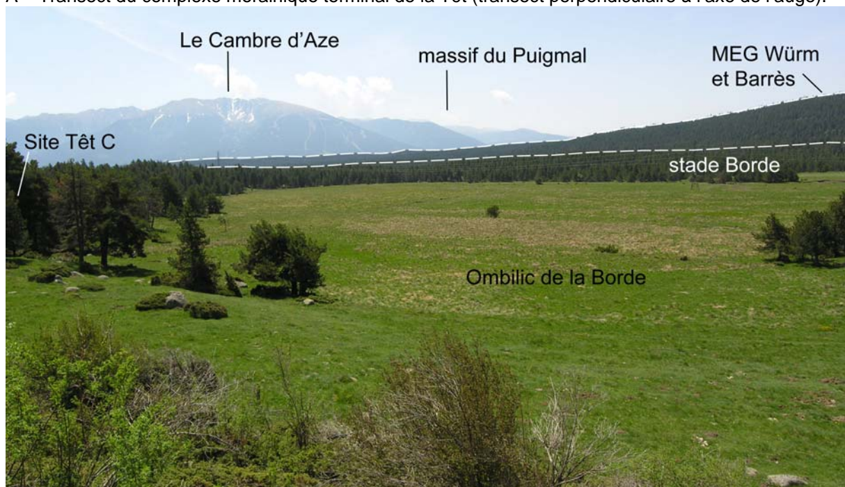
B – L'ombilic de la Borde, vue vers le sud. Noter la position du site d'échantillonnage en vue de datations par le cosmonucléide ^{10}\text{Be} (Site Têt C : trois échantillons sur sommets de blocs erratiques prélevés sur le cordon morainique qui ferme l'ombilic de la Borde). Le site Têt D, non visible sur la photo) correspond à verrou localisé au plancher de l'auge, immédiatement en amont de l'Ombilic.
