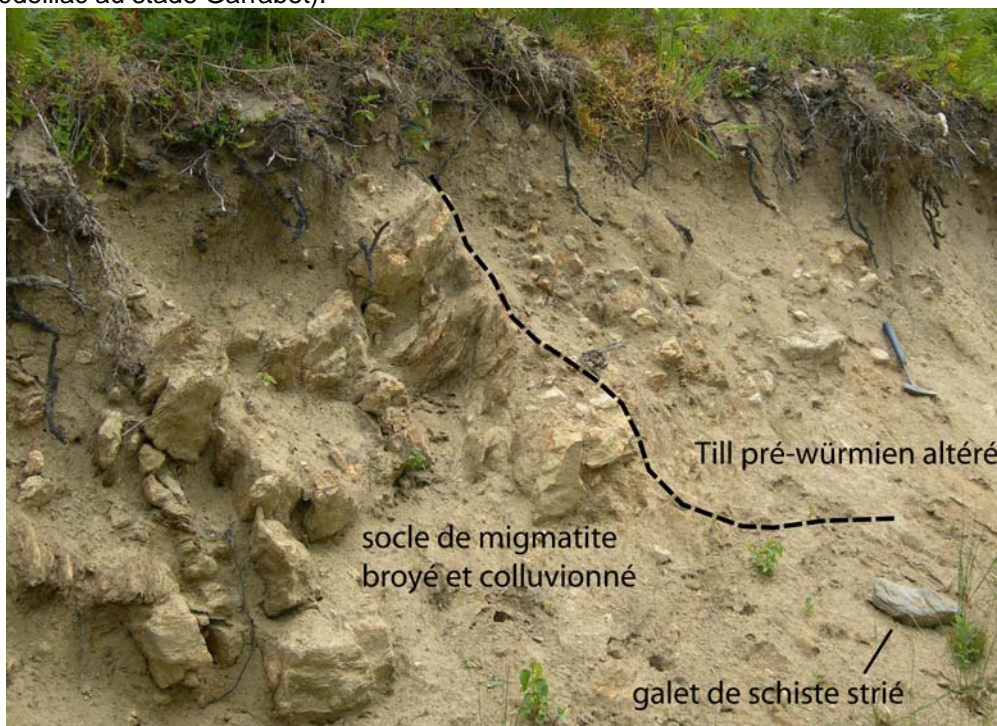
D - Dépôts morainiques pré-würmiens de Coume Jouan
