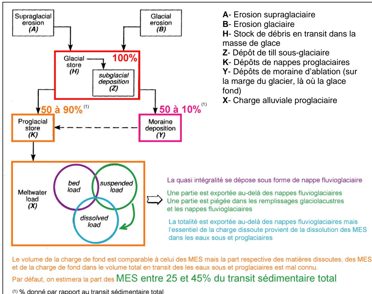
Fig. 7.8 : Part des MES dans le transfert sédimentaire glaciofluvial (D'après Warburton et al., 1993)
