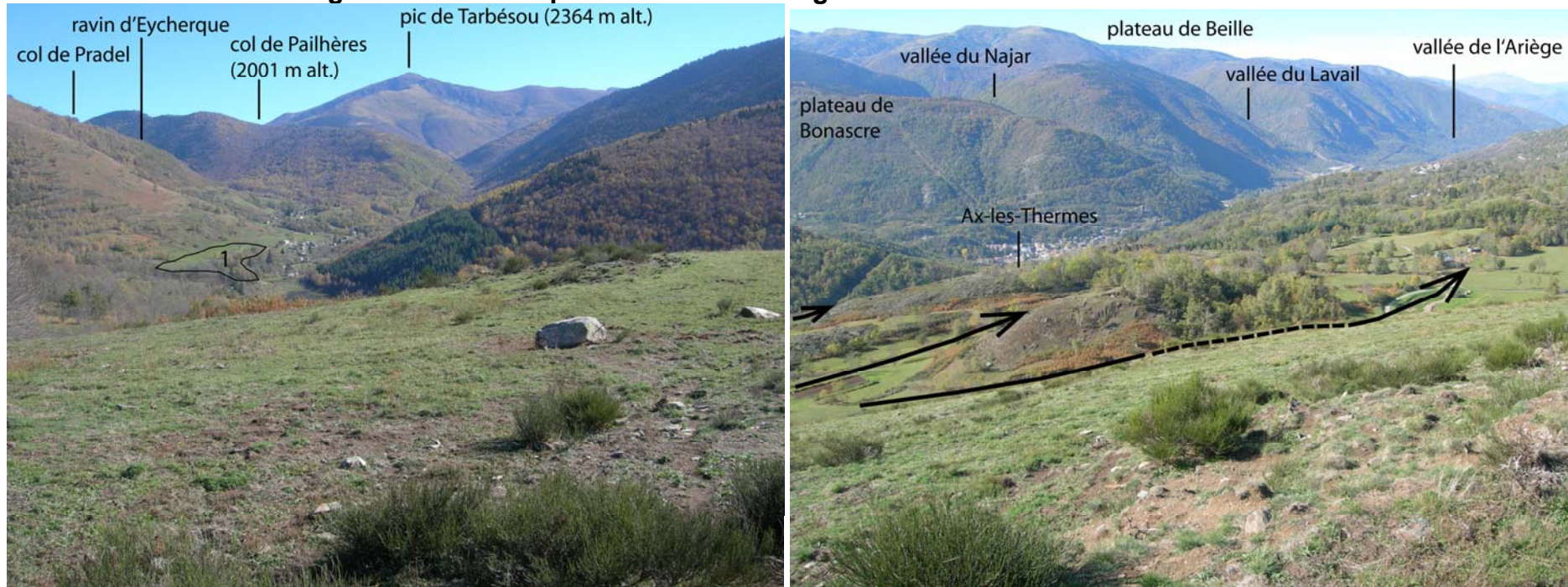
Fig. 5.43 : Würm et pré-Würm sur la marge nord du bassin d’Ax-les-Thermes
