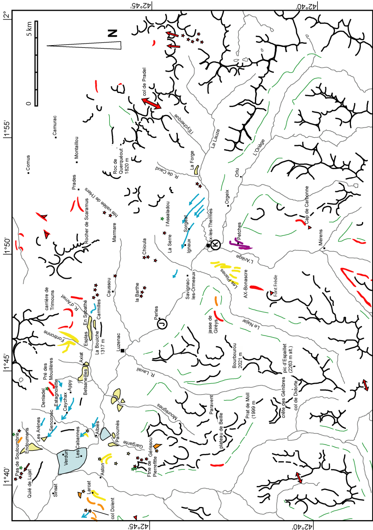
Fig. 5.29 : Carte géomorphologique des formes et dépôts glaciaires : Haute vallée de l'Ariège (Légende p. 157)
