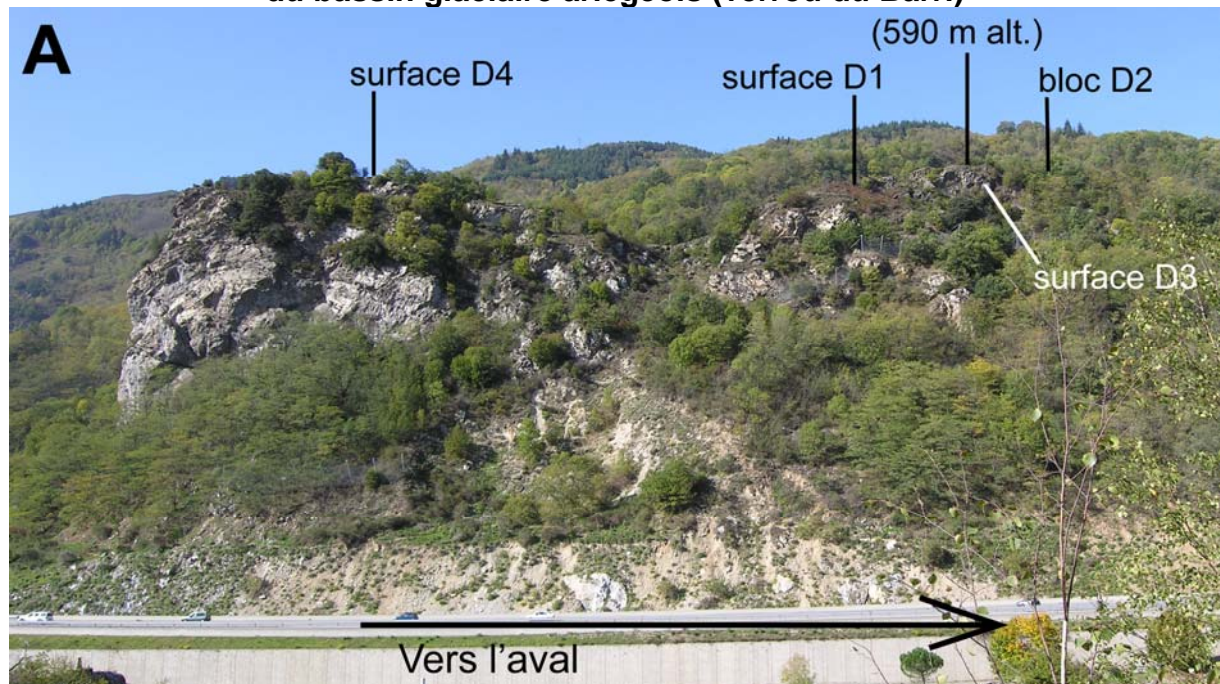
Fig. 6.13 : Les surfaces rocheuses échantillonnées sur le site D du bassin glaciaire ariégeois (verrou du Barri)
