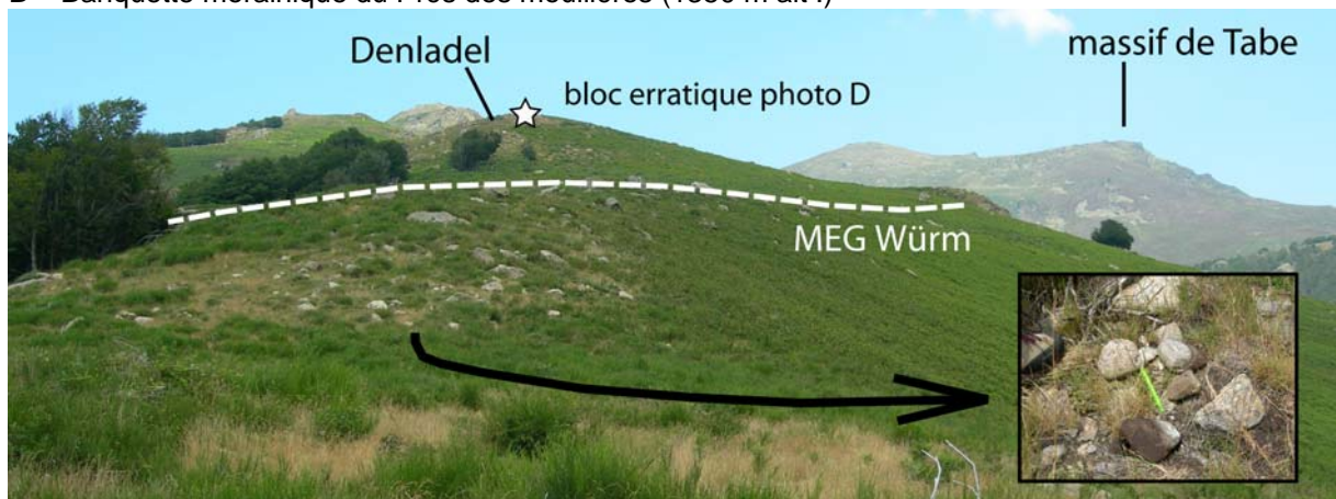
C – Cordon morainique latéral situé vers 1450 m d'altitude et associé au MEG Würm.
