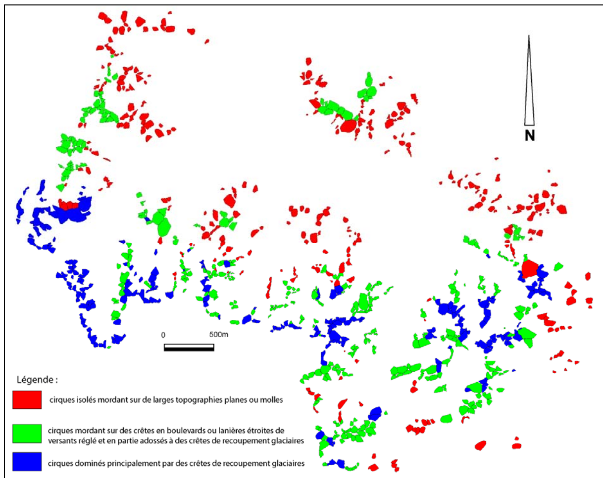
Fig. 8.9 : Carte des types de crêtes auxquelles sont adossés les cirques glaciaires est-pyrénéens
