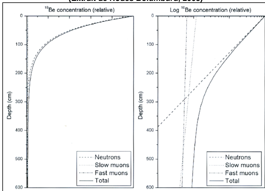
Fig. 4.2 : Variation du taux de production en fonction de la profondeur (Extrait de Rodas Bolumburu, 2008)
