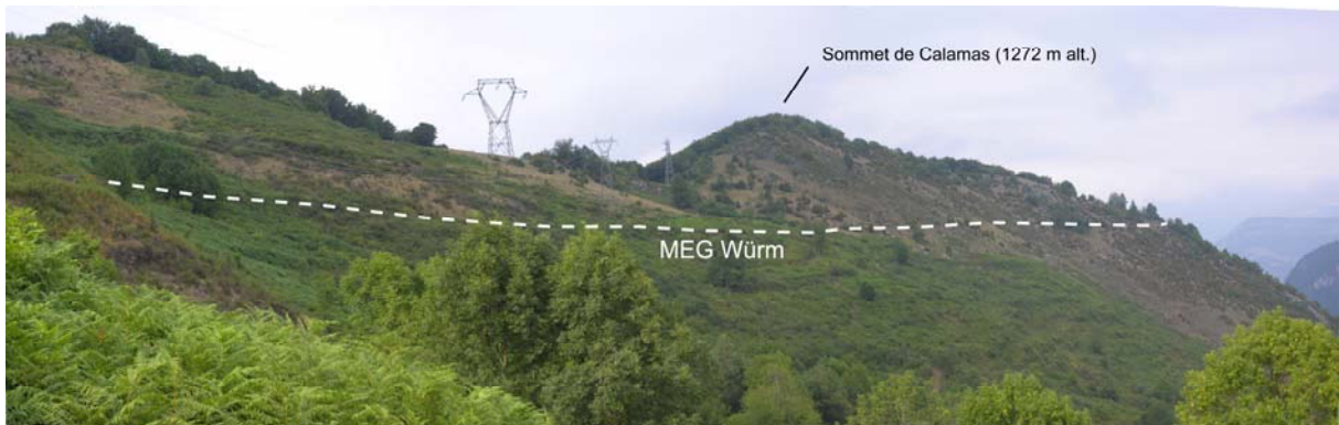
A – La banquette morainique de Lapège-Pladétis.
