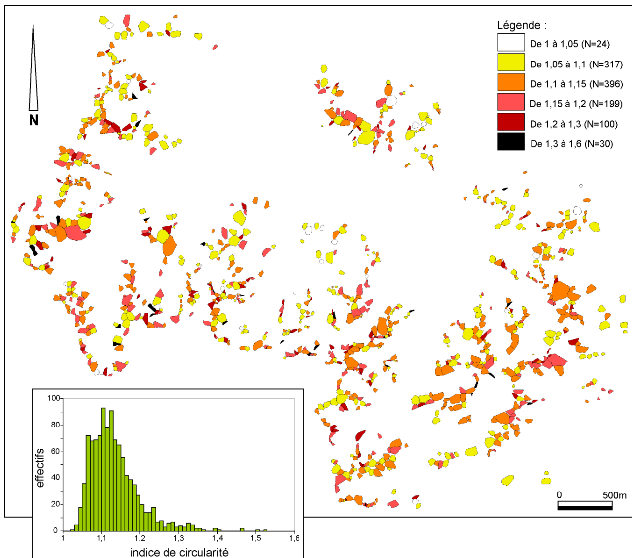
Tabl. 8.14 : Analyse descriptive du paramètre indice de circularité
