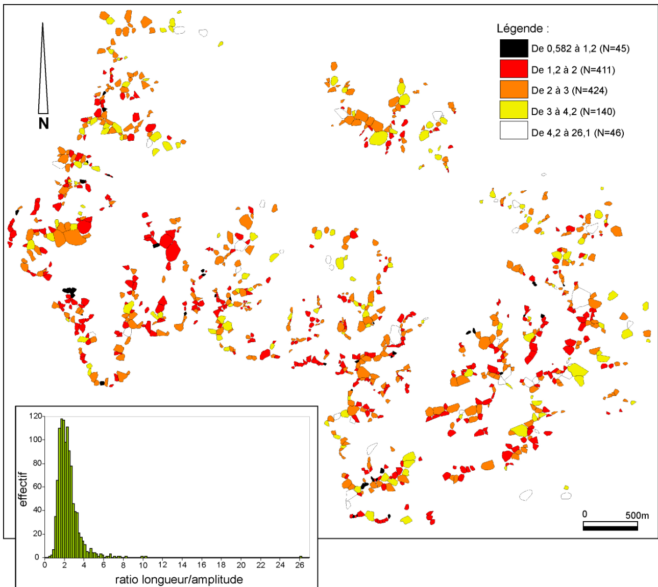
Fig. 8.19 : Cartographie du paramètre ratio longueur-amplitude
