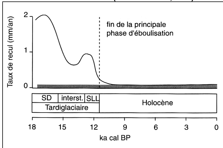
Fig. 1.16 : Evolution du taux de recul des parois rocheuses dans le nord de l'Écosse (Extrait de Hétu, 2004)
