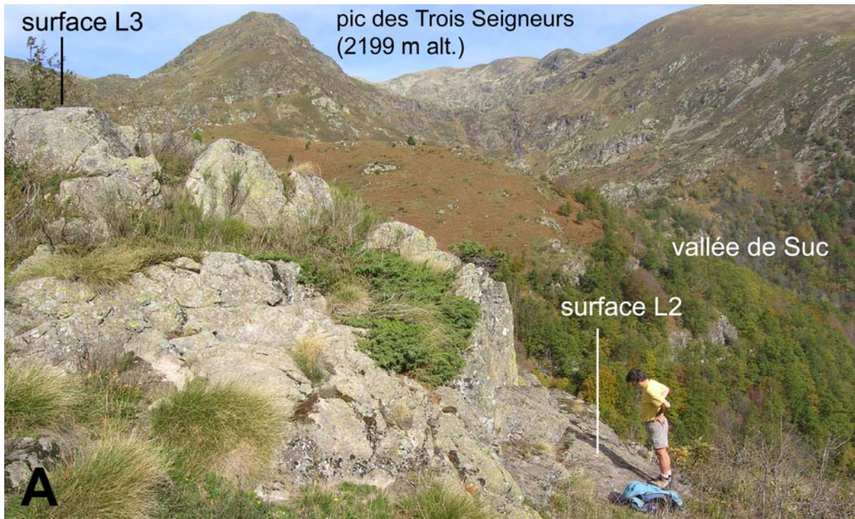
A - Position des échantillons prélevés sur le verrou de Freychinèdes (site L). Noter la position de ce verrou, au débouché des cirques du Pic des Trois Seigneurs La surface polie associée à une trace d'écaillage (L2, Py06-16) est datée à 14 \pm 0,7 ka. La surface polie située sur le sommet de la bosse rocheuse (L3, Py06-17) est datée à 14,4 \pm 1,1 ka. Une autre surface polie, non visible sur la photo, est datée à 16,7 \pm 2,3 ka (L1, Py05-16) et à 16,9 \pm 3,3 ka (L1bis, Py05-16HF4).
