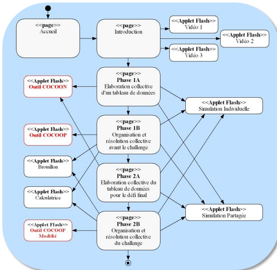
Figure 35 : Diagramme global UML simplifié de la navigation de l'apprenant dans le système
