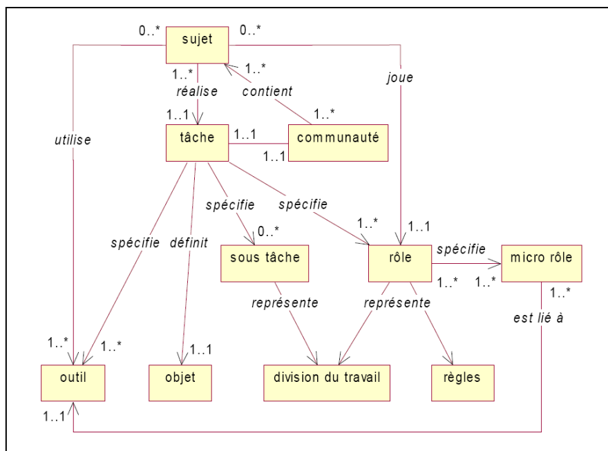
Figure 4 : Modèle conceptuel d'une activité dans DARE [Bourguin 00]
