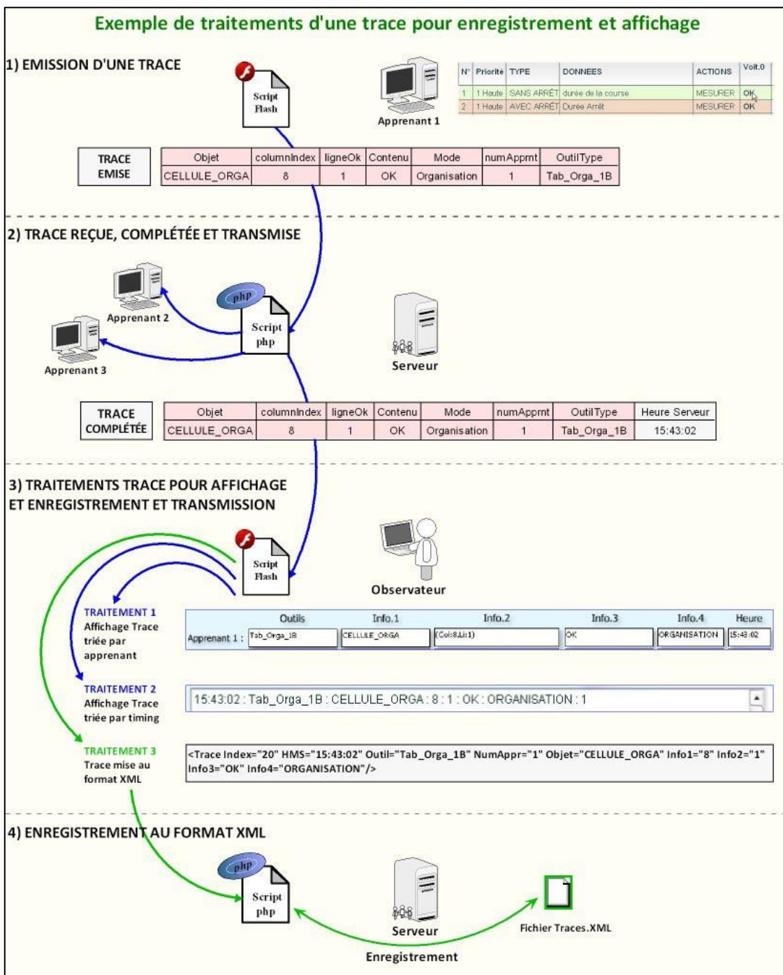
Figure 83 : Exemple de gestion d'une trace
