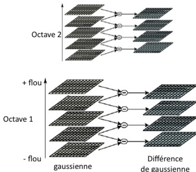
FIGURE 2.6 – Application de cinq filtres gaussiens sur une image et les quatre différences de gaussiennes créées sur deux octaves.
