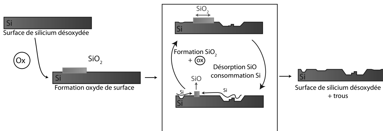
FIGURE C.6 – Mécanisme de la formation des trous par diffusion de surface du silicium pour la désorption de SiO.
