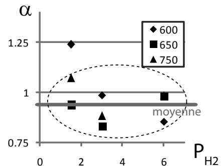
FIGURE 2.18 – Valeurs mesurées et dispersion du coefficients \alpha , v \sim (P_{SiH_4})^\alpha .
