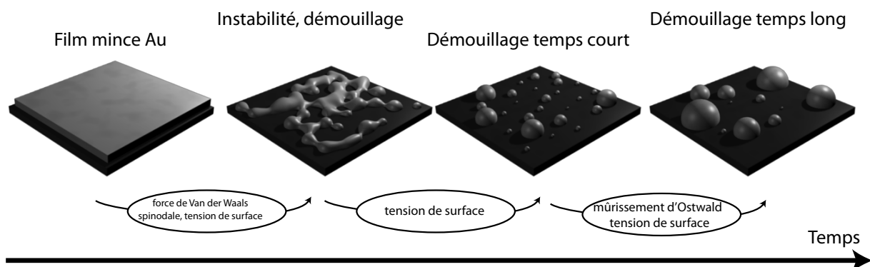
FIGURE 3.12 – Etapes principales du processus de démouillage
