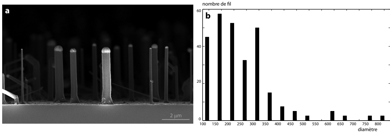
FIGURE 3.11 – [a] Image SEM d'un échantillon de nanofils obtenu à partir du démouillage d'une couche d'or (2nm) sur Si[111]. [b] Histogramme de la distribution des fils selon leur diamètre. (Recuit-démouillage, 850°C, 10 min, 20 mbar H 2 ; croissance fils 650°C, 20 sccm SiH 4 , 8 min).
