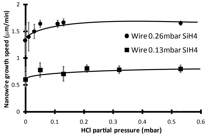
FIGURE 4.9 – Vitesse de croissance de nanofils, obtenus à partir de colloïdes d’or de 200nm de diamètre, en fonction de la pression partielle en fonction du flux de HCl introduit dans le réacteur (650°C, SiH 4 25 sccm ou 50 sccm, HCl variable, H 2 3700 sccm, 20 mbar, 15 min).
