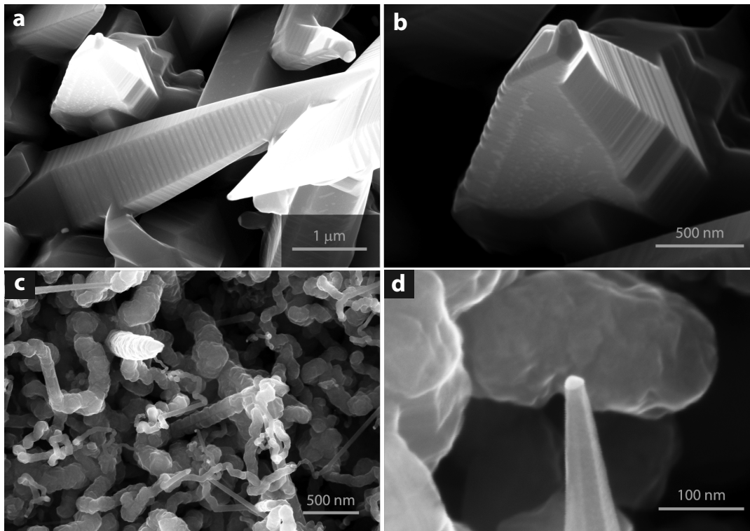
FIGURE 3.53 – Image SEM de nanostructures de Si réalisées à partir de PtSi déposé sur Si[100]. [a] et [b] Croissance à haute température (850°C, SiH 4 20 sccm, 40 min). [c] et [d] Croissance basse température (650°C, SiH 4 20 sccm, 40 min).
