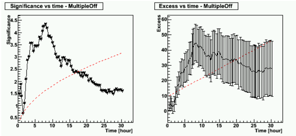
FIG. 5.19: Variation de la significativité et du nombre de gamma en provenance de J1854 au cours du temps sur l'ensemble des périodes d'observations.
