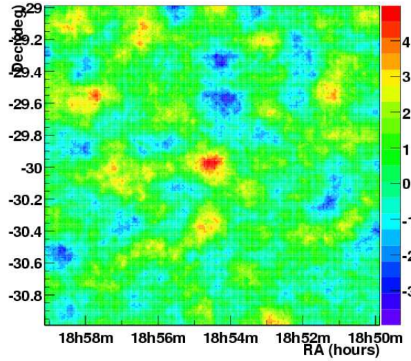
FIG. 5.10: Carte de significance de la région du ciel centrée sur le faible signal J1854 pour l'analyse X_{\text{eff}} à 200 pe.
