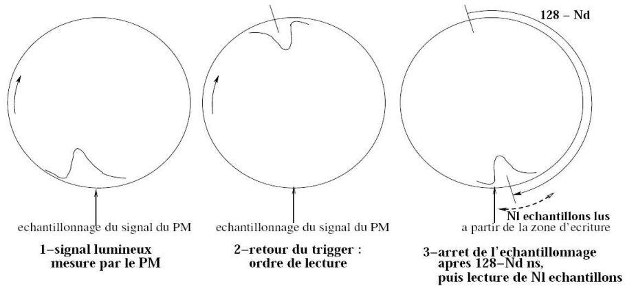
FIG. 2.10: Lecture d'une voie d'une mémoire analogique et définitions des paramètres N_d et N_L .
