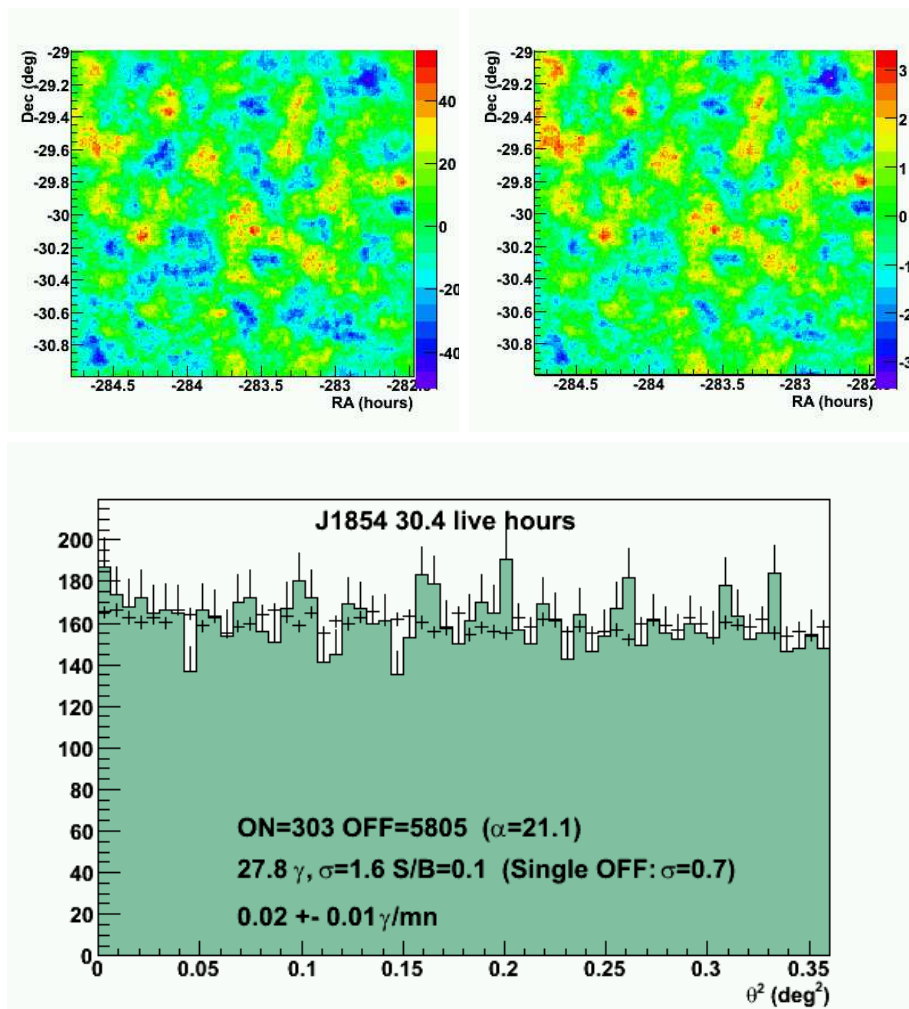
FIG. 5.18: Haut :Cartes d'excès ( gauche ) et de significativité ( droite ) d'une région de ciel de 2.5^\circ \times 2.5^\circ centrée sur la position de J1854. Bas : Distribution radiale des événements par rapport à la position de référence de J1854. Les valeurs données correspondent à une coupure angulaire de 0.01^\circ autour de la position de J1854. Les résultats présentés correspondent à une analyse X_{\text{eff}} avec une coupure en charge totale de l'image de 200 pe pour l'année 2008.
