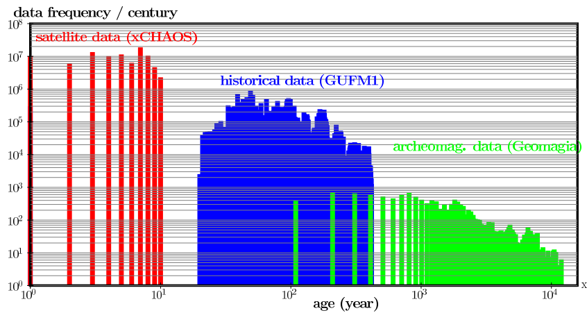
FIG. 2.5 – Nombre de données par siècle, en fonction de l'âge des données (en années, les époques récentes sont donc 10^0 ). Les différentes couleurs correspondent aux données satellitaires (rouge, nombre de données utilisées pour le modèle de champ magnétique xCHAOS (Olsen et Mandeia 2008)), aux données historiques (bleu, nombre de données utilisées pour le modèle de champ magnétique gufm (Jackson et al. 2000)) et aux données archéomagnétiques (vert, pour la base de données Geomagia Korhonen et al. (2008)). L'obtention de modèles de champ est décrite dans la section 2.1.3. Communication de N. Gillet.
