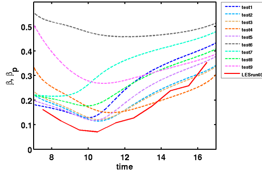
FIG. 7.6 – Evolution temporelle des de \beta paramétrisé par le flux de surface, la prise en compte de l'évolution de l'énergie cinétique turbulente et le cisaillement de vent en Z_i pour les simulations 1D avec des conditions initiales de vent différentes. Le \beta obtenu dans la LES (cf. eq. 3.1) est représenté en rouge.
