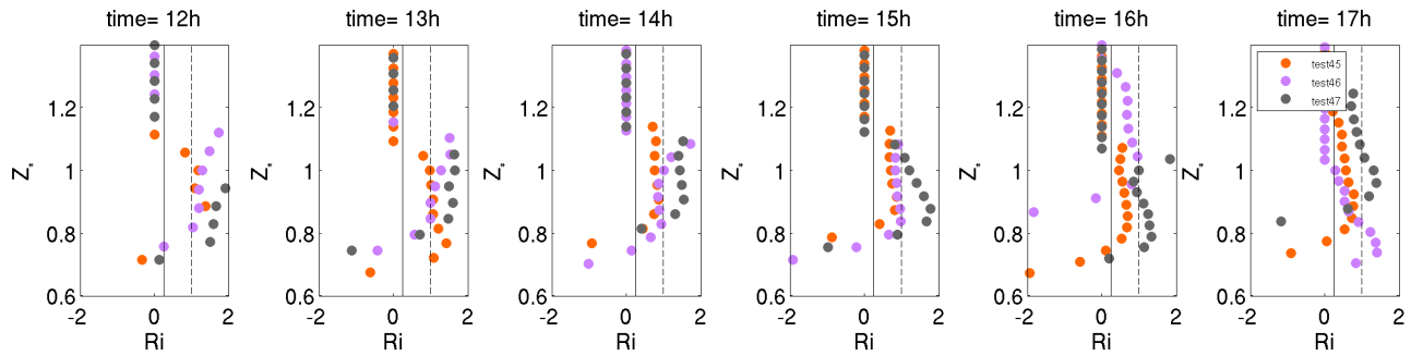
FIG. 6.41 – Evolution temporelle du profil du nombre de Richardson flux pour les tests 45, 46 et 47 (voir figure 6.21). Le trait noir correspond à Ri_{critique} = 0.25 qui délimite les conditions instables et les conditions stables.
