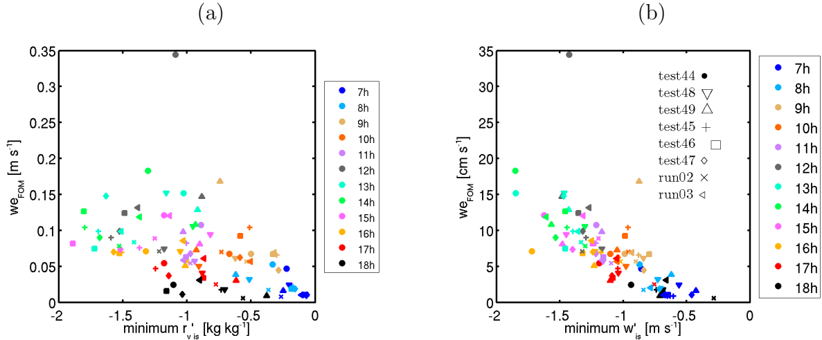
FIG. 6.36 – Comparaison entre (a) le minimum de fluctuation de r_v et la vitesse d'entraînement dans les intrusions sèches, (b) le minimum de fluctuation de w et la vitesse d'entraînement dans les intrusions sèches
