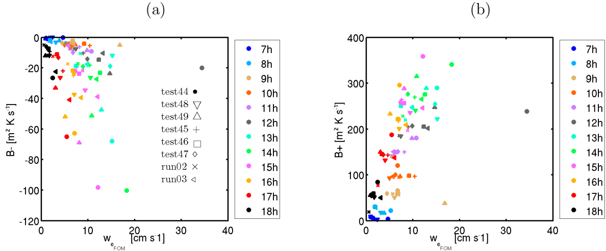
FIG. 6.27 – Comparaison entre (a) l'aire négative du flux de flottabilité et la vitesse d'entraînement (b) l'aire positive du flux de flottabilité et la vitesse d'entraînement calculée à partir d'un modèle d'ordre 1 pour les 8 cas de l'étude et pour chaque heure.
