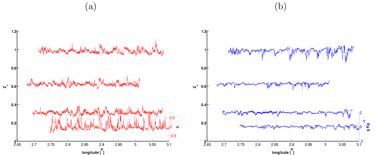
FIG. 5.1 – Représentation des mesures haute fréquence obtenues par l'ATR-42 dans un plan vertical pour la journée du 6 juin 2006 (vol 18) de (a) la température potentielle et (b) le rapport de mélange pour les paliers dans la CLA. L'axe de gauche indique le niveau de chaque palier par rapport à Z_i et l'axe de droite indique l'échelle des fluctuations.
