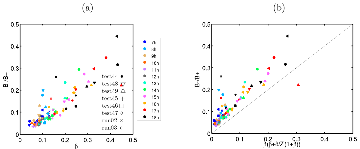
FIG. 6.25 – (a) Comparaison entre le rapport des aires négatives et positives du flux de flottabilité et le taux d'entraînement, (b) comparaison entre le rapport des aires négatives et positives du flux de flottabilité et le calcul par la méthode des aires appliquée à un modèle d'ordre 1 (cf. eq. 3.37) pour les 8 cas de l'étude.
