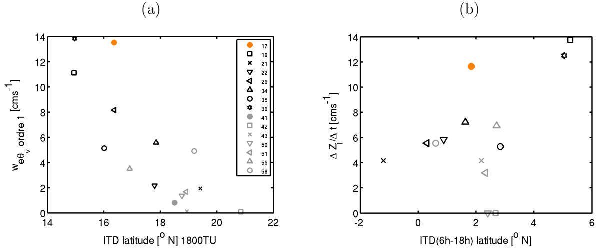
FIG. 5.10 – Comparaison entre (a) la vitesse d’entraînement calculée avec la température potentielle virtuelle à partir de la paramétrisation d’ordre 1 et la position de l’ITD à 18H00 à la longitude de Niamey; (b) Taux d’accroissement de la CLA en fonction de la variation diurne de la position de l’ITD entre 6h et 18h. Les symboles gris représentent les vols de la période de mousson active et les symboles noirs les vols de la période pré-onset. Le symbole orange correspond au 5 juin.
