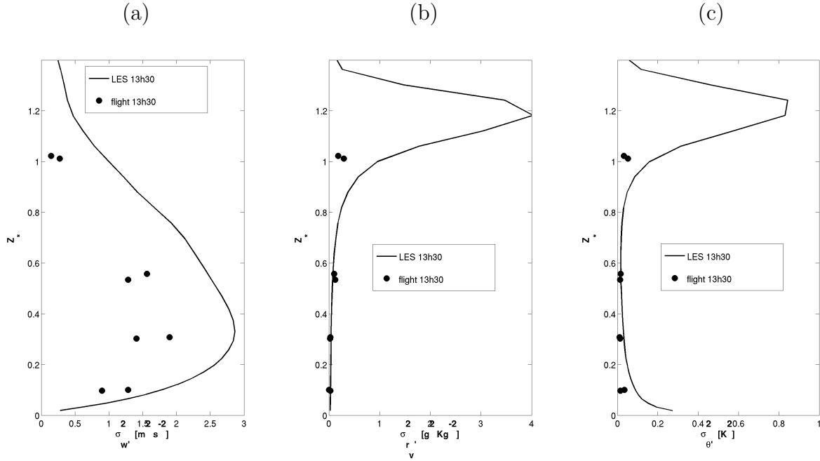
FIG. 6.13 – Profils verticaux de la variance simulée (trait plein) et observée (points) (a) de la vitesse verticale, (b) du rapport de mélange et (c) de la température potentielle le 5 juin 2006. Z_* est déterminé avec Z_i observé pour les données de l'avion et avec Z_i de la LES pour les données de la simulation.
