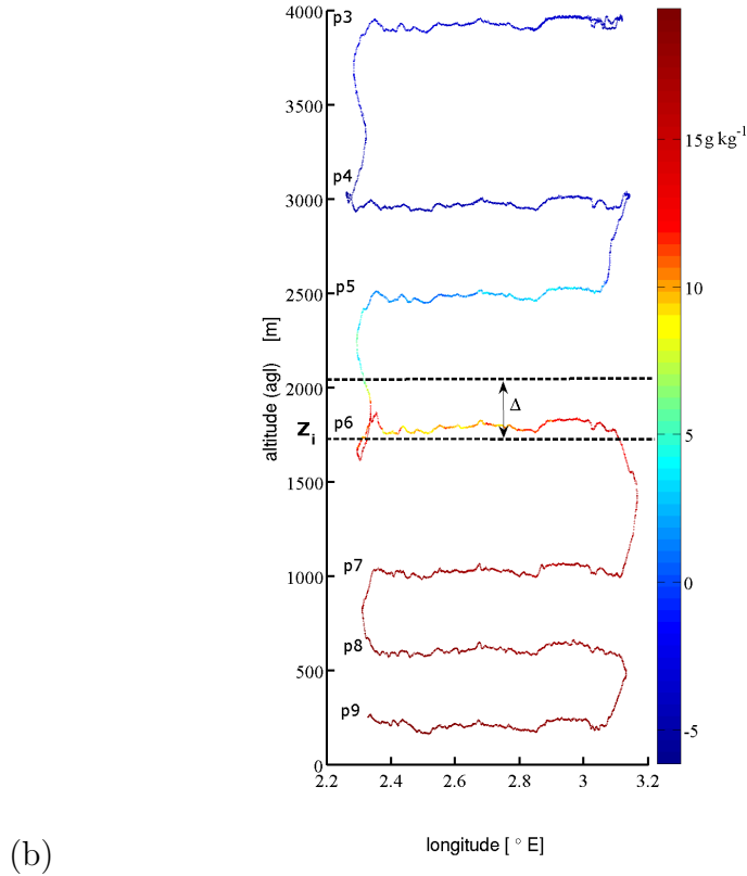
FIG. 4.5 – (a) Trace horizontale de la trajectoire des 15 vols de cette étude. (b) Exemple de mesure du rapport de mélange lors du plan est-ouest du vol 17 décrivant 3 paliers dans la CLA, 1 au niveau de Z_i et 3 dans la troposphère libre.
