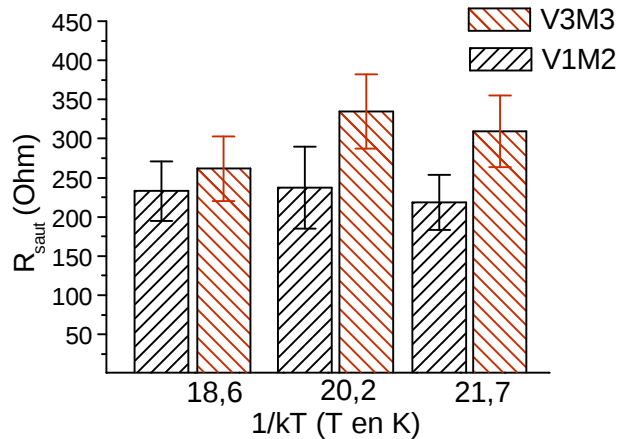
Figure IV-7 : Evolution de R_{\text{saut}} avec la température
