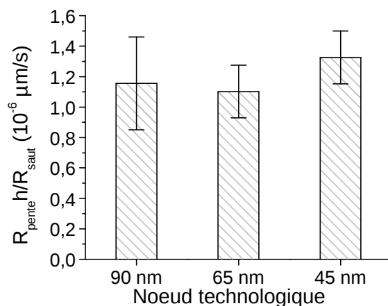
Figure IV-5 : Comparaison des vitesses de dégradation de différents nœuds technologiques
