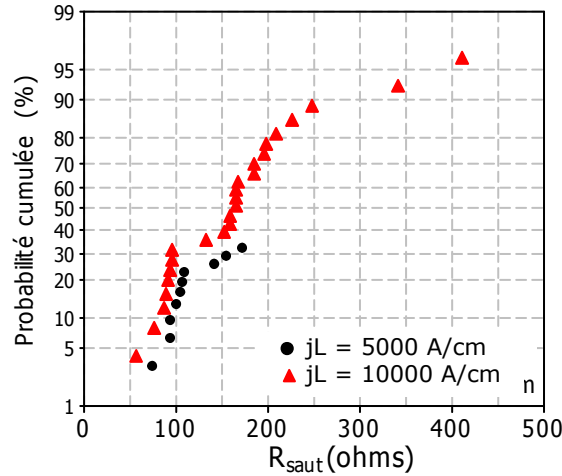
Figure V-13 : Comparaison des distributions de R_{saut} entre 5000 et 10000 A/cm pour L = 25 \mu m
