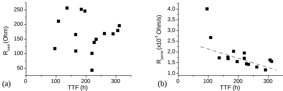
Figure IV-19 : Evolution de (a) R_{\text{saut}} et (b) R_{\text{pente}} en fonction du TTF
