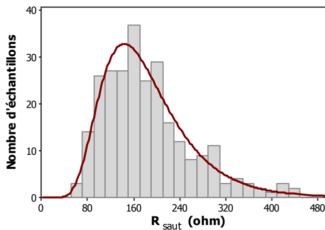
Figure III-23 : Histogramme des R_{\text{saut}} ajusté par une distribution lognormale
