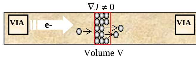
Figure II-10 : Dégradation induite par une discontinuité de flux
