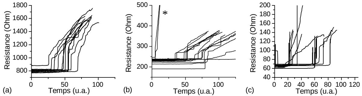
Figure IV-1 : Evolution de la résistance des lignes de (a) 90 nm, (b) 300 nm et (c) 1 \mu m de large
