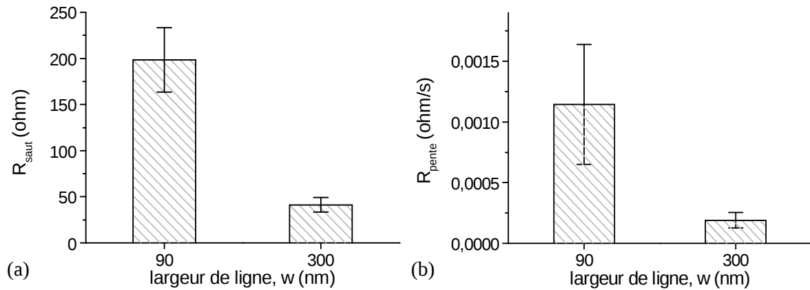
Figure IV-3 : Evolution des valeurs brutes de (a) R_{\text{saut}} et (b) R_{\text{pente}} en fonction de la largeur
