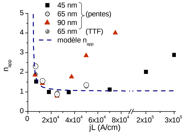
Figure V-3 : Evolution du n_{app} en fonction du produit jL
