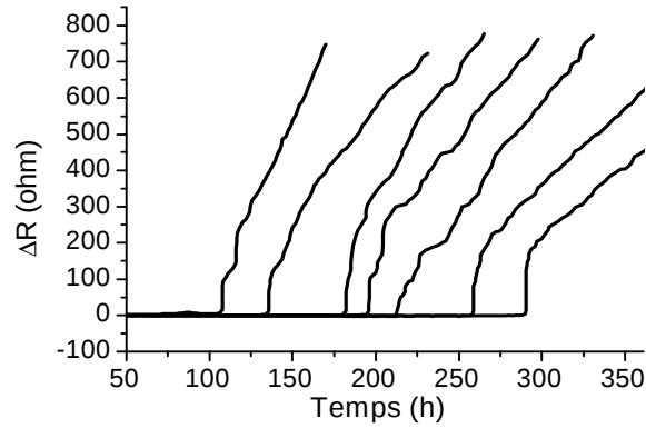
Figure IV-18 : Courbes R(t) illustrant la corrélation R_{\text{pente}} / \text{TTF}
