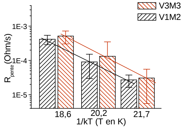
Figure IV-8 : Evolution de R_{pente} en fonction de 1/kT
