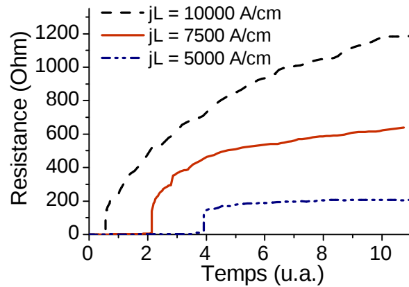
Figure V-24 : Evolution de la résistance d'une ligne de 50 \mu m pour jL \leq 10000 A/cm
