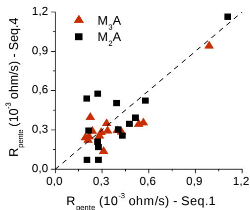
Figure IV-11 : Reproductibilité de la mesure de R_{pente} par échantillons à T = 260^{\circ}\text{C}
