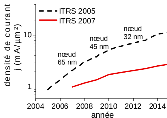
Figure I-5 : Prévision de l'ITRS des densités de courant maximales dans les interconnexions à 105°C
