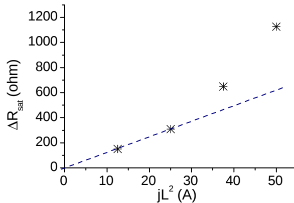
Figure V-25 : Evolution de \Delta R_{sat} en fonction de jL^2
