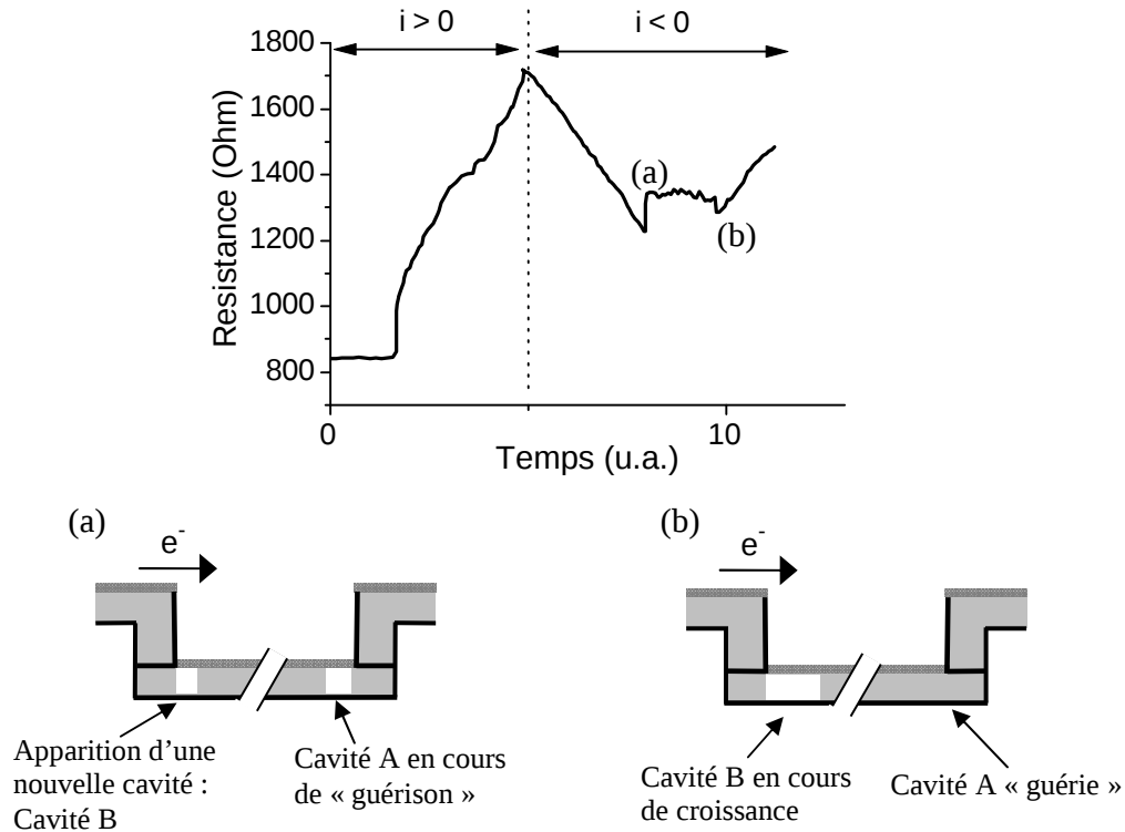
Figure V-26 : Courbe R(t) d'un test bidirectionnel
