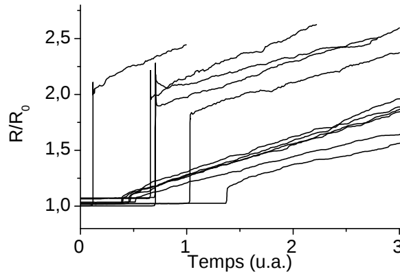
Figure IV-23 : Evolution relative de la résistance
