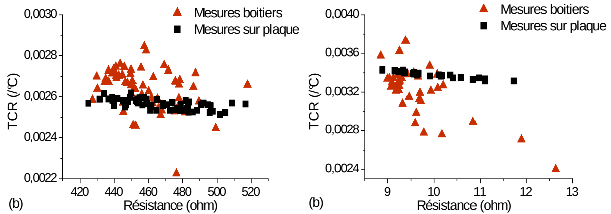
Figure III-13 : Comparaison des TCR mesurés en boitiers et sur plaque (a) w = 90 \text{ nm} , (b) w = 3 \mu\text{m}
