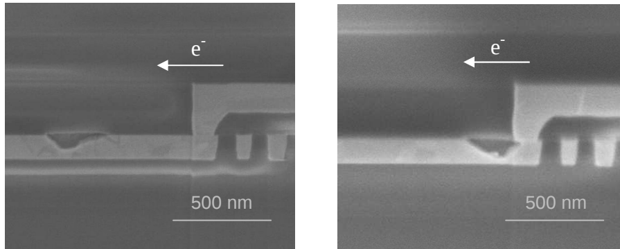
Figure V-14 : Observation FIB/MEB des lignes de 25 \mu m non défailles pour jL = 5000 A/cm
