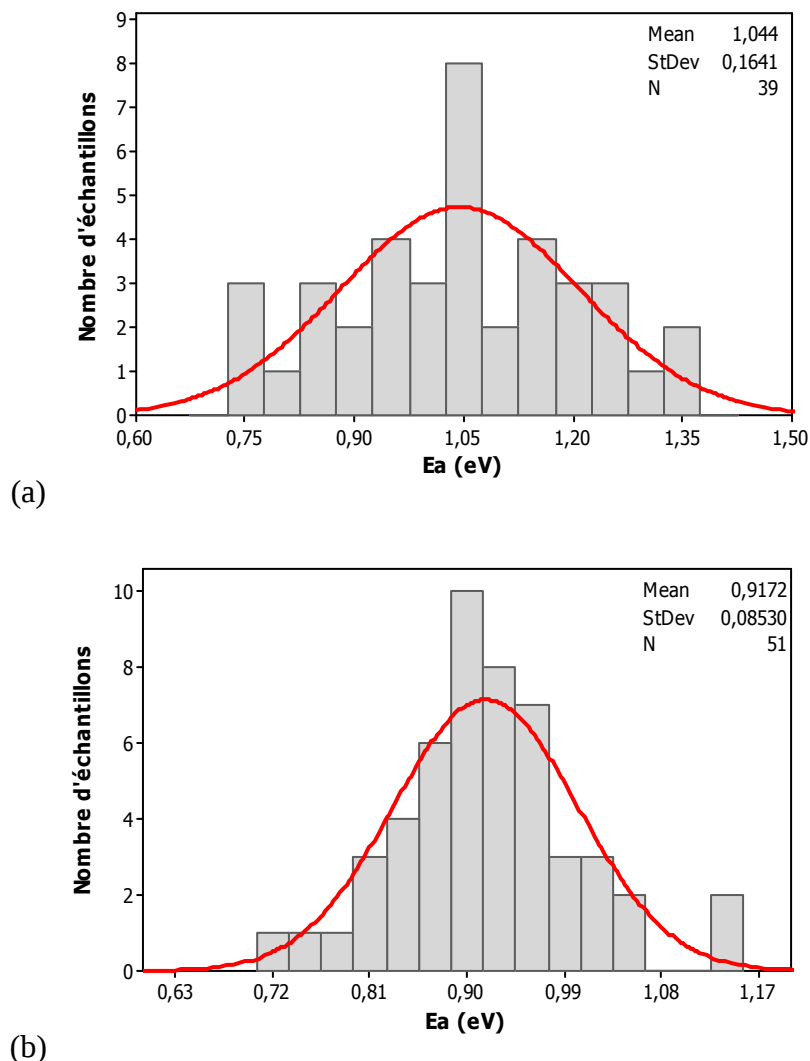
Figure IV-13 : Histogrammes des valeurs individuelles de E_a pour (a) la structure V1M2 et, (b) la structure V3M3
