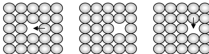
Figure II-1 : Diffusion lacunaire
