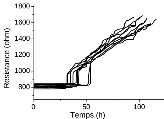
Figure IV-21 : Courbes R(t) illustrant la corrélation R_{\text{saut}} / \text{TTF}
