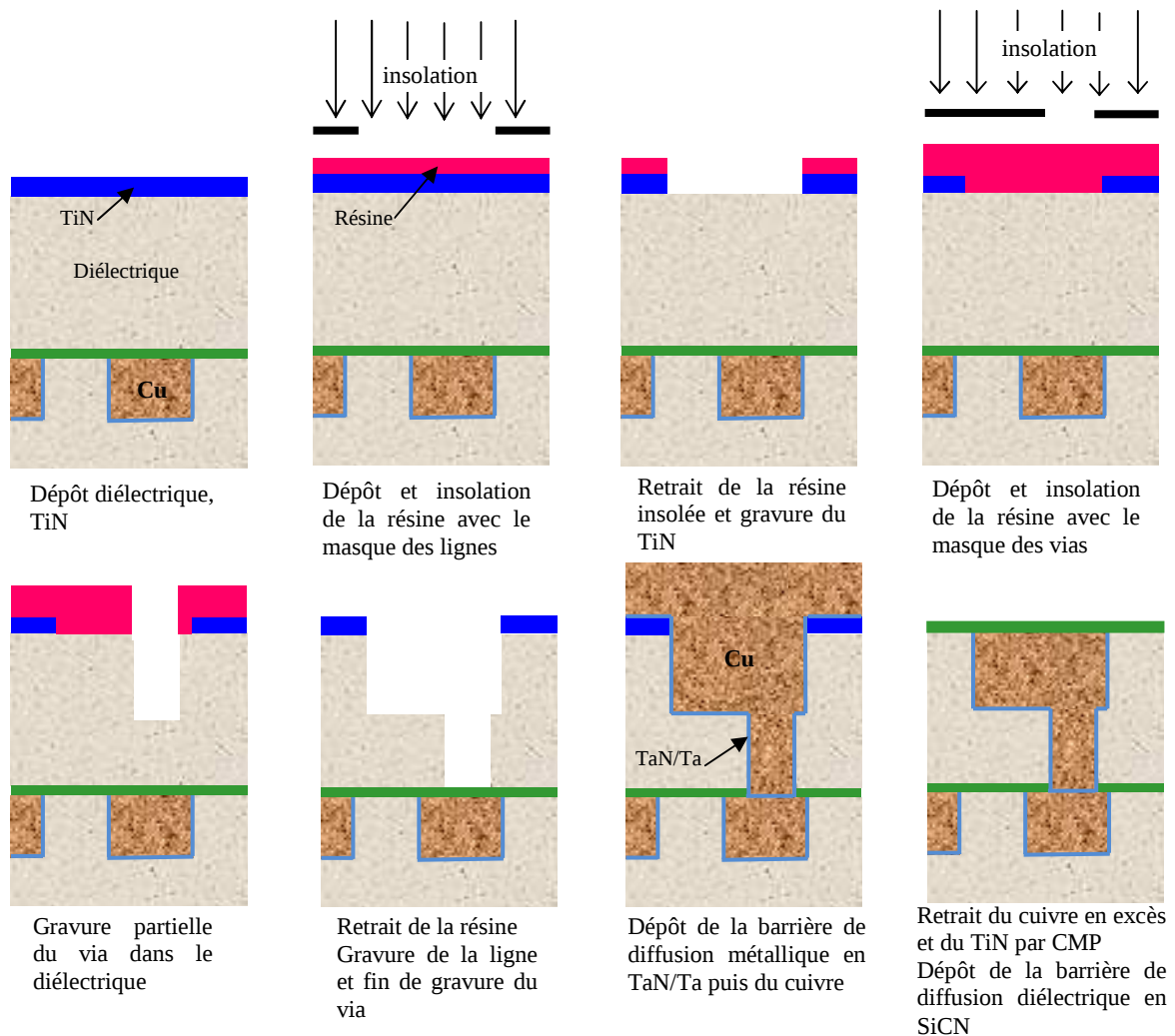
Figure I-2 : Description des étapes de fabrication du procédé double damascène
