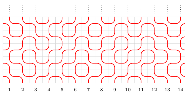
FIG. F.2 – Un exemple d’une configuration du CPL, ici avec n = 7 . Chaque ligne est composée de 14 plaquettes qui peuvent être de deux types. Les bords de gauche et de droite sont identifiés pour former un cylindre. À chaque boucle fermée on donne le poids \tau .
