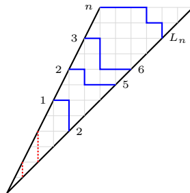
FIG. F.5 – La somme \sum_{\alpha} \psi_{(p)\alpha} compte les NILP avec p chemins fixés verticalement, comme le montre cette figure.
