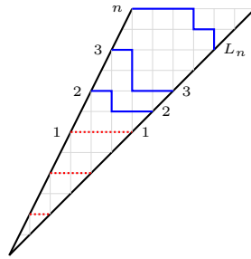
FIG. F.4 – La somme \sum_{\pi} \psi_{(\pi)_p} compte le nombre de NILP avec n + p chemins présentés dans cette figure où les p + 1 premiers chemins sont fixés horizontalement.
