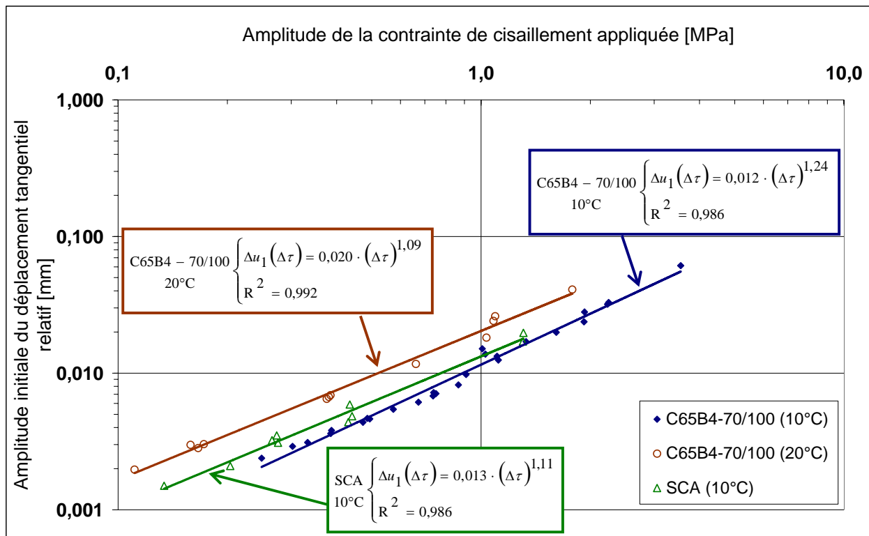
Figure V.1-1. Amplitude initiale du déplacement relatif en fonction de la sollicitation appliquée
