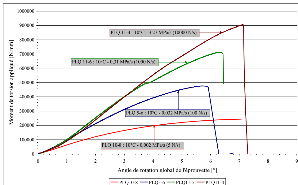
Figure IV.4-4. Moment de torsion en fonction de l'angle de rotation de l'éprouvette (essais à 10°C)
