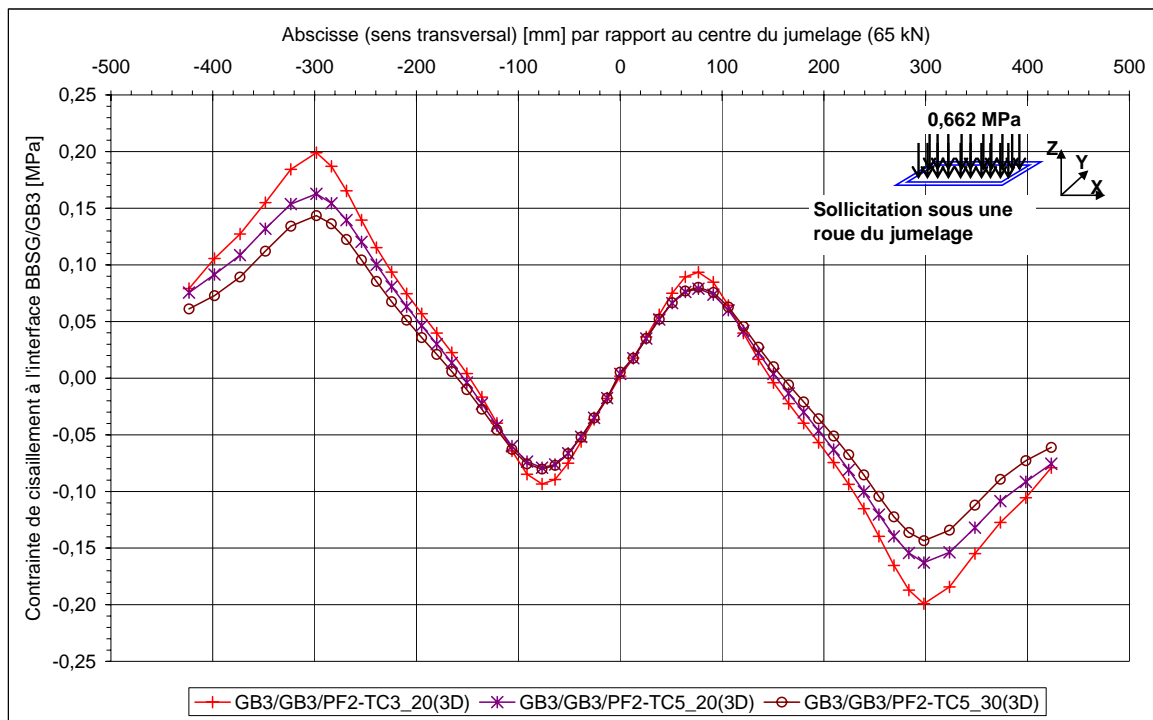
Figure VI.3-12. Valeurs de contrainte de cisaillement à l'interface BBSG/GB3 ( interfaces collées telles que K_{S1} = 81 \text{ MPa/mm} , sollicitation normale verticale de 0,662 MPa )
