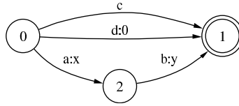
FIG. 1.6 – Un transducteur d'états finis
