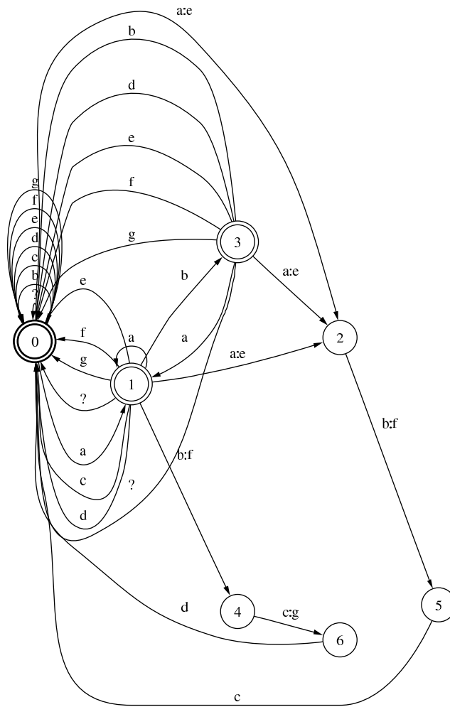
FIG. 5.6 – Le transducteur de règles R
