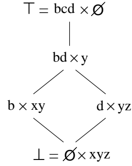
Treillis de Galois de \mathcal{R}_0
