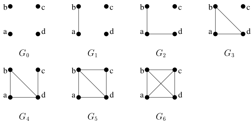
FIG. 2.3 – Famille de graphes associée à la dissimilarité du contre-exemple 2.2.3.
