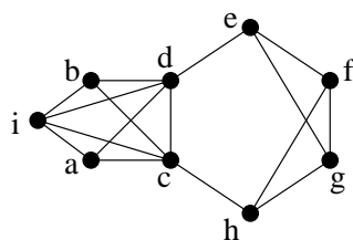
FIG. 5.1 – Le graphe G de l'exemple 5.1.7.
