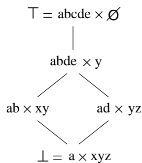
Le treillis de Galois \mathcal{L}(\mathcal{R})
