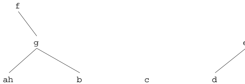
FIG. 6.6 – Construction de la sous-hiérarchie sur les intensions \mathcal{I}(\mathcal{R}) de l'exemple 6.1.12.
