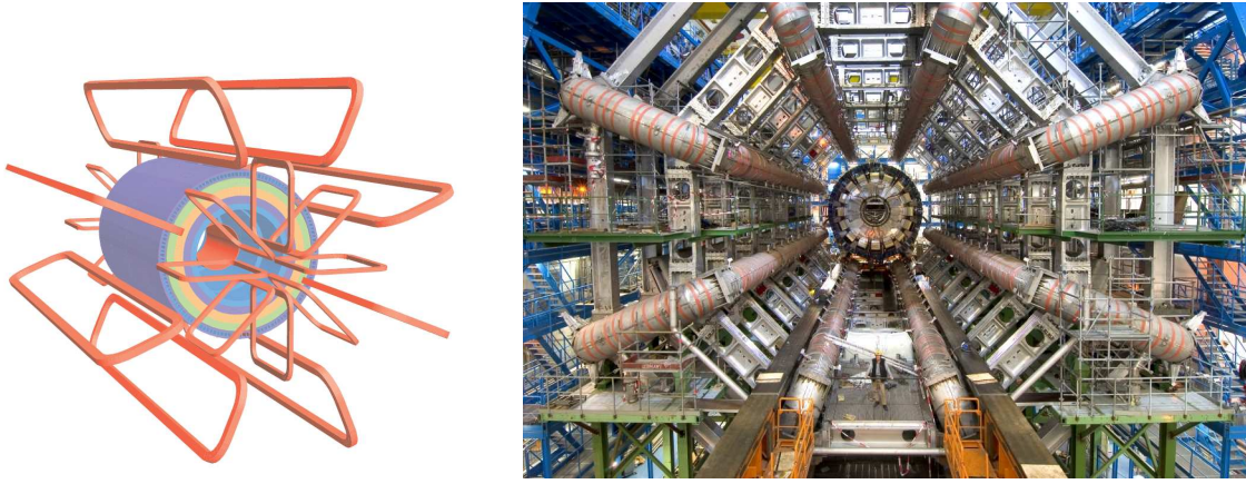
FIGURE 2.23 – Gauche : Vue d'artiste du système d'aimantation d'ATLAS; solénoïde, 8 aimants toroïdaux tonneau et les 16 aimants toroïdaux bouchons. Droite : Photo des aimants toroïdaux centraux en place dans la caverne d'ATLAS (octobre 2005).
