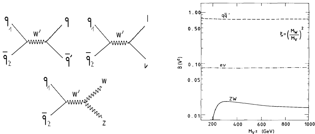
FIGURE 1.13 – Gauche : Diagrammes de Feynmann des processus incluant un boson de jauge lourd W' = V^{\pm} dans le cadre du modèle de référence. Droite : Rapports de branchements pour V^{\pm} \rightarrow W^{\pm}Z (ligne pleine), V^{\pm} \rightarrow q\bar{q}' (tirets) et V^{\pm} \rightarrow e^{\pm}\nu(\bar{\nu}) \times 10 (tirets et points) en fonction de la masse du boson de jauge lourd chargé M_{V^{\pm}} , dans le cadre du modèle de référence [25]
