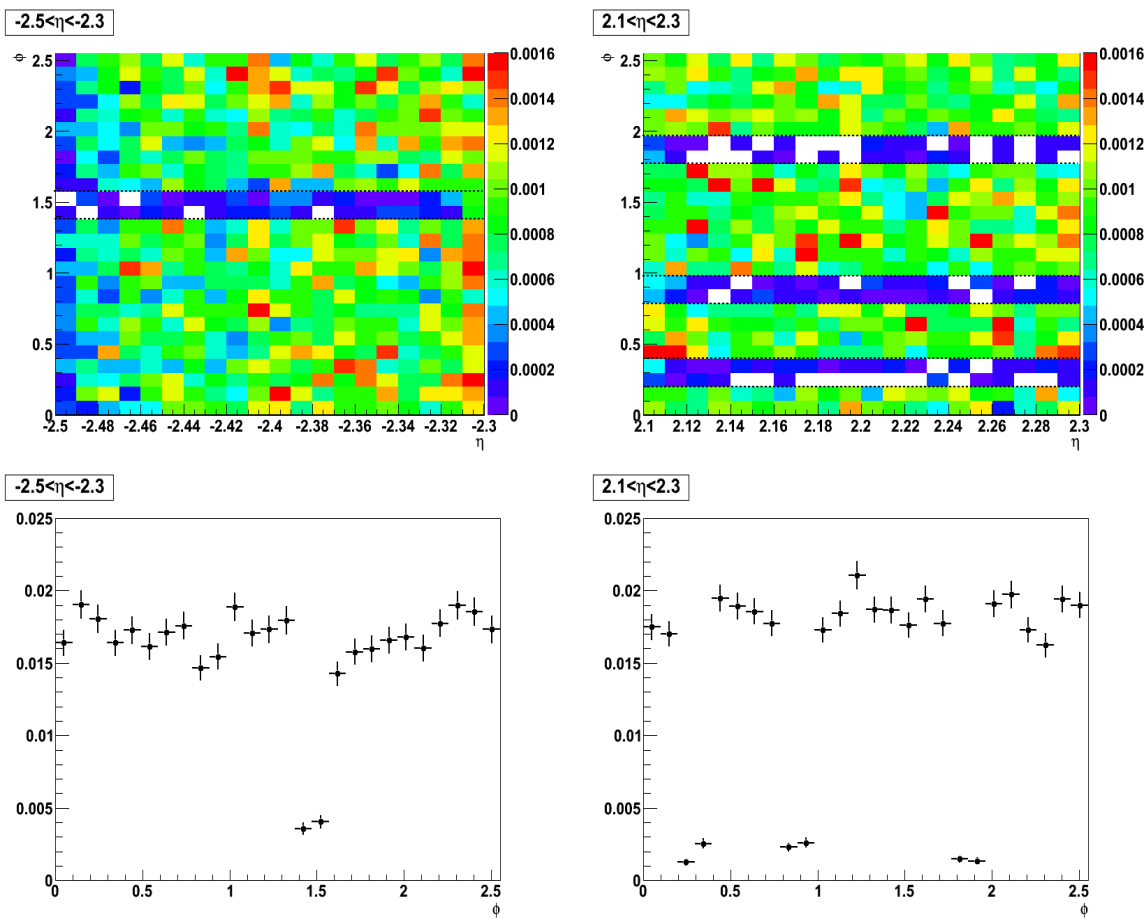
FIGURE 6.3 – Distributions en \eta et \phi (haut) et profil selon \phi (bas) de la position de 1.4 millions d'agglomérats calorimétriques issus de 20 millions d'événements de biais minimum. Les quatre zones présentant un taux anormalement bas d'objets électromagnétiques reconstruits ( \sim 80\% en moins que sur le reste de la couverture du calorimètre) sont \{\phi = 1.4 - 1.6, -2.5 < \eta < -2.3\} à gauche et \{\phi = 0.2 - 0.4, 2.1 < \eta < 2.3\} , \{\phi = 0.8 - 1.0, 2.1 < \eta < 2.3\} et \{\phi = 1.8 - 2.0, 2.1 < \eta < 2.3\} à droite.
