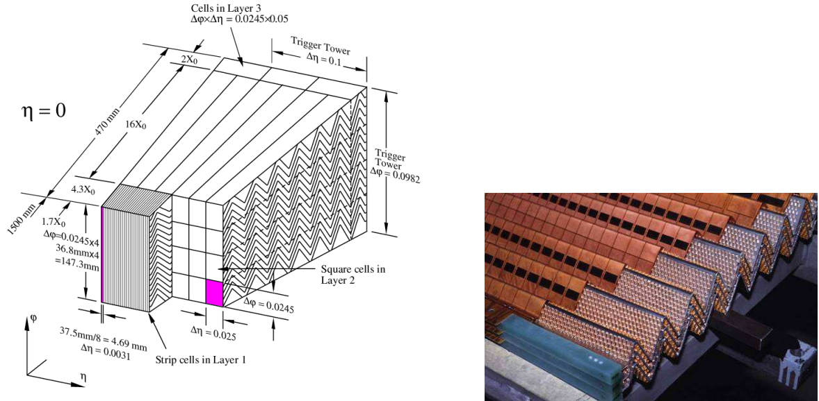
FIGURE 2.15 – Gauche : Schéma d'une région \Delta\eta \times \Delta\phi = 0.1 \times 0.1 du tonneau. Les différentes couches longitudinales sont visibles, ainsi que la granularité des cellules en \eta et \phi dans chacune des trois couches. Une tour de déclenchement est aussi représentée sur ce dessin. Droite : Photo d'une électrode, plomb et espaceur du calorimètre électromagnétique
