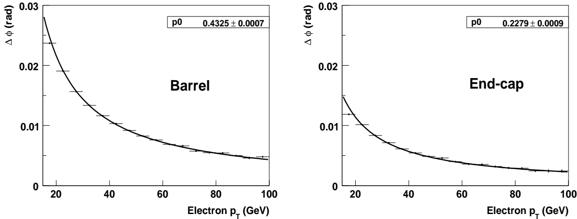
FIGURE 5.15 – Déviation moyenne pour un électron dans le champ magnétique solénoïdal à l’entrée du calorimètre électromagnétique dans le tonneau (gauche) et dans les bouchons (droite), en fonction du vrai p_T de l’électron. En supposant que les photons de bremsstrahlung soient dans le même amas de cellules calorimétriques que l’électron, la courbe représente la distance typique en \phi entre un électron et un photon émis depuis le point d’interaction. Les lignes sont le résultat d’un ajustement avec la fonction p_0/p_T .
