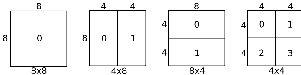
FIG. 4.4 – Partitions de sous-macroblots : 8 \times 8 , 4 \times 8 , 8 \times 4 et 4 \times 4 .
