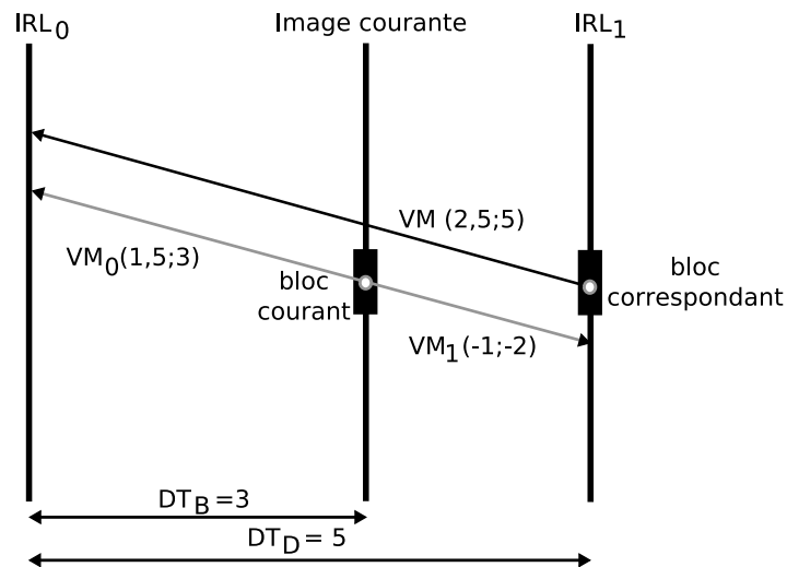
FIG. B.3 – Dans le mode temporel direct, un bloc a deux vecteurs de mouvement dérivés VM_0 et VM_1 pointant vers deux images de référence de la liste 0, IRL_0 , et de la liste 1, IRL_1 .
