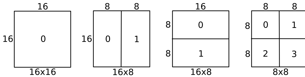
FIG. 4.3 – Partitions de macroblocs : 16 \times 16 , 8 \times 16 , 16 \times 8 et 8 \times 8 .
