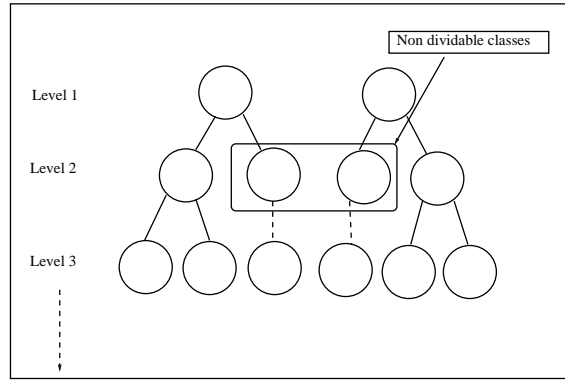
FIG. 4.3 – Classification hiérarchique descendante.
