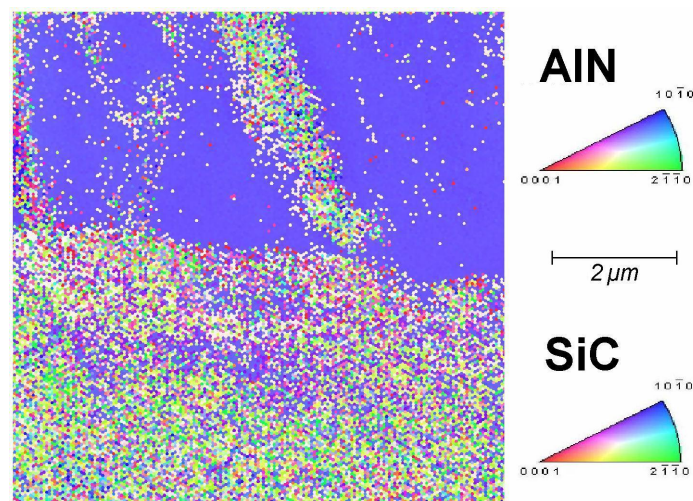
FIG. 5.26 – Image EBSD de la tranche d’une couche d’AlN épitaxié sur SiC 4H 8° off. L’étude des orientations cristallines est difficile au niveau du substrat de SiC (en bas) car le polissage n’était pas suffisant pour éliminer la zone écrouie. Le code de couleur correspondant aux orientations est représenté par les triangles à droite.
