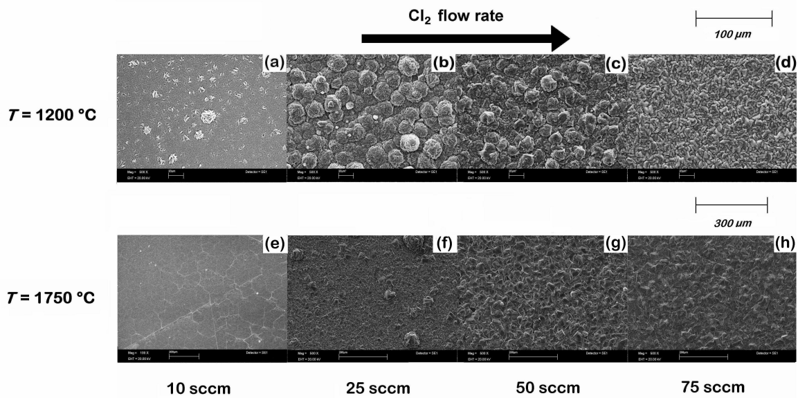
FIG. 4.14 – Effet du débit de \text{Cl}_2(g) sur la morphologie des couches d'AlN déposées sur un substrat de \text{SiC } 4H off axis non collé
