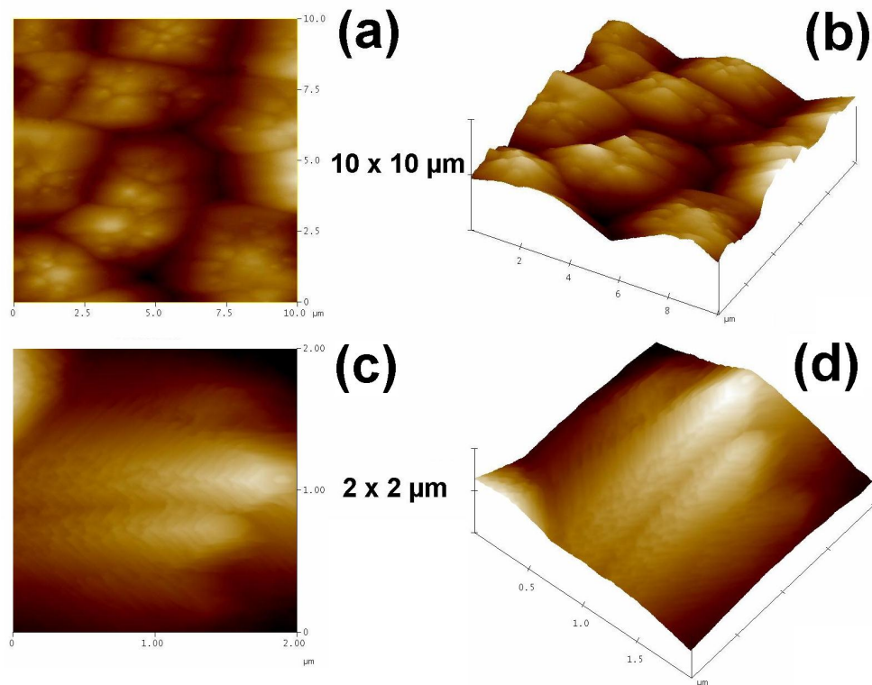
FIG. 5.45 – Images AFM d'un dépôt d'AlN élaboré sur AlN template à 1600°C pour Cl_2(g) = NH_3(g) = 7,5 sccm
