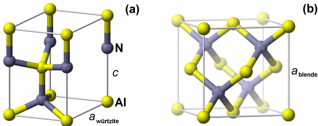
FIG. 1.1 – Structures cristallines Würtzite (a) et Zinc Blende (b) du nitrure d'aluminium
