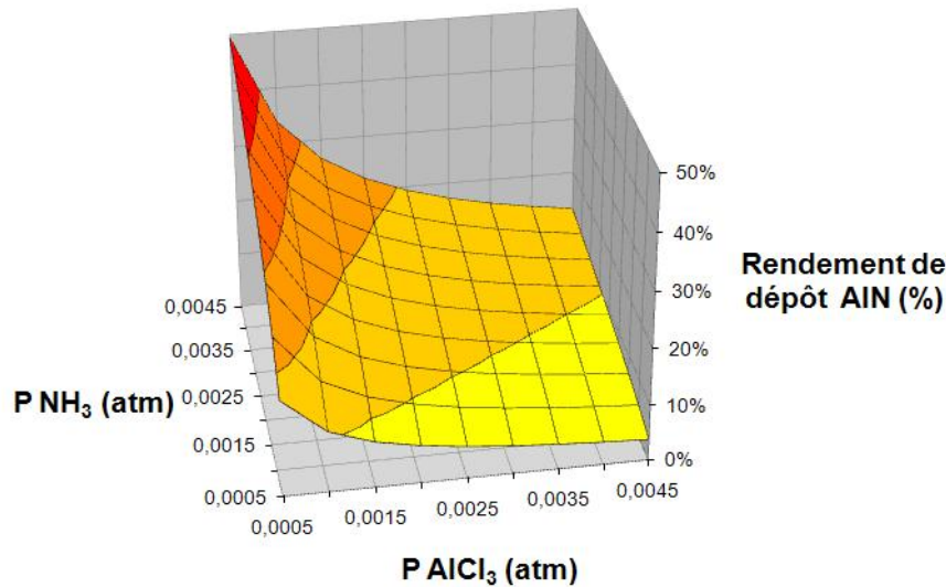
FIG. 3.24 – Courbe d'isoréponse calculée de rendement d'AlN à 1100°C et 0,01 atm en fonction des pressions partielle d' \text{AlCl}_3(g) et de \text{NH}_3(g)
