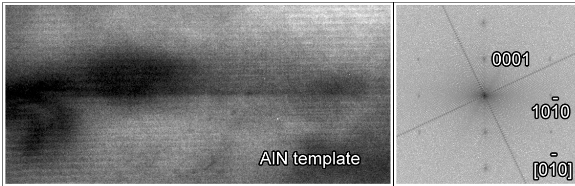
Figure 5.50: Image haute résolution de l'interface entre la couche AlN déposée et le template AlN utilisé comme substrat et sa transformée de Fourier associée.
