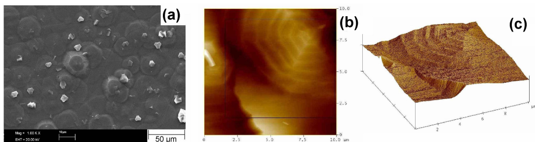
FIG. 5.21 – Images MEB (a) et AFM (b et c) d'un dépôt d'AlN de 6\ \mu\text{m} d'épaisseur sur substrat de SiC 6H (0001) élaboré à 1750^{\circ}\text{C} .
